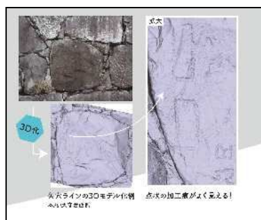
矢穴の解説(抜粋)
