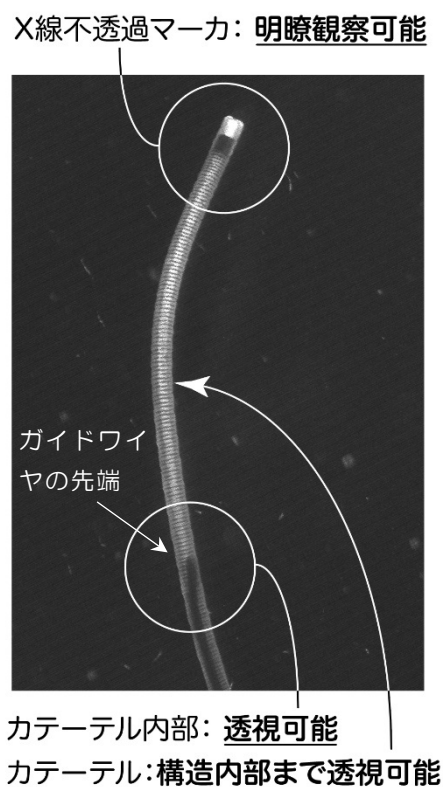
(b) 本製品による近赤外線観察
