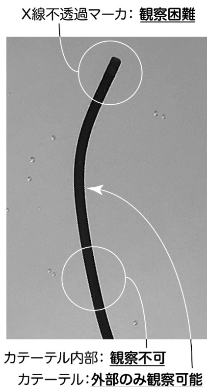
(a) 通常の光学顕微鏡による可視光観察
