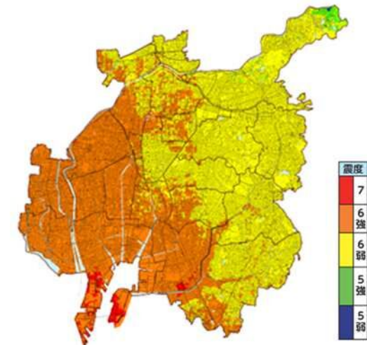
南海トラフ巨大地震の被害想定 震度分布 (あらゆる可能性を考慮した最大クラス)
