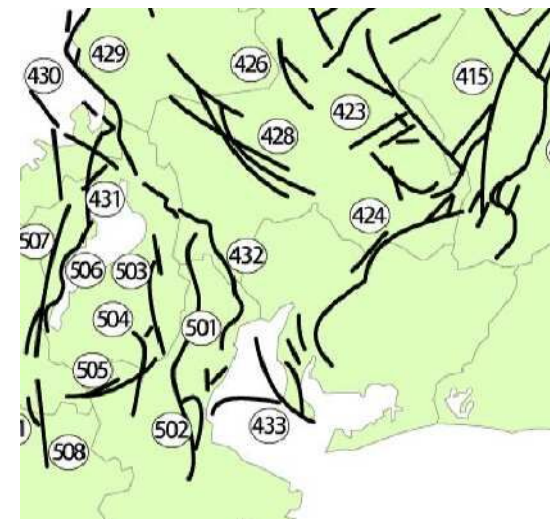
主要活断層帯の概略位置図
