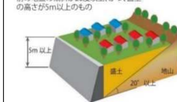
◇腹付け型大規模盛土造成地 傾斜地に盛土した造成宅地で、盛土する 前の地盤の傾斜が20度以上、かつ、盛土 の高さが5m以上のもの
