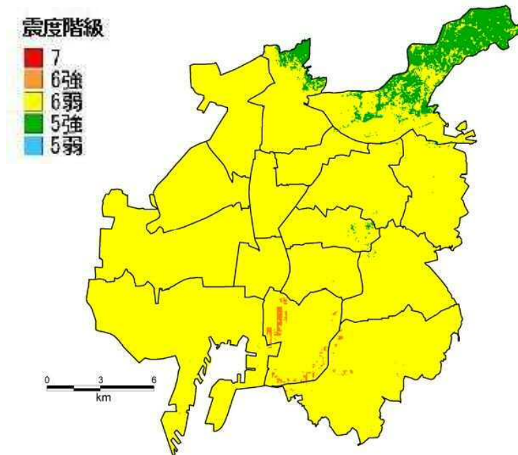
過去の地震を考慮した最大クラスの震度分布図
