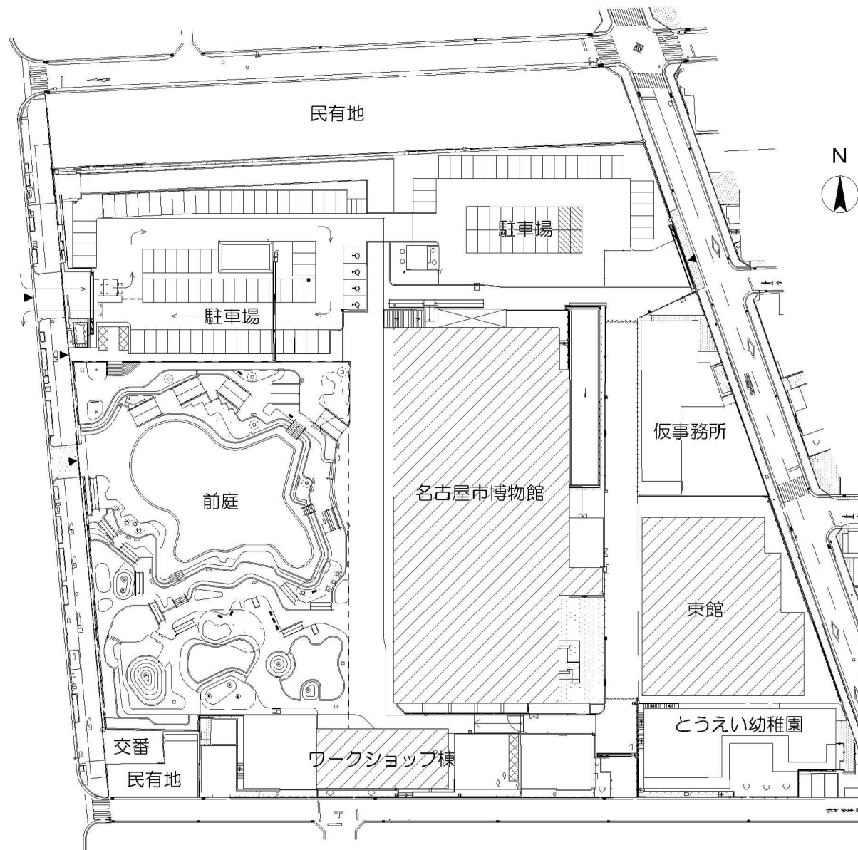
配置図
