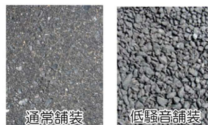
通常舗装と低騒音舗装の見た目の違い
