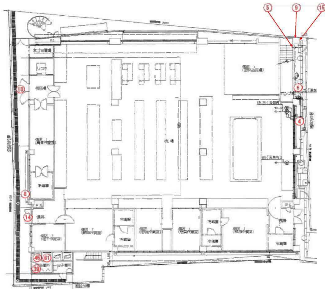
1階 平面図
