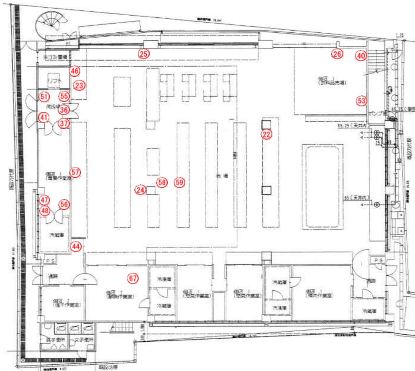
1階 平面図
