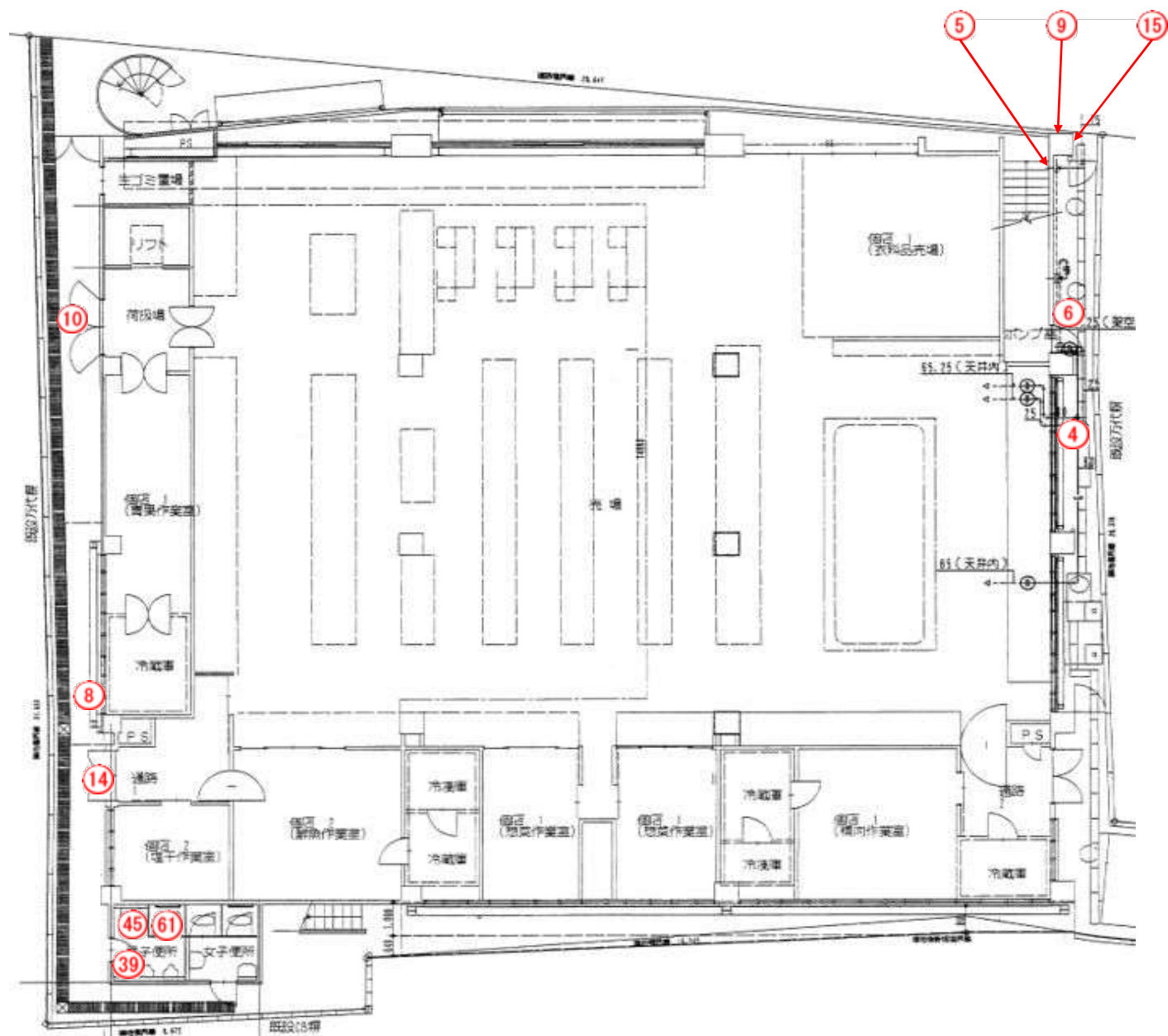
1階 平面図
