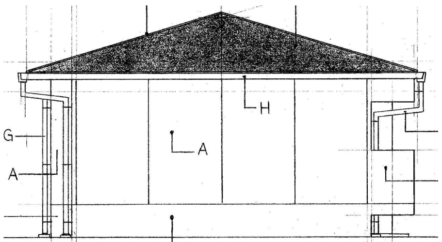
西 立面图 1/100
