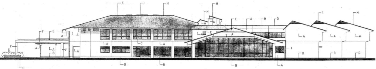
西 立 面 图 1/200
