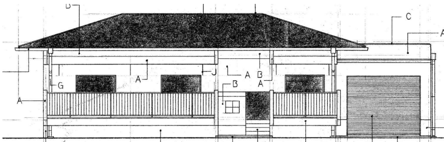
南 立面図 1/100
