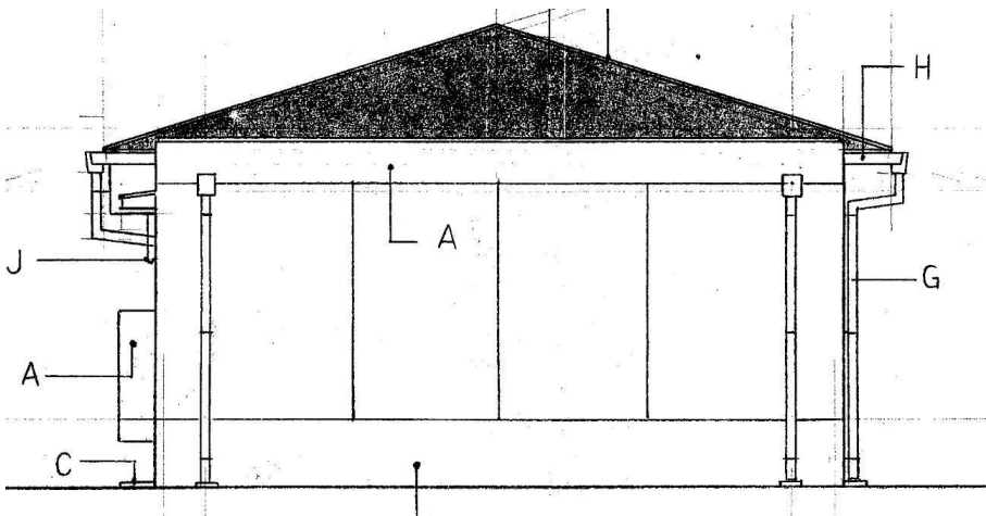
東 立面図 1/100
