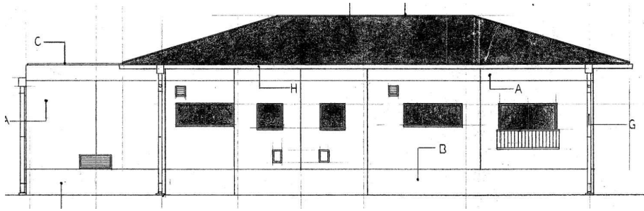
北 立面图 1/100
