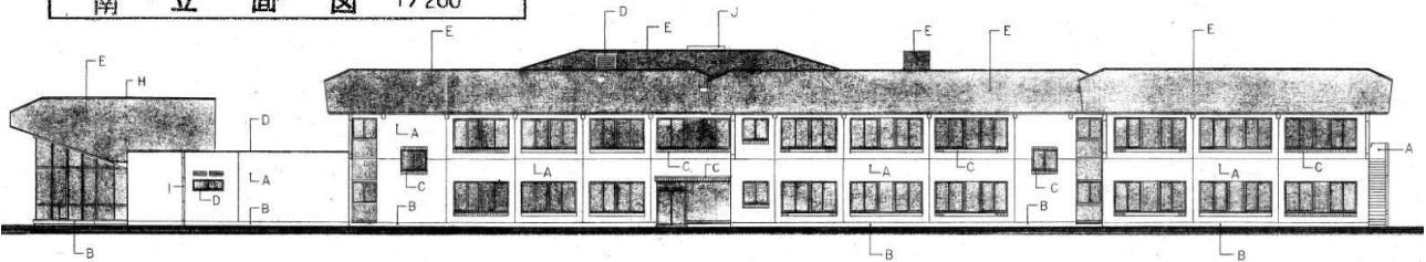
南 立 面 图 1/200
