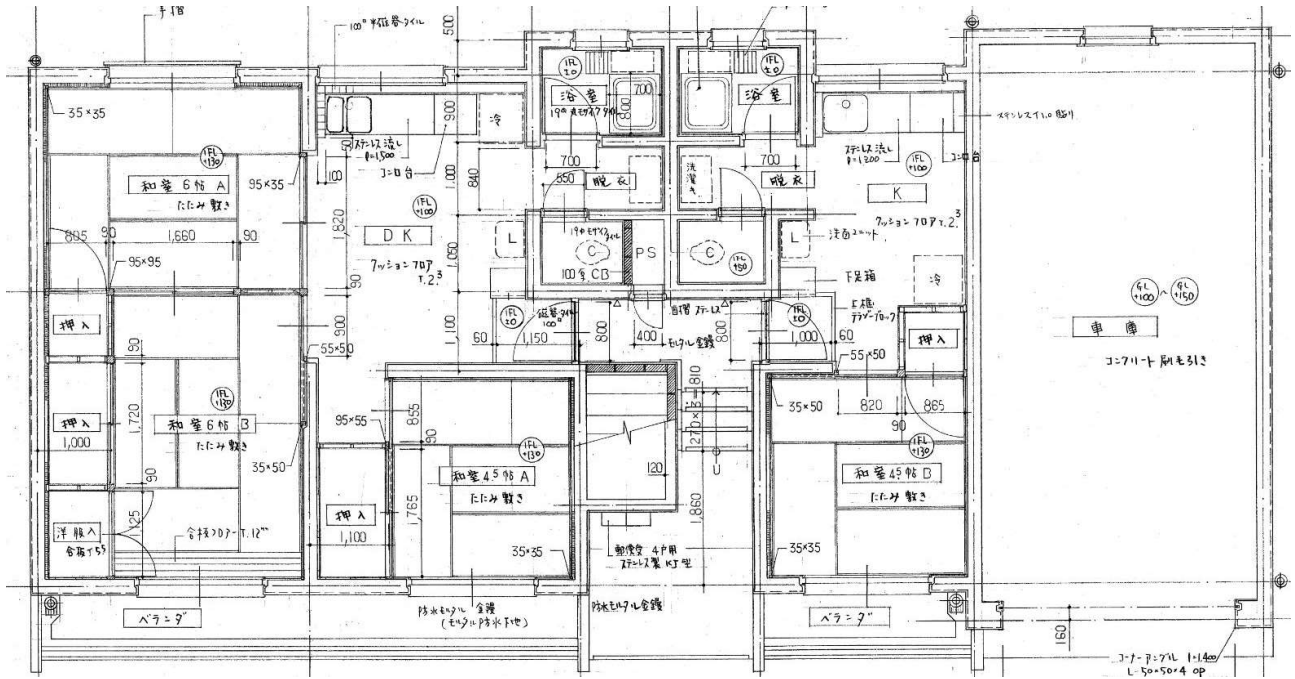
建物② 1階平面図
