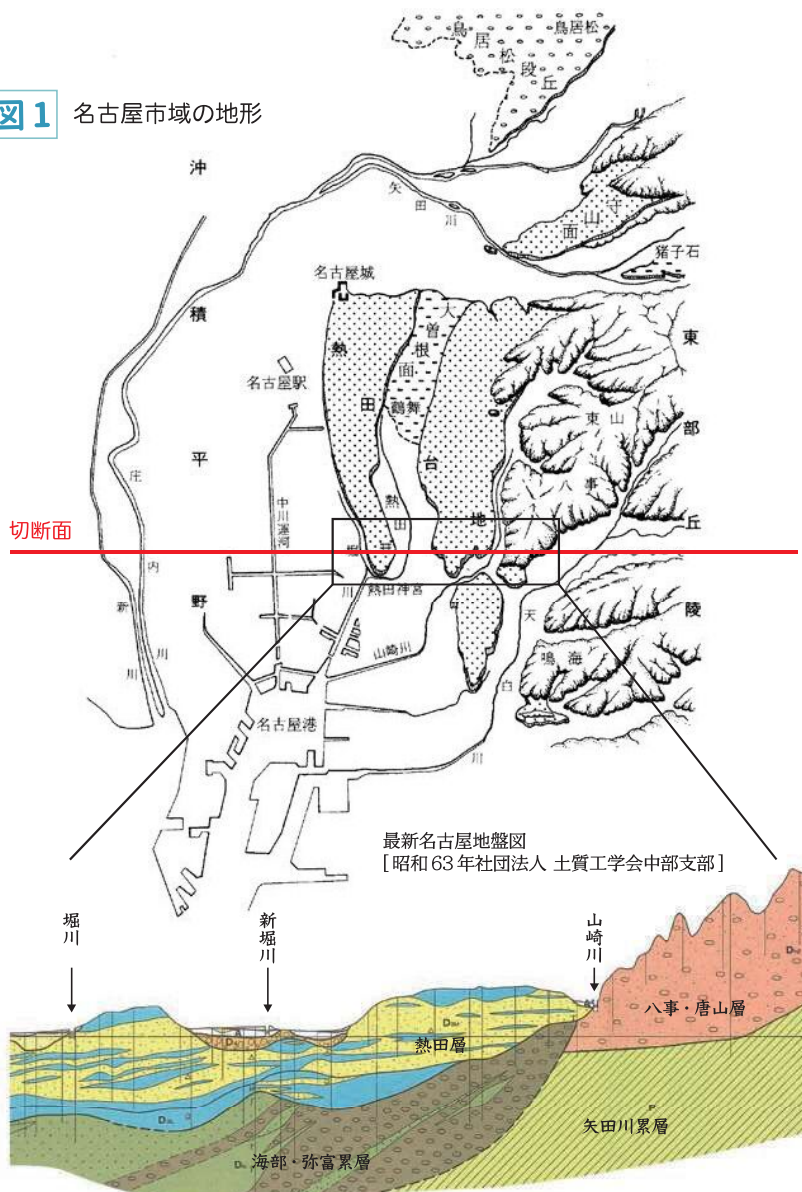
図 2 名古屋市域の断面図（切断面は図 1 参照）
