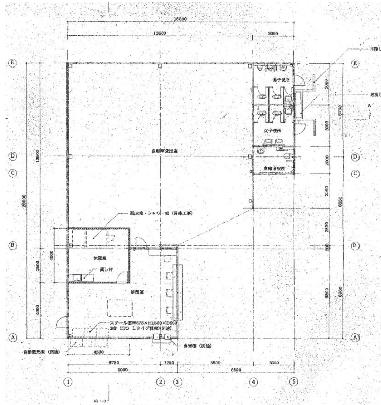
平面図 S=1:100
