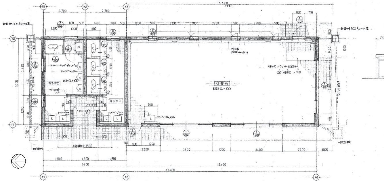
平面図 S=1:100
