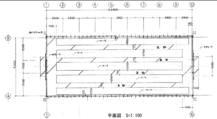
平面図 S=1:100
