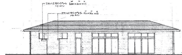
東立面図 S=1:100
