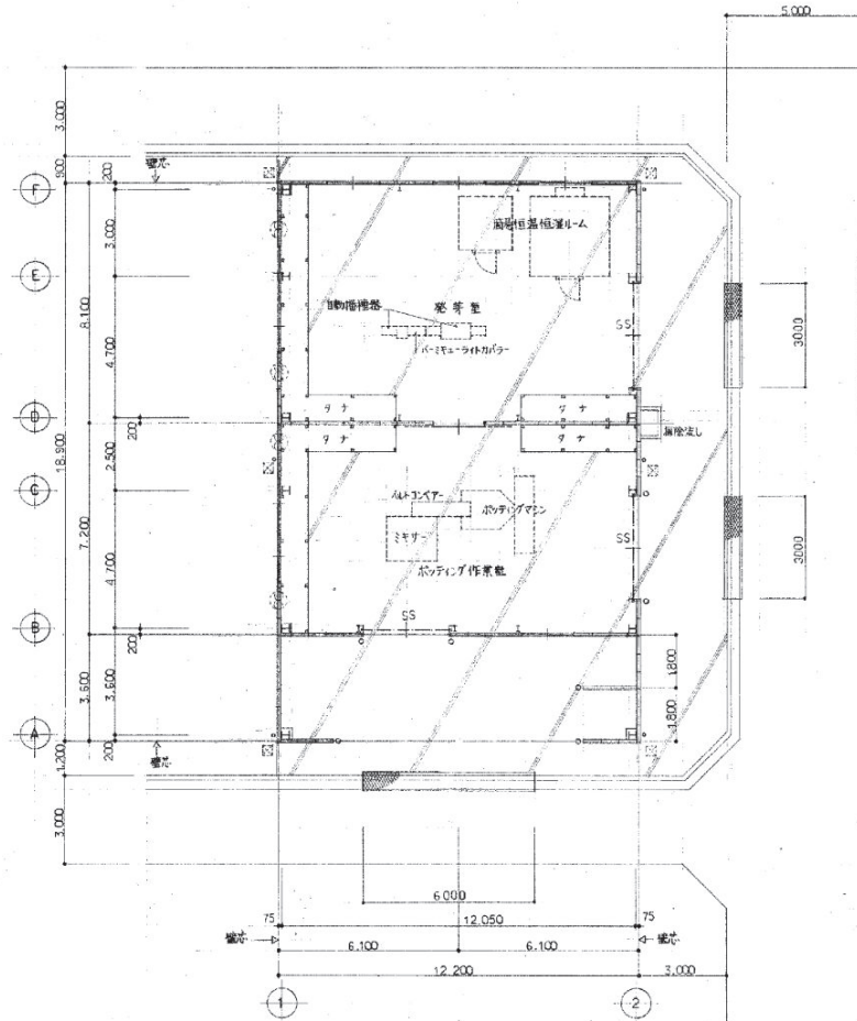
平面図 S=1:100
