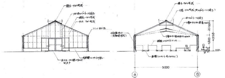
妻側立面図 S=1:100
