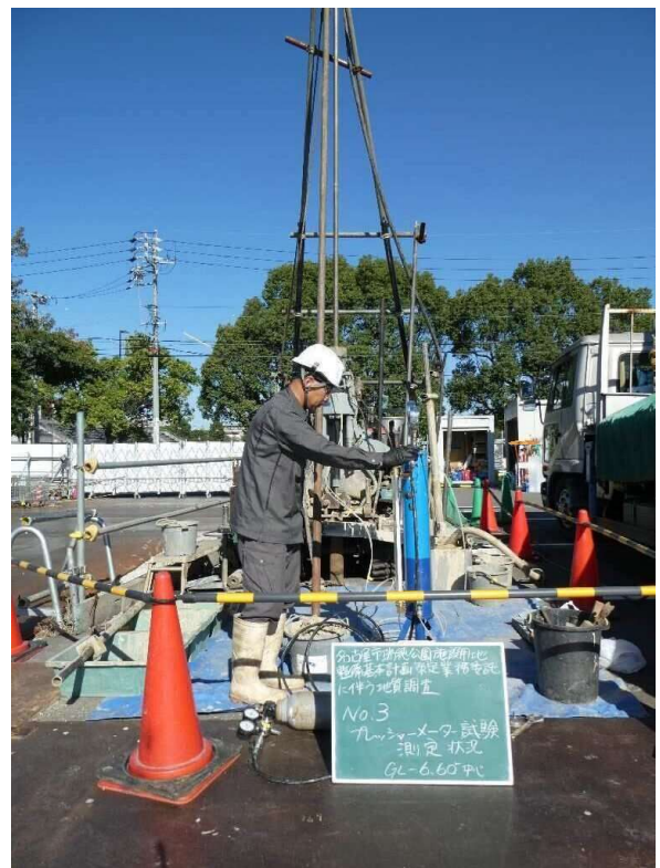
プレシャーマーター試験
