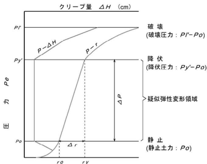
図 2.6 プレッシュャーメーター試験結果例
