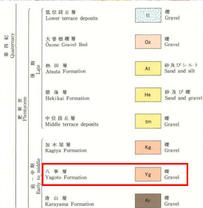
図 3.2 調査地周辺の地質図 ●:調査地 (『名古屋南部地域の地質』/地質調査所)
