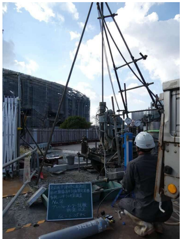
プレシャーマーター試験 GL-6.0m
