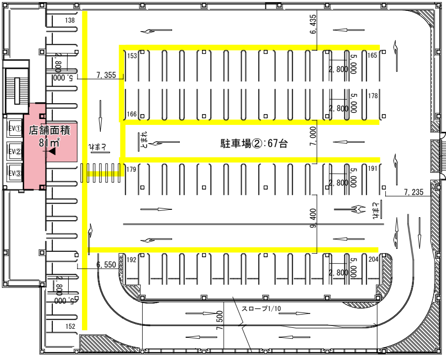
3階平面図
