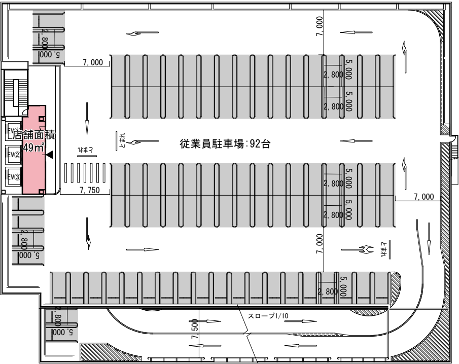
R階平面図
