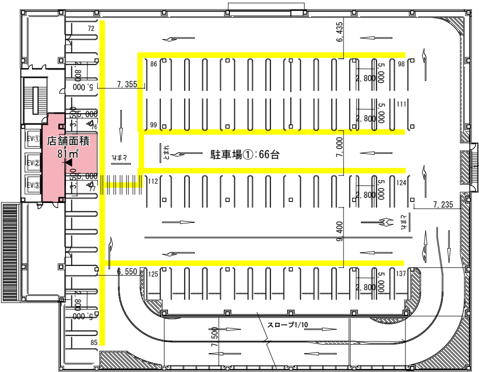
2階平面図
