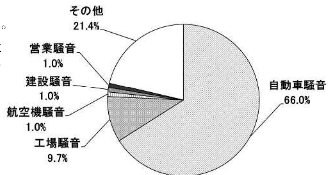
図 3 主な寄与音源
