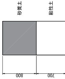
A2 試掘断面図 S=1:50
