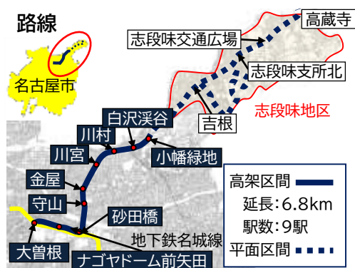
幅7.5mのコンパクトな高架構造物とし、建設費を低減
