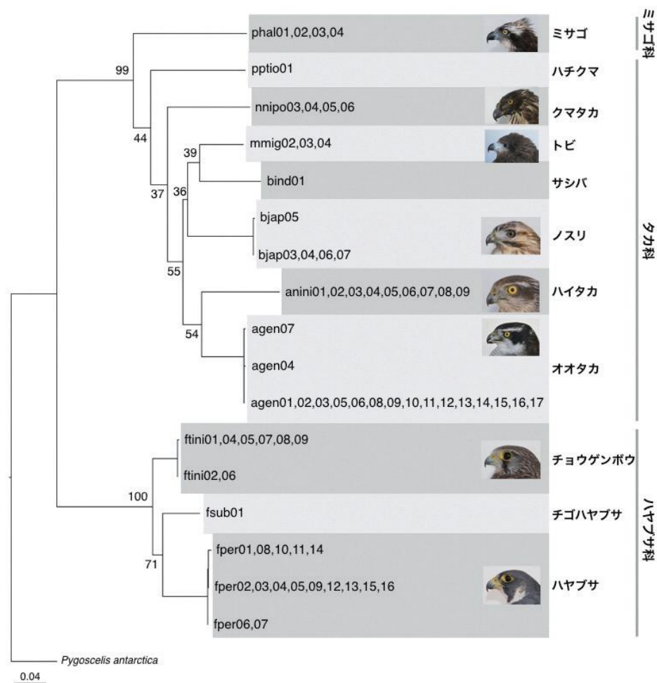
図1. DNAバーコード領域の塩基配列（アラインメント後693サイト）を用いて作成した名古屋周辺ワシタカ類の最尤系統樹。タクソンは同一のハプロタイプを持つものをまとめて解析し、タクソン名には該当するサンプルID番号を記した。外群にはヒゲペンギン（ Pygoscelis antarctica : INSD アクセッション番号 EU525475）を使用し、各結節点には1000回の試行から求められたブートストラップ確率を示した。
