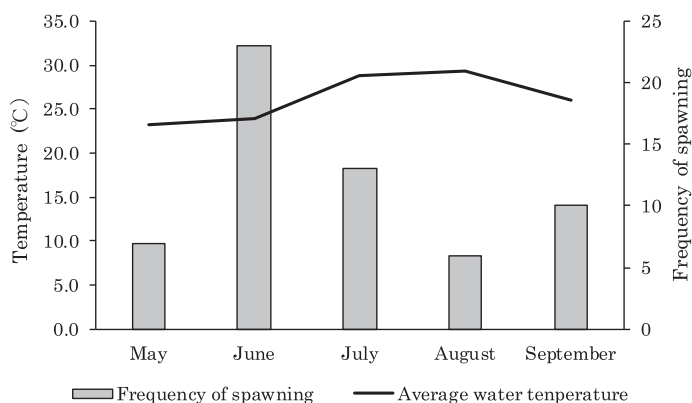
図2. 月ごとの平均水温と産卵頻度の関係
