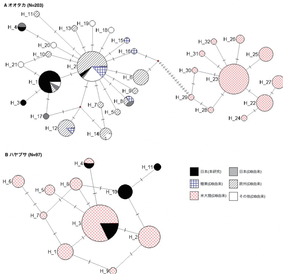
図3. 制御領域の塩基配列を用いて作成したオオタカ及びハヤブサのハプロタイプネットワーク図。節における円の大きさはハプロタイプの相対頻度を表す。本研究でシーケンスした名古屋周辺のサンプル（黒）、BOLDまたはINSDデータベース（DB）由来の日本国内のサンプル（灰色）、欧州産のサンプル（斜線）、極東産のサンプル（格子）、米大陸産のサンプル（斜め格子）、その他の地域のサンプル（白）。各ハプロタイプをつなぐ線上の一区切りは、1塩基置換を示す。
