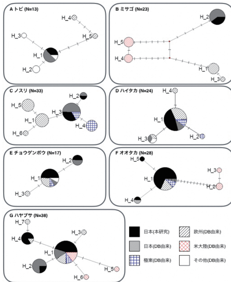
図2. DNAバーコード領域の塩基配列を用いて作成したハプロタイプネットワーク図。節における円の大きさはハプロタイプの相対頻度を表す。本研究でシーケンスした名古屋周辺のサンプル(黒)、BOLDまたはINSDデータベース(DB)由来の日本国内のサンプル(灰色)、欧州産のサンプル(斜線)、極東産のサンプル(格子)、米大陸産のサンプル(斜め格子)、その他の地域のサンプル(白)。各ハプロタイプをつなぐ線上の一区切りは、1塩基置換を表す。
