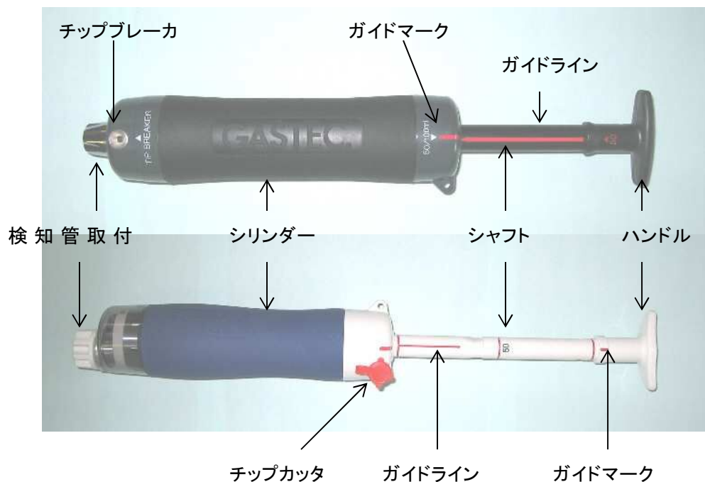
図6 ガス採取器の1例
