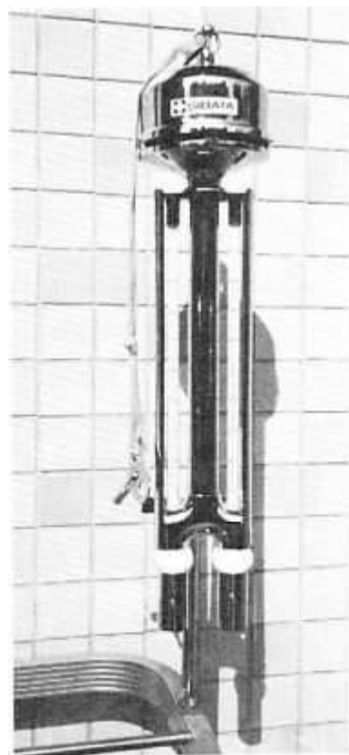
図9 アスマン通風乾湿計
