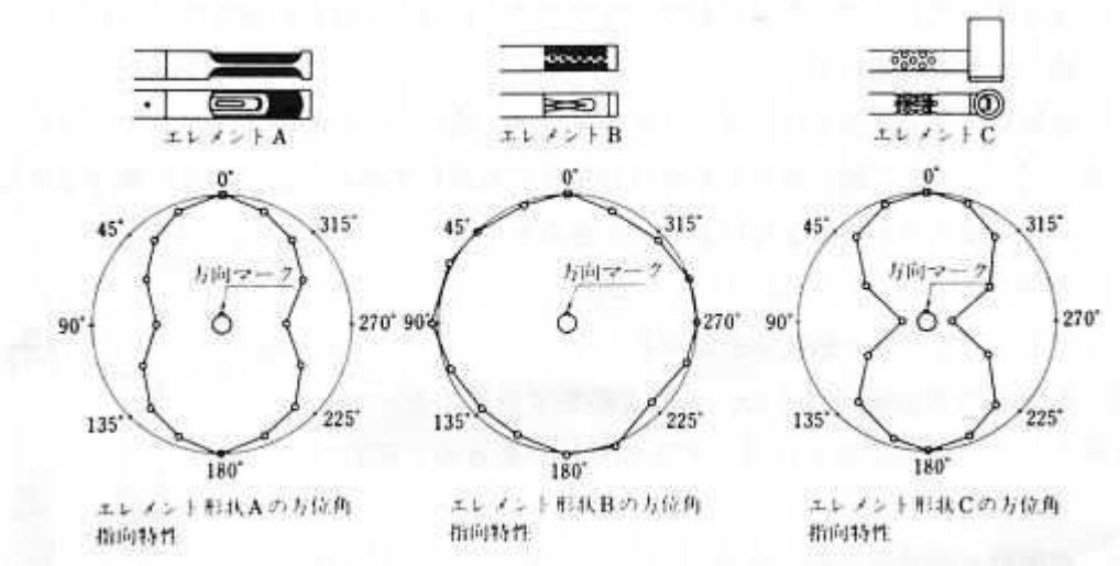
図 11 エレメントの形状と方位角指向特性
