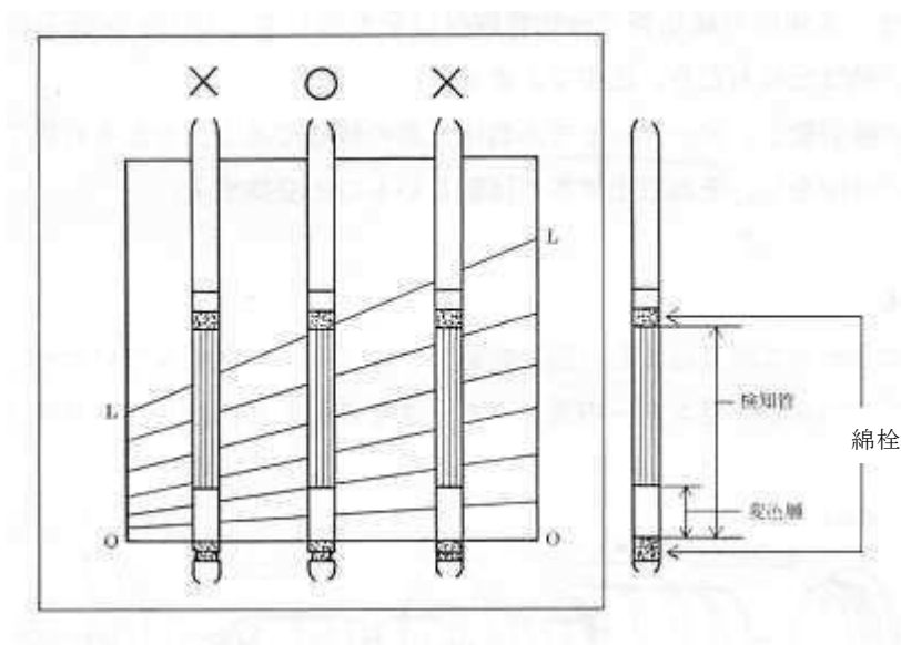
図 7 濃度表式の検知管の濃度の読み方
