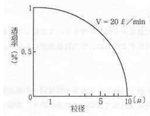
図3 多段型分粒装置の分粒特性
