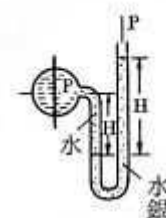
U字管液柱圧力計 (マノメータ)
