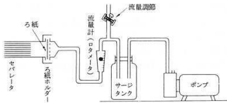
図1 ローボリウムエアサンプラの構成図
