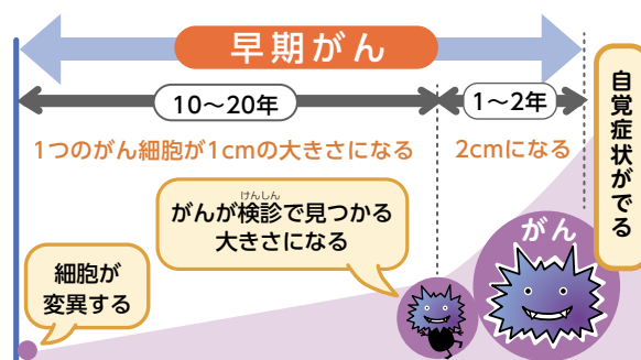
がんの発生と進行（乳がんの場合）
