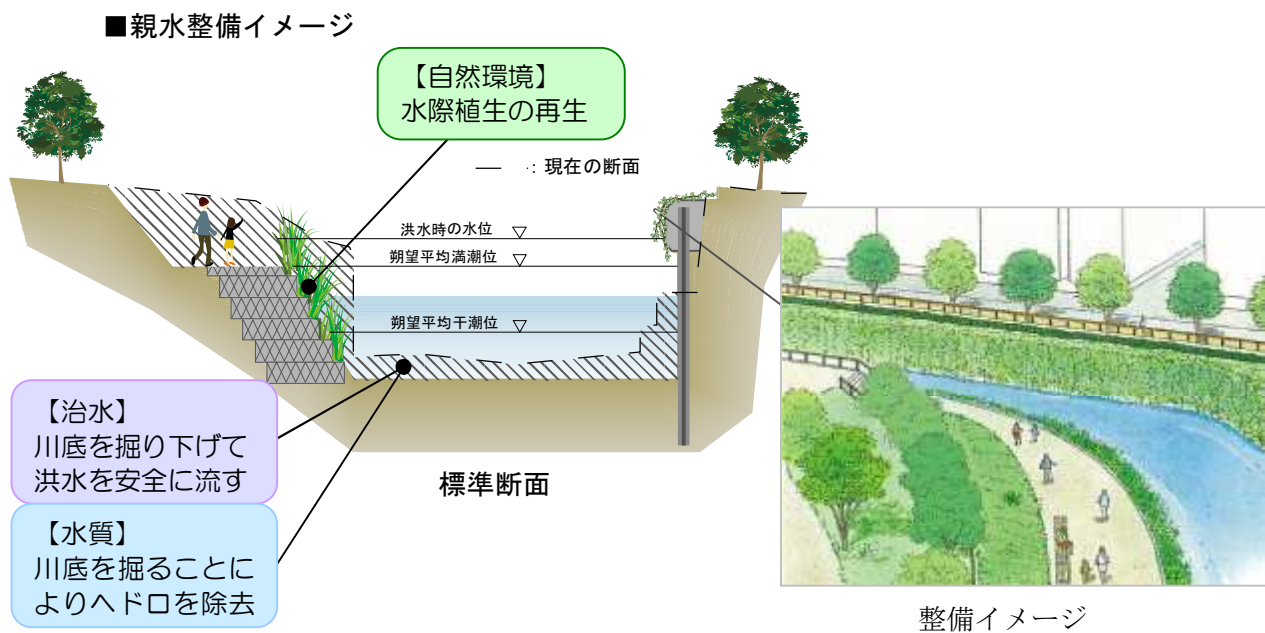
図-3.5 緩勾配整備イメージ（名城地区：10.65km～12.10km）
