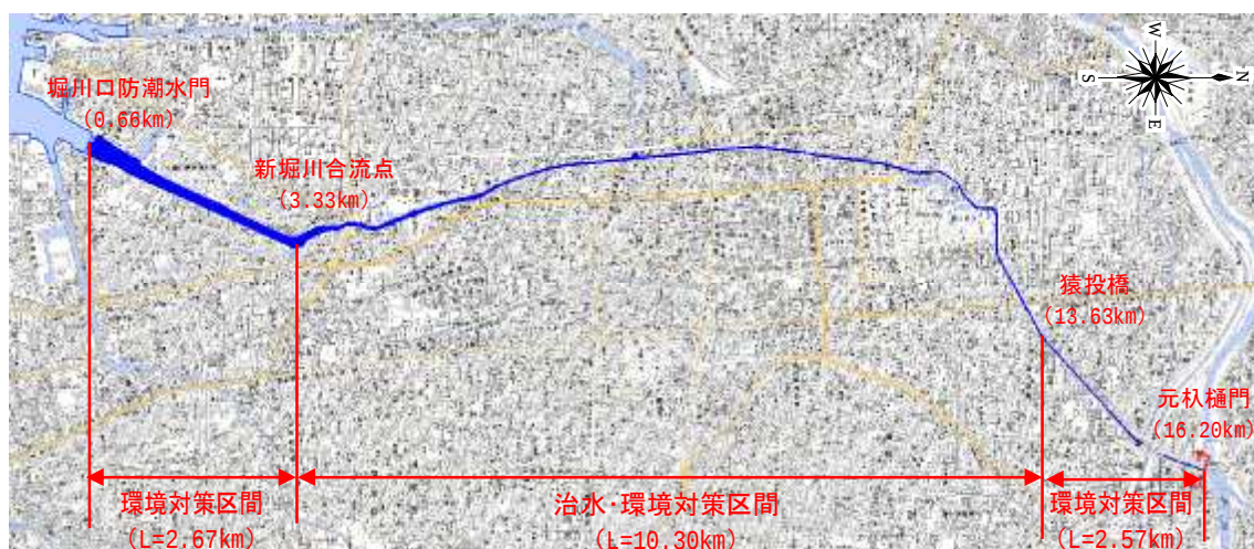
図-3.3 堀川 河川改修区間位置図
