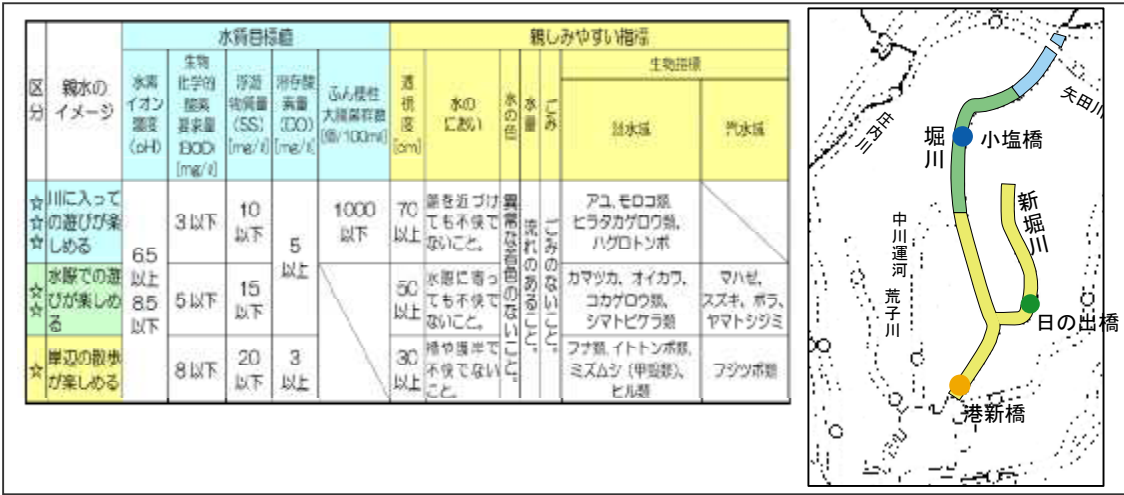
図-1.15 名古屋市 水質汚濁に係る環境目標値及び調査地点位置
