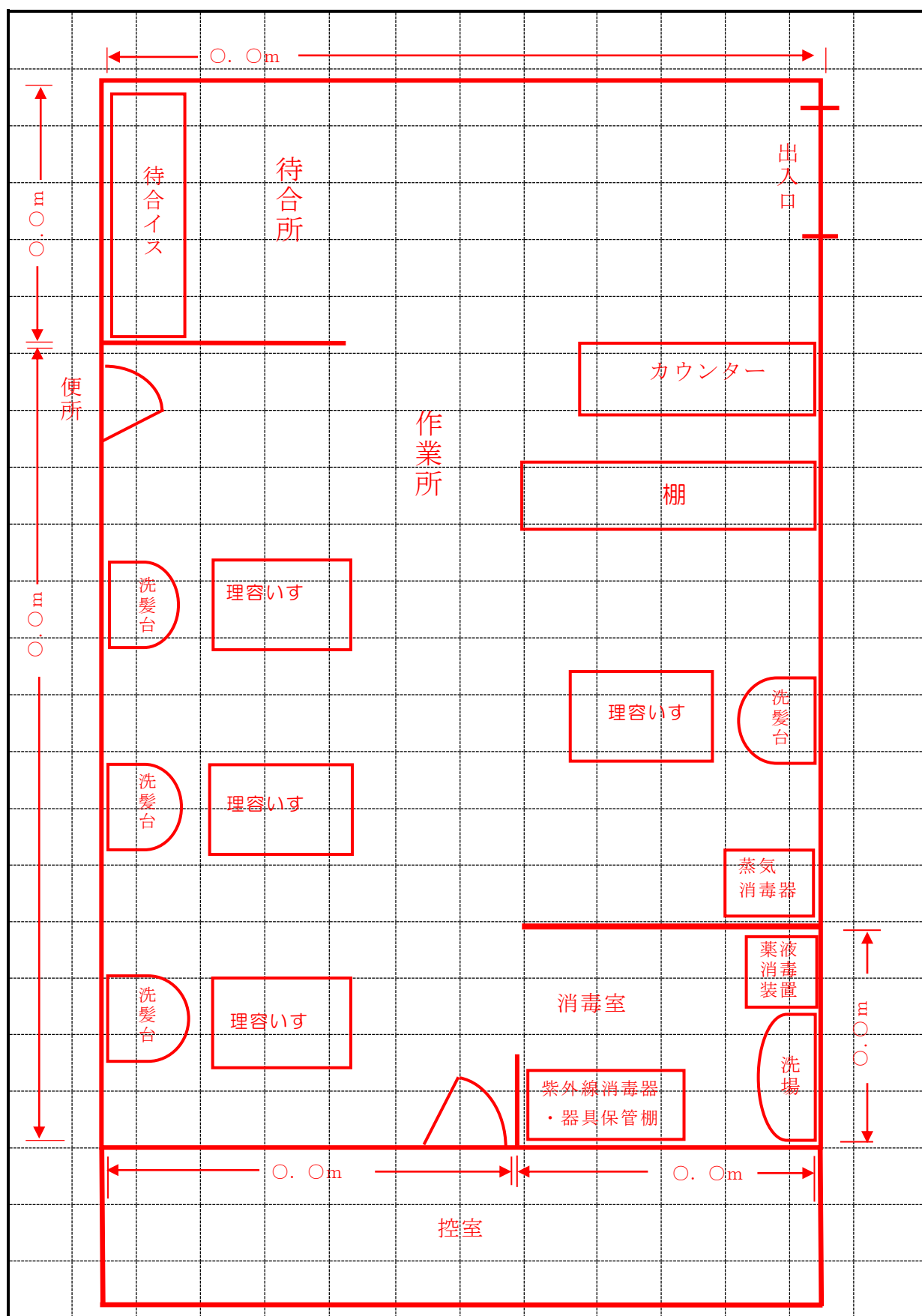
理容所の平面図及び機械器具等の配置図
