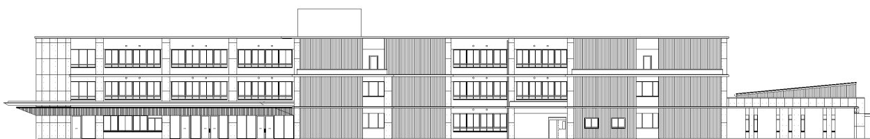
北立面图
