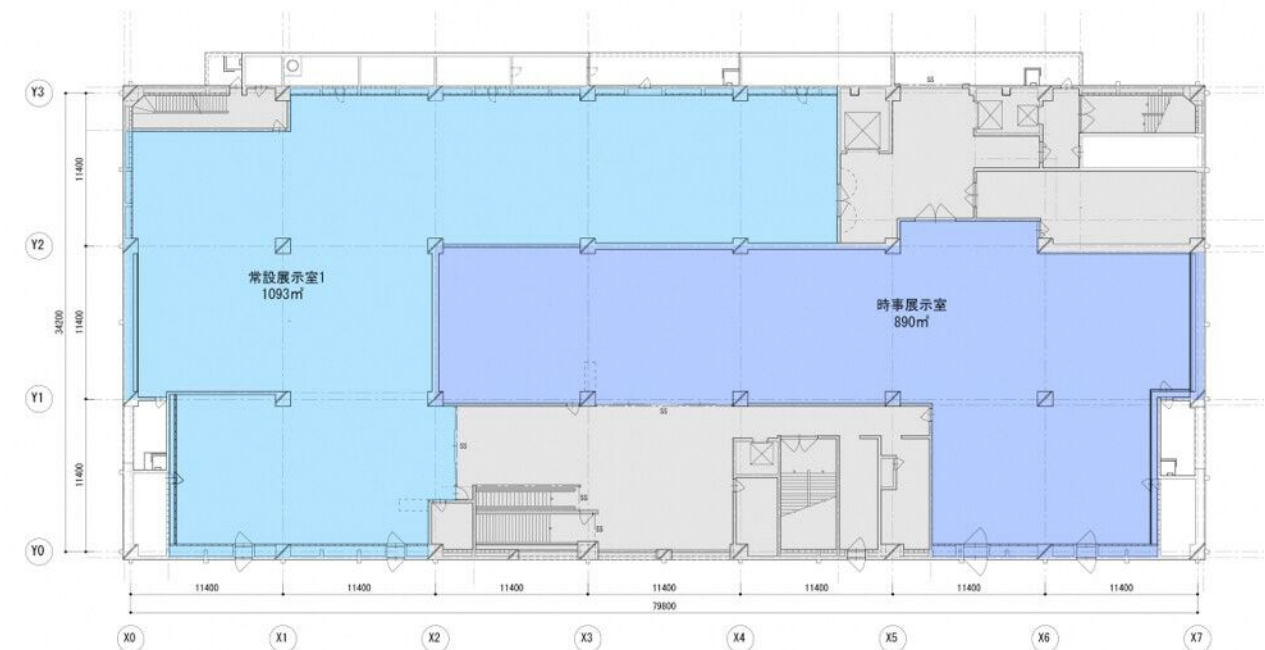
3階 平面図（改修案）
