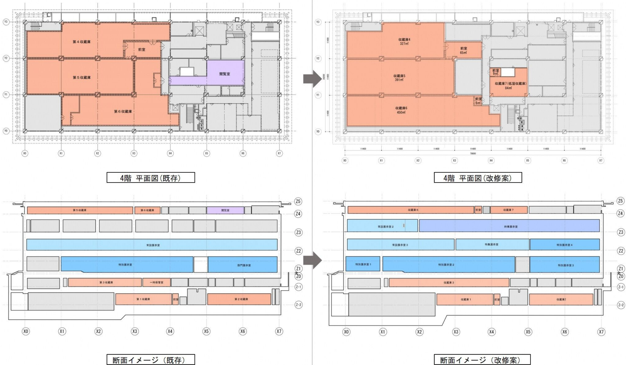
図 22 4 階、断面イメージ
