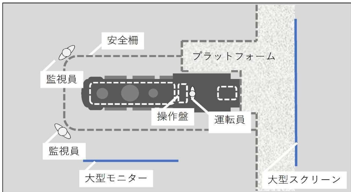
B6型蒸気機関車模型図(平面図)
