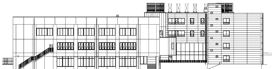
西立面图
