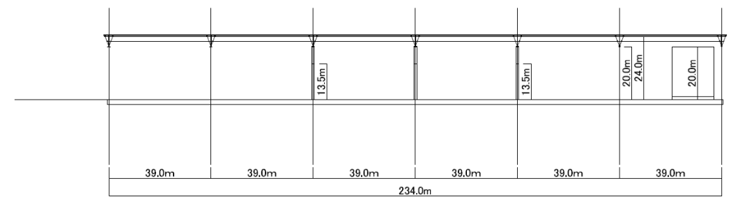
a-a断面図 S=1/2000
