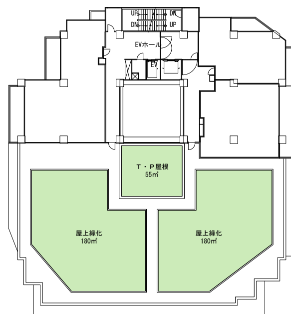
1 5 ～ 1 7 階平面図
