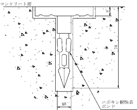
断面図
