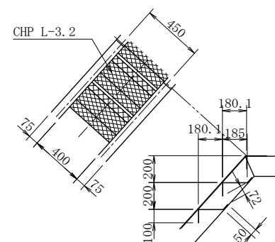
階段部詳細図
