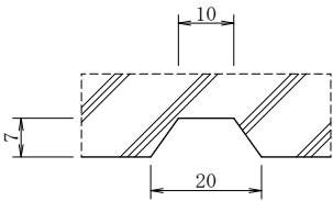
化粧目地詳細図
