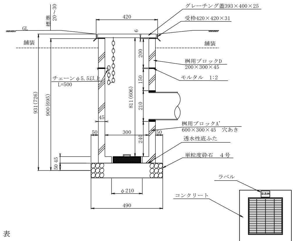
(300B', 浸透)
