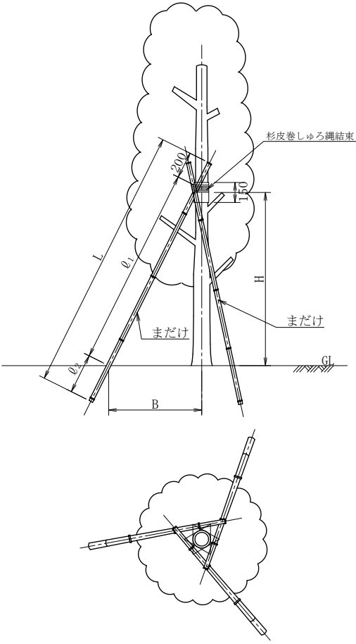
三本竹支柱
