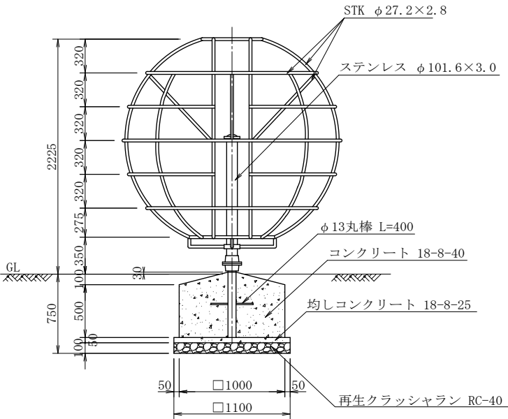
立 面 図
