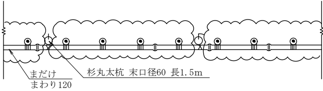
正面図
