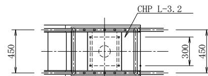
デッキ部平面図
