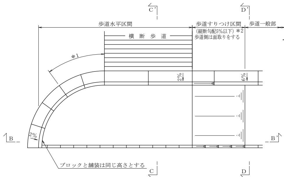
平面図
