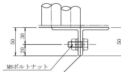
B部取付詳細図
