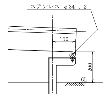
C部取付詳細図
