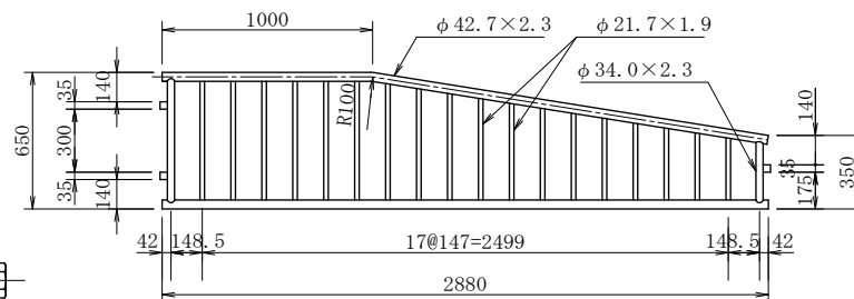
(端部パネル)
