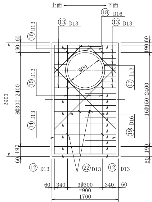
頂 版
