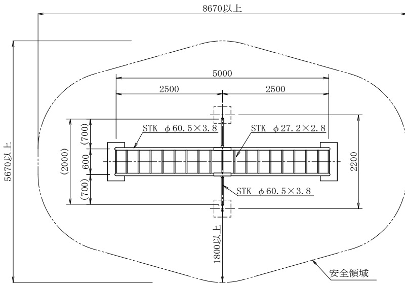
平面图
