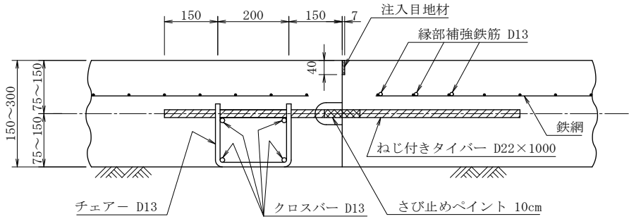
突 合 せ 目 地
