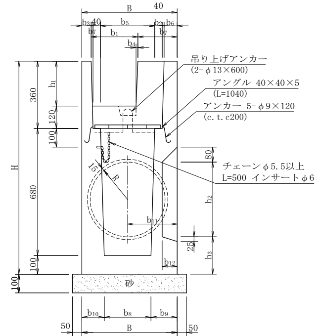
A-A 断 面 図
