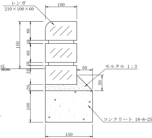
レンガ植樹 3 段
