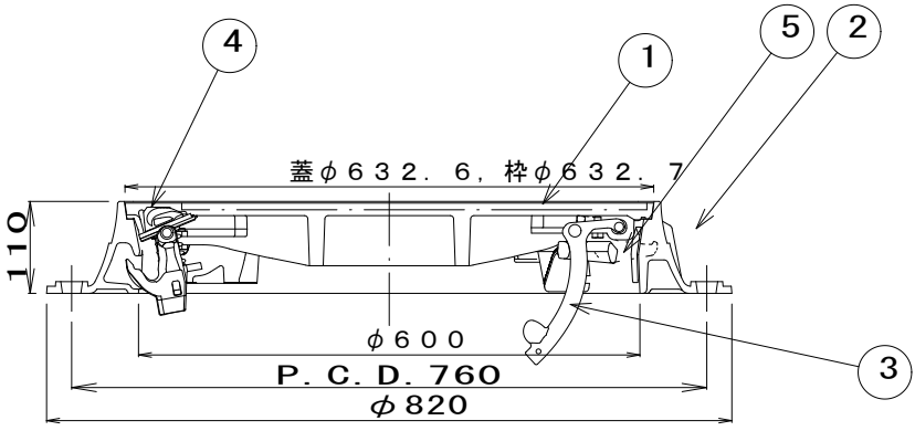
蓋, 枠断面図
