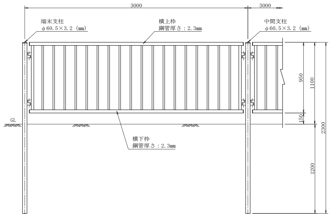
組立図
