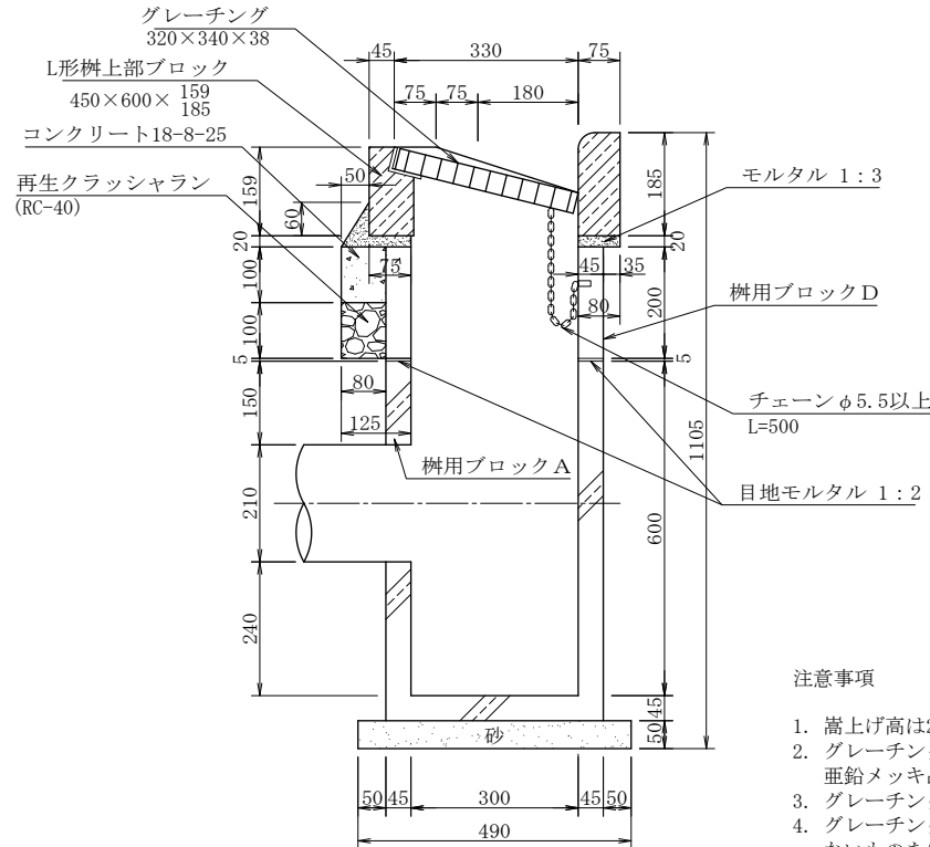
A-A 断 面 図
