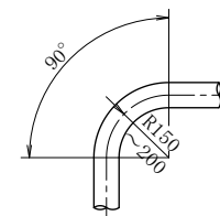
曲部詳細図
