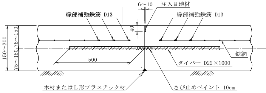
ダ ミ ー 目 地
