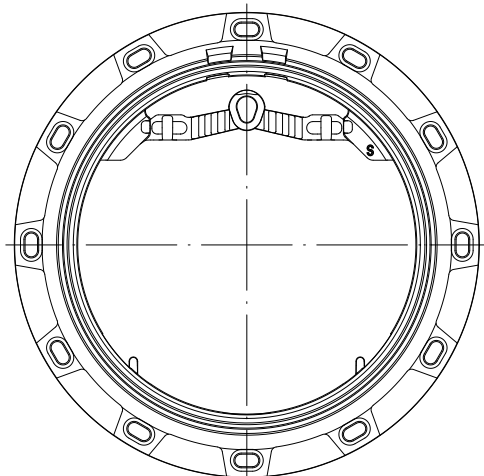
枠平面図
