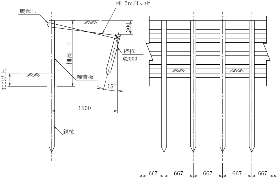
柵高 1.0m～1.2m
