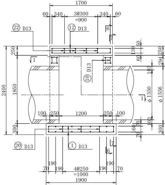
2 - 2 断 面
