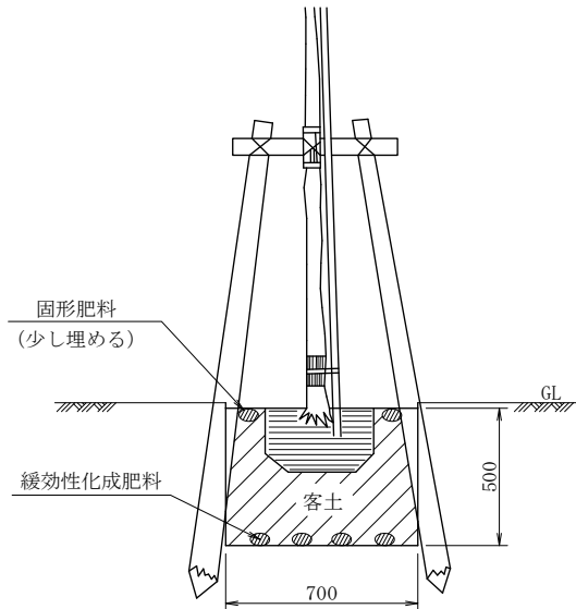
断面図
