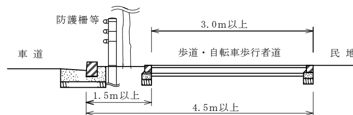
フラット式 セミフラット式
