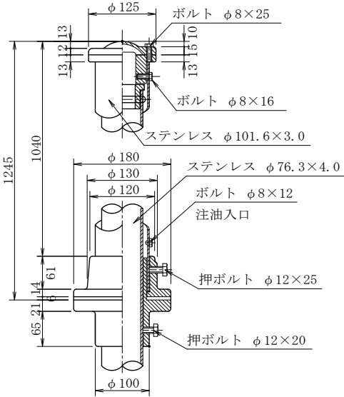
ツカミ部詳細図
