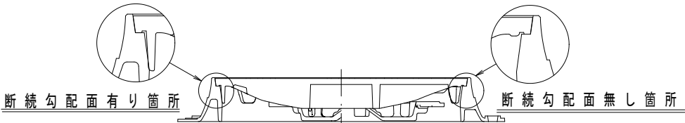
A - A 断面図
