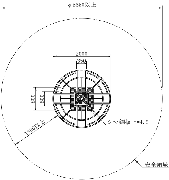
平 面 図
