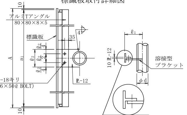
アンカーボルト詳細図
