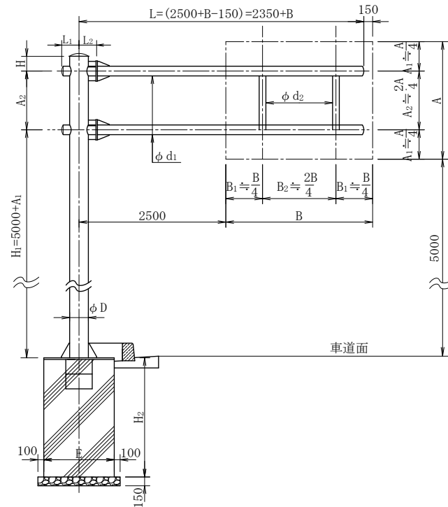
(単位: mm)
