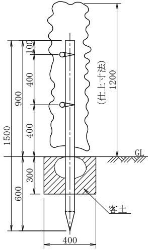
側面図
