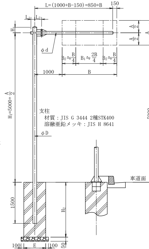
(単位: mm)
