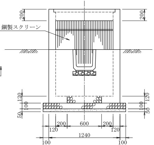
B-B 断面図
