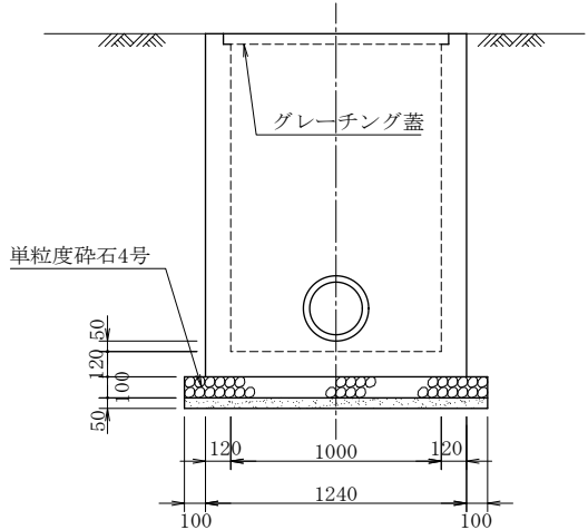
C-C 断面図
