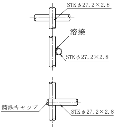
ツカミ部詳細図
