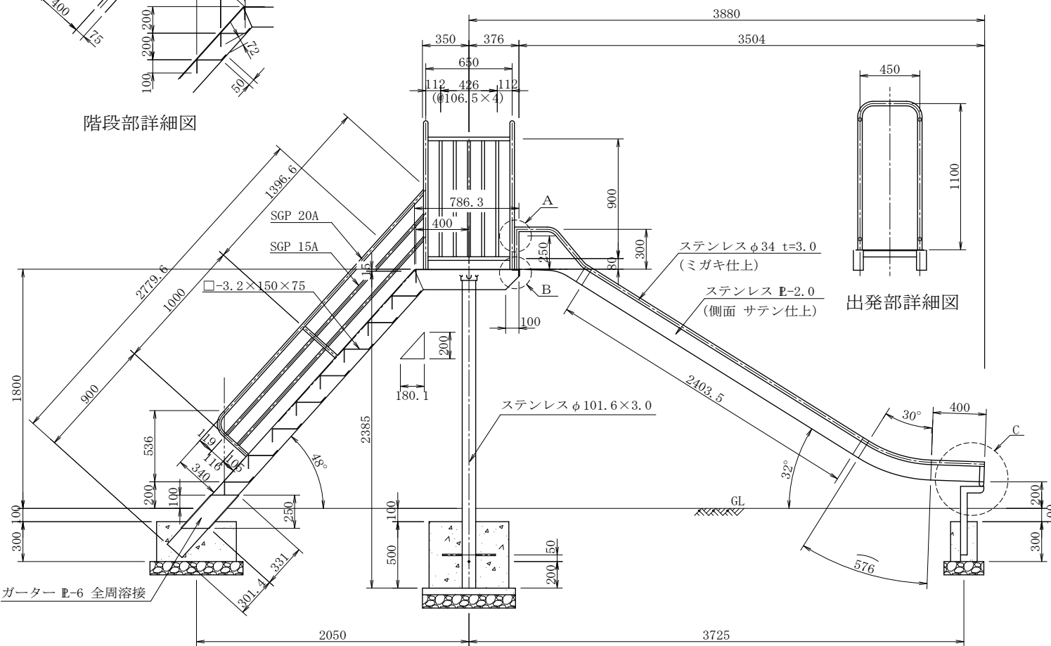
立面詳細図
