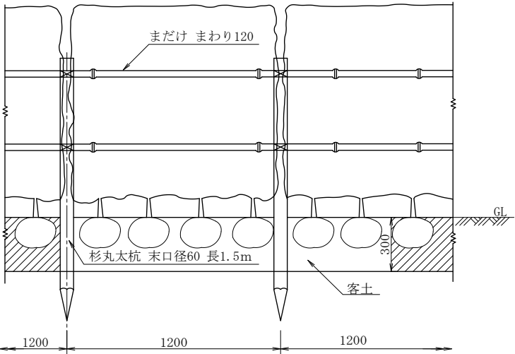
正面図
