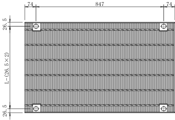
細目グレーチング
