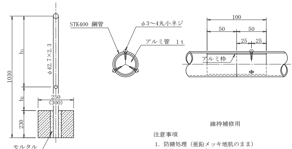
基礎工詳細図
