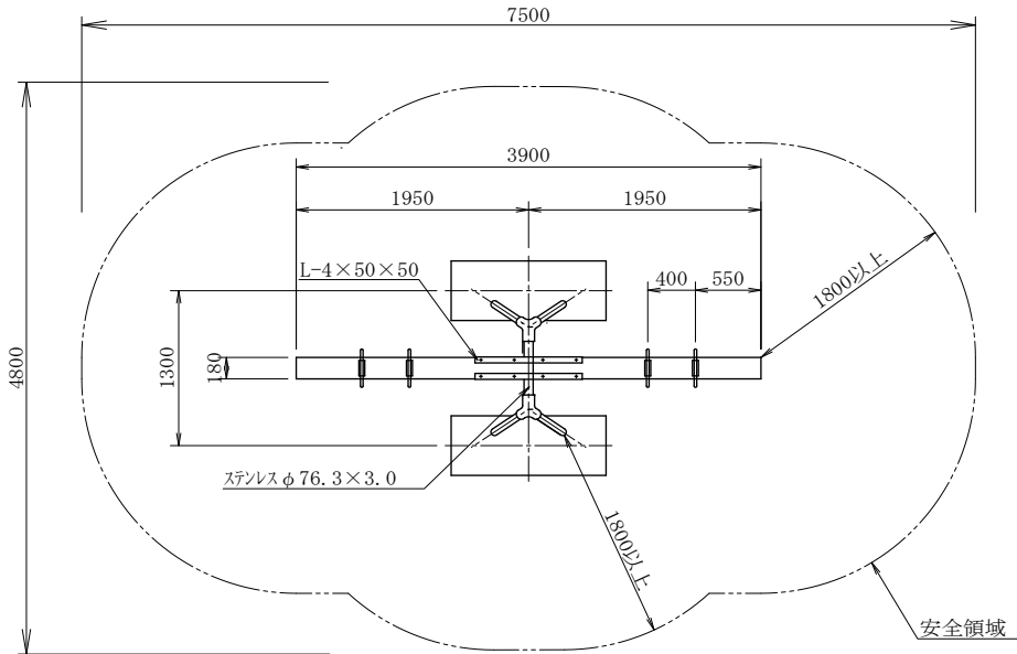
平面図
