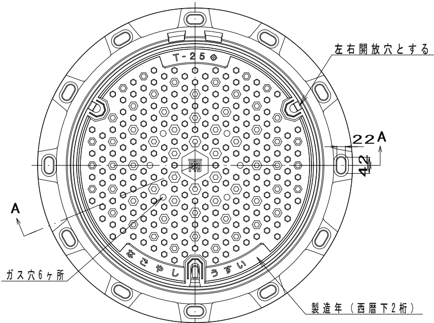
蓋, 枠平面図
