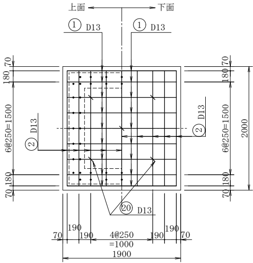
底 版
