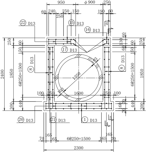
3 - 3 断 面
