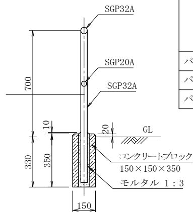
断面図 H=0.7m
