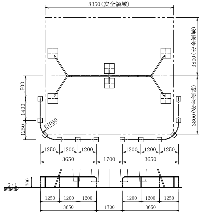
Ⓐ 地際補強参考図
