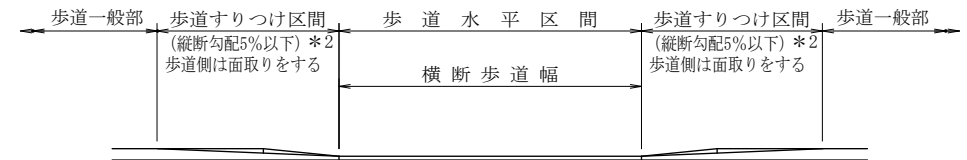
A-A'断面
