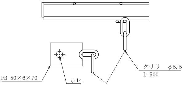
細目用クサリ・FBアンカー詳細
