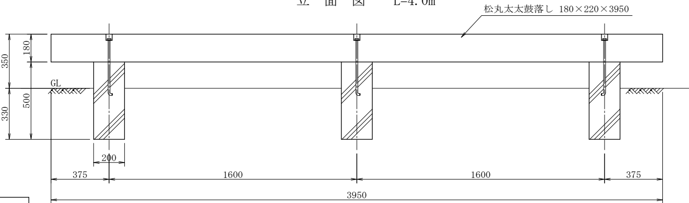
立 面 図 L=4.0m
