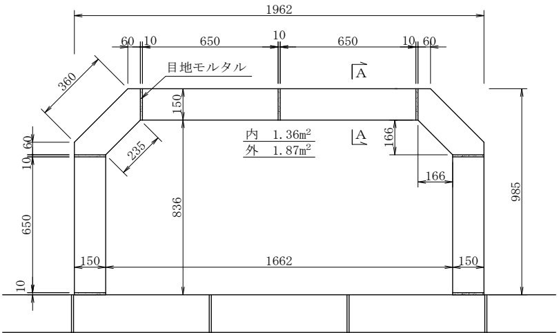
C 平 面 図
