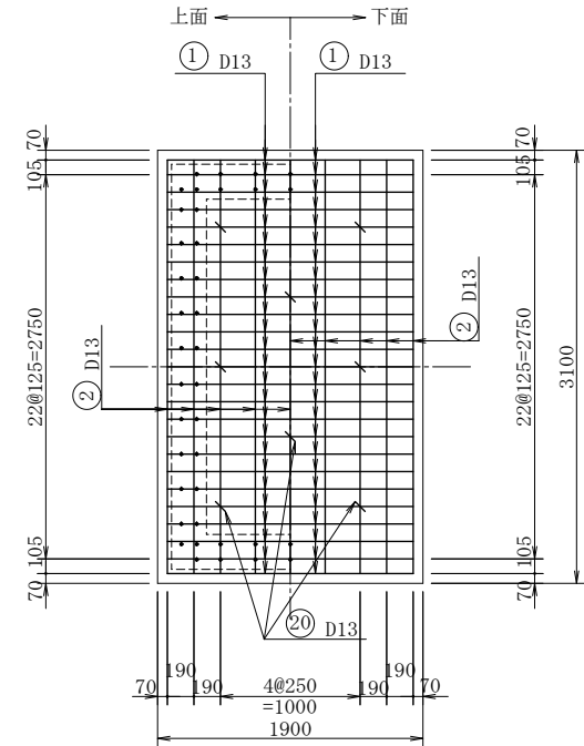
底 版
