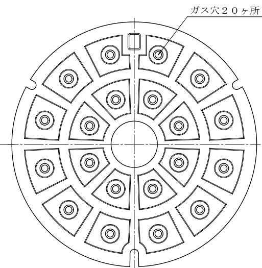
① 蓋平面図
