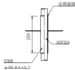
Ⓐ 地際補強参考図
