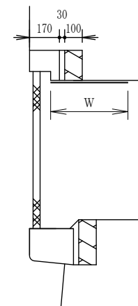
断 面 図
