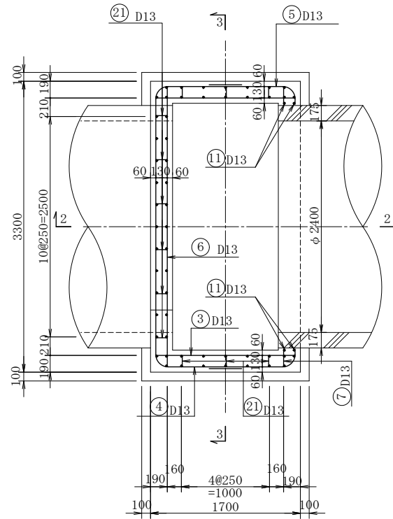
1 - 1 断 面
