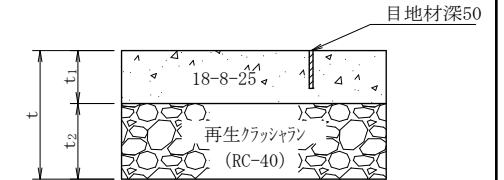
コンクリート舗装工
