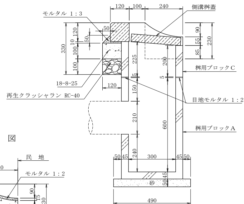
A—A 断面图
