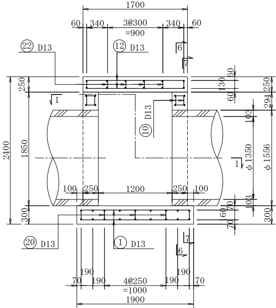
2 - 2 断 面
