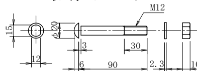
取付ボルト
