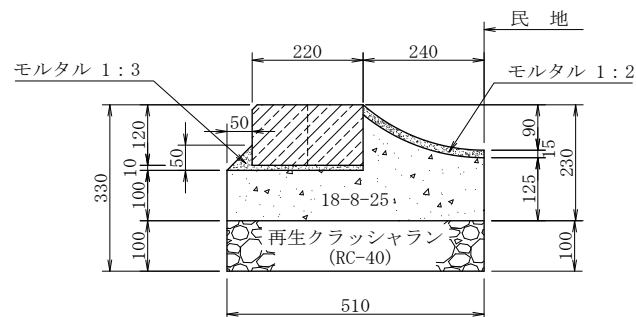
B-B 断面图
