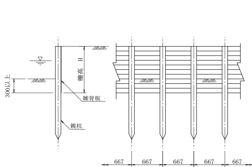
柵高 0.6m～1.0m
