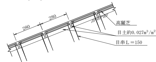
(E') 断面図
