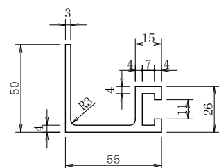
補強リブ
