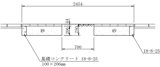
A－A 断 面 図
