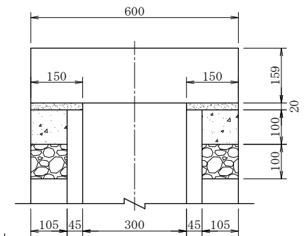
B-B 断 面 図
