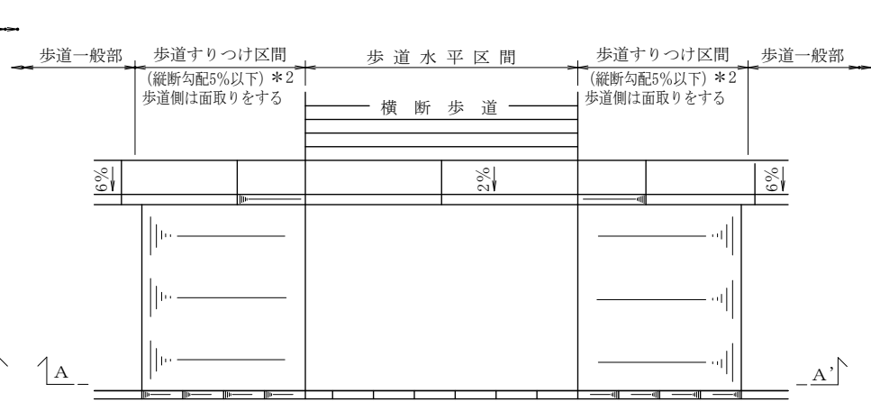
D 横断歩道の場合 平面図 歩道切下げ平面図
