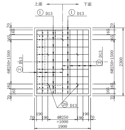
底 版
