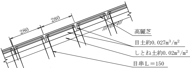
(E') 断 面 図
