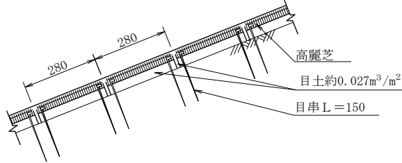
(E') 断 面 図
