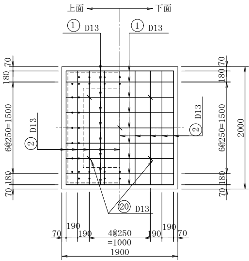
底 版
