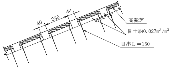
(B') 断 面 図
