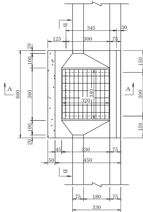
平 面 図
