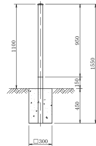
断 面 図
