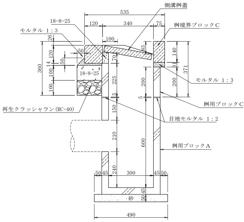
A-A 断 面 図
