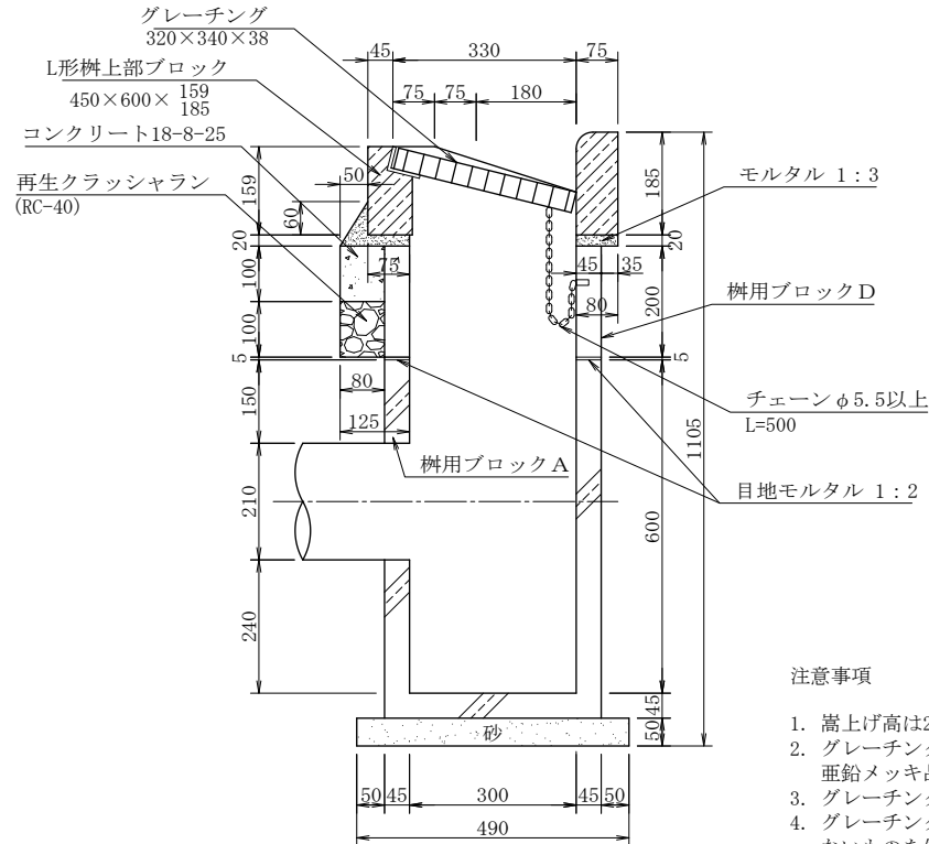
A-A 断 面 図
