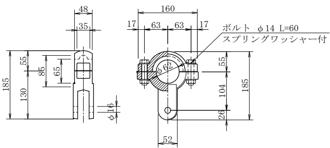
鑄鉄回転軸詳細図
