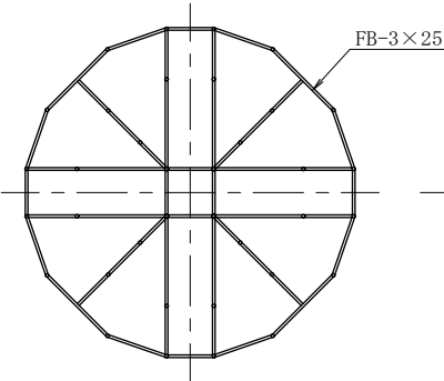
A 断面図
