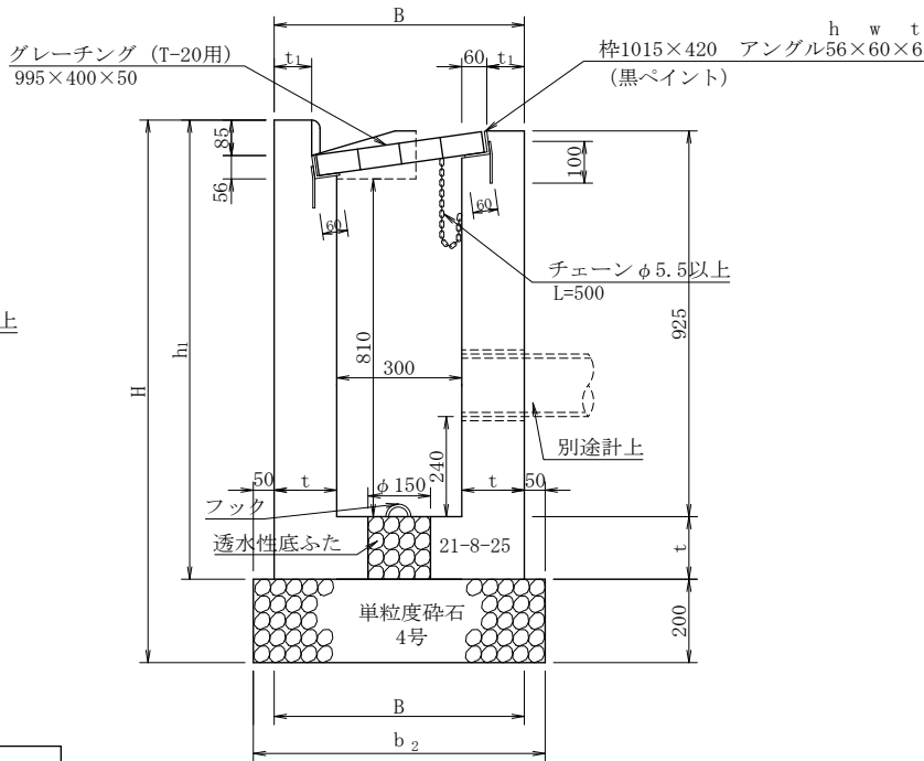
A-A 断面図
