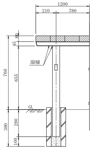
正 面 図
