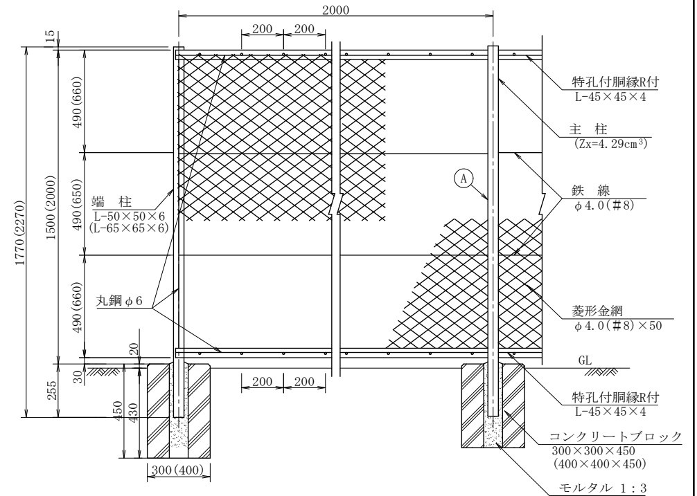
正面図 H=1.5m, H=2.0m
