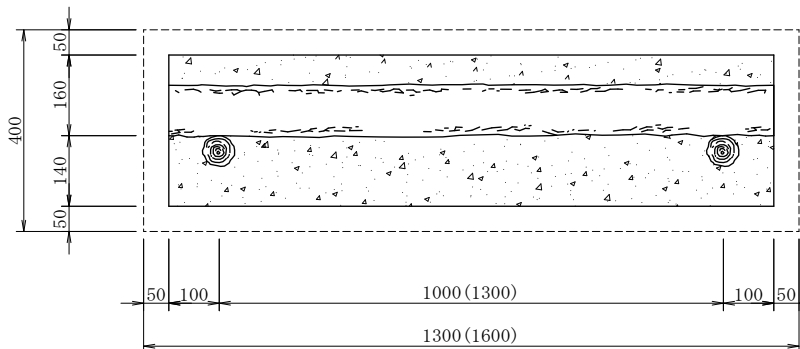
平 面 図
