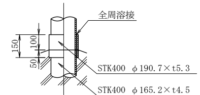
① 地際補強図
