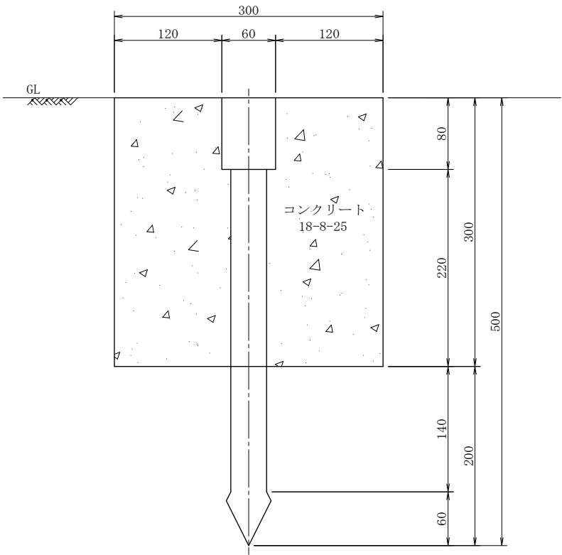
断 面 図
