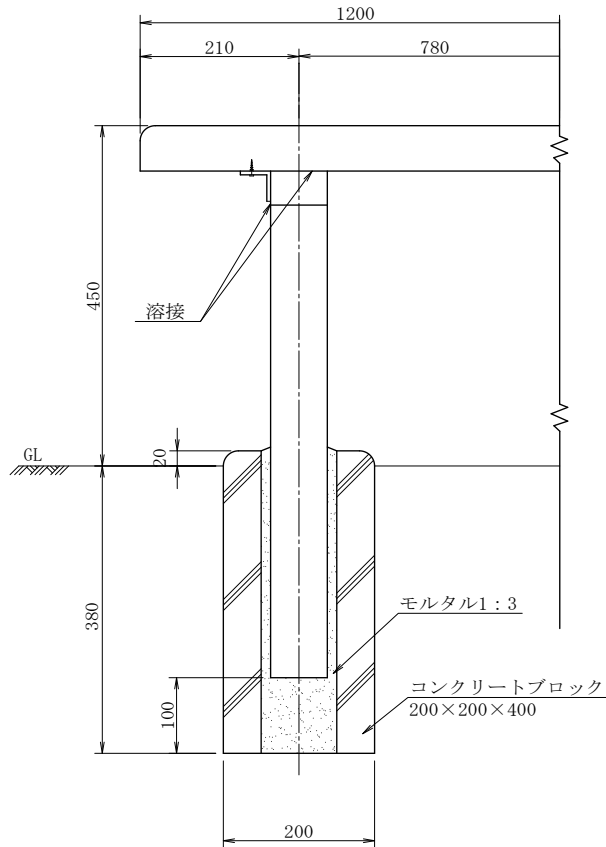
正面図
