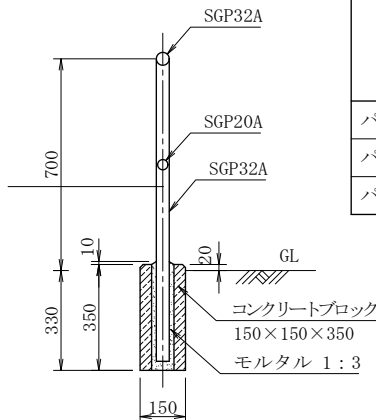
断面図 H=0.7m
