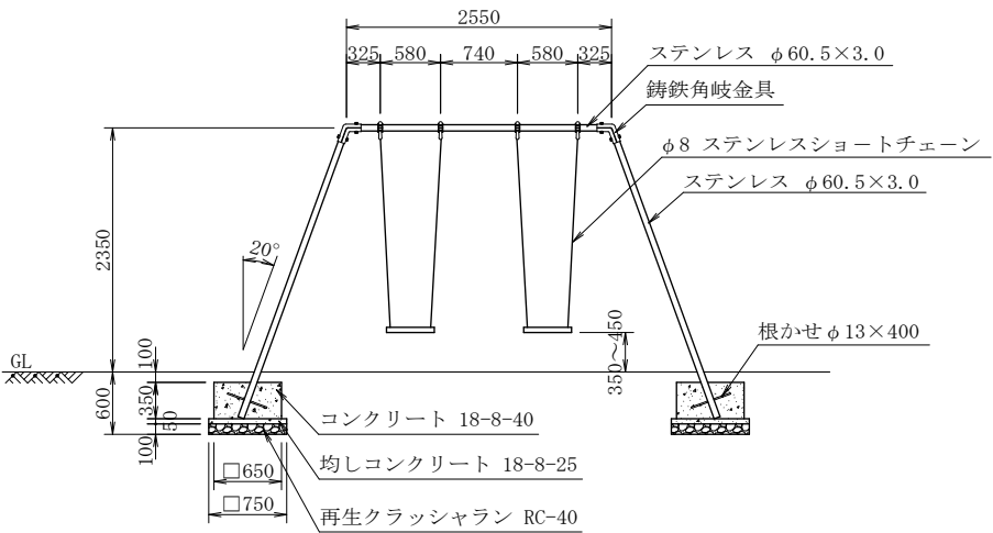
正 面 図
