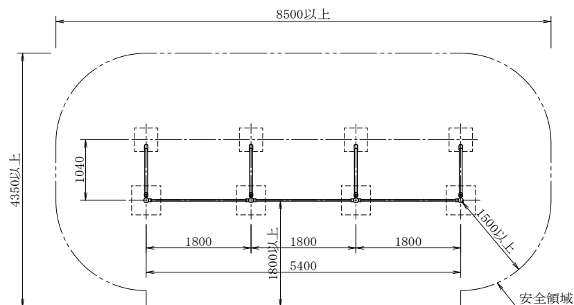
平面图
