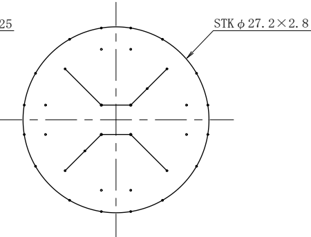
C 断面図
