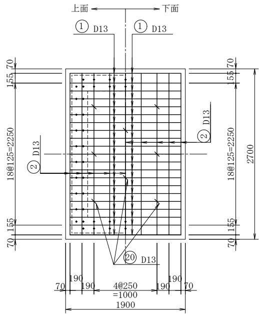
底 版
