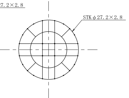
D 断面図
