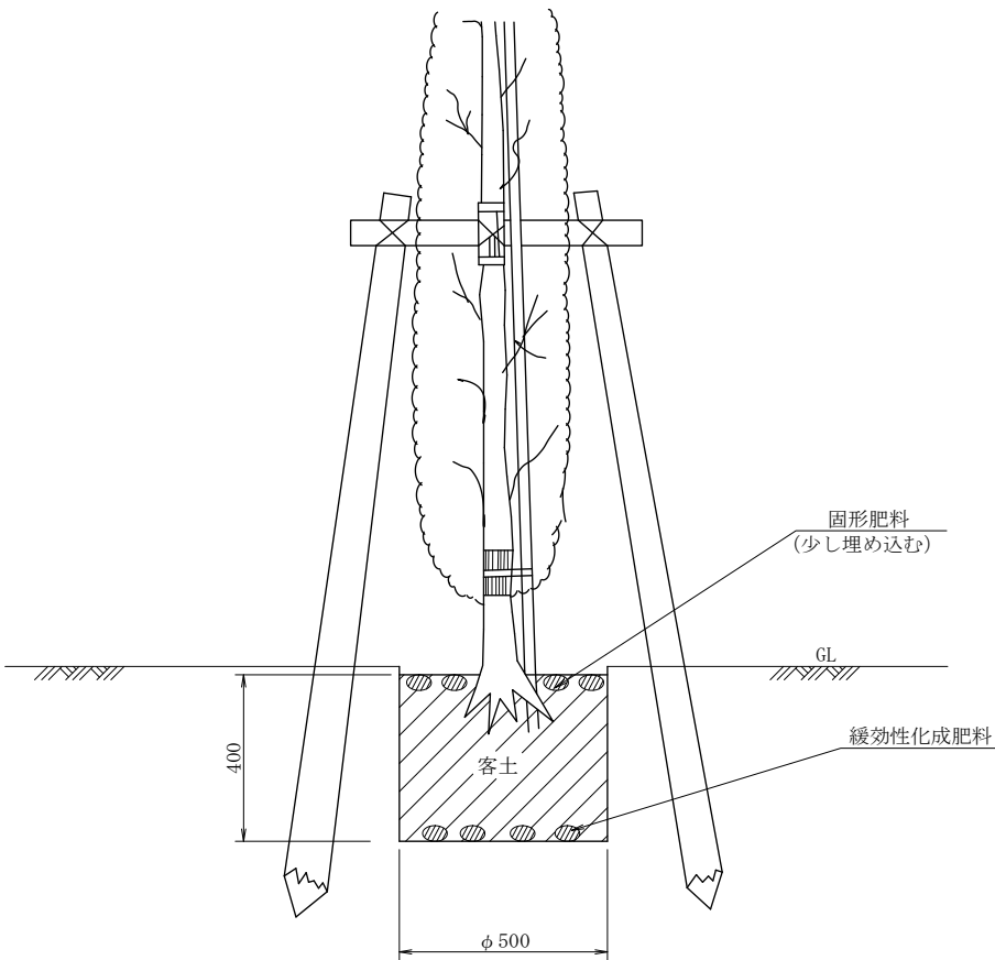
断 面 図
