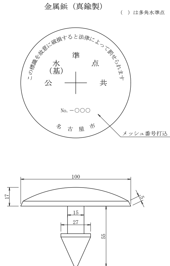
測量標(水準点・多角水準点)設置工材料表
