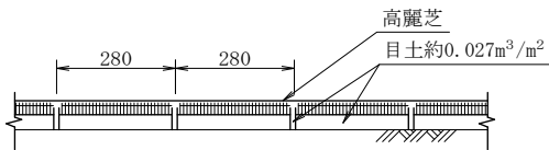
(D') 断 面 図
