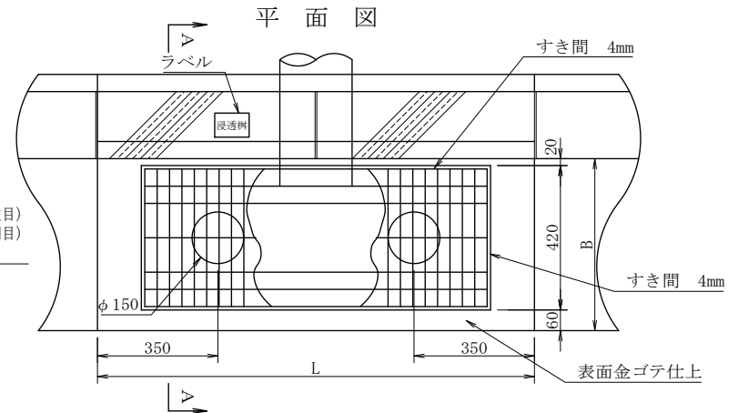
名 称 寸 法 単位 (mm) 摘 要 B b 1 b 2 b 3 b 4 H h 1 h 2 h 3 h 4 h 5 t t 1 t 2 L 街渠柵工 500B用 現 場 打 560 205 255 600 700 1270 250 150 210 120 1050 150 90 50 1270 ブロック 500 205 255 540 640 1240 250 150 240 120 1020 120 60 20 1210 街渠柵工 500C用 現 場 打 560 210 260 600 700 1320 300 200 210 170 1050 150 90 50 1270 ブロック 500 210 260 540 640 1290 300 200 240 170 1020 120 60 20 1210 街渠柵工 500A用 ブロック 500 170 220 540 640 1240 200 150 240 120 1020 120 60 20 1210
