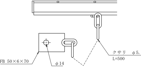
細目用クサリ・FBアンカー詳細
