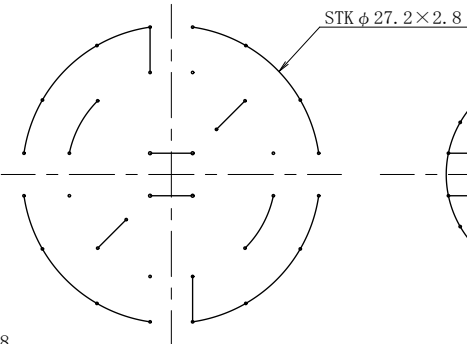
B 断面図
