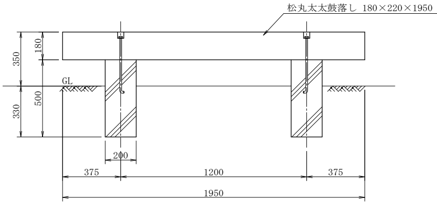
立 面 図 L=2.0m
