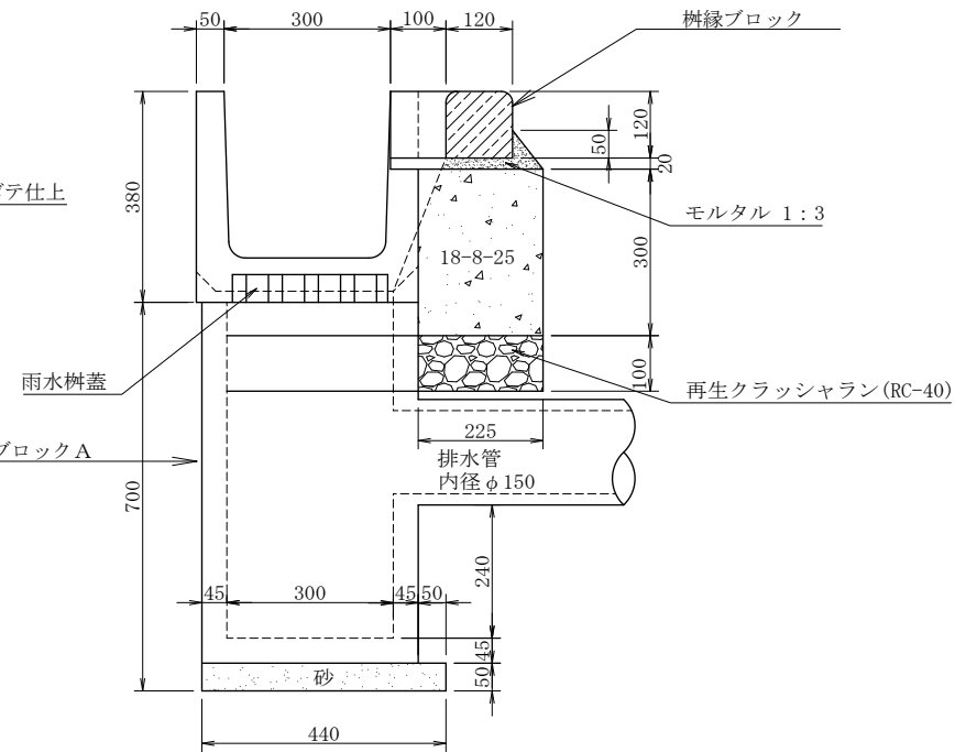
A-A 断 面 図
