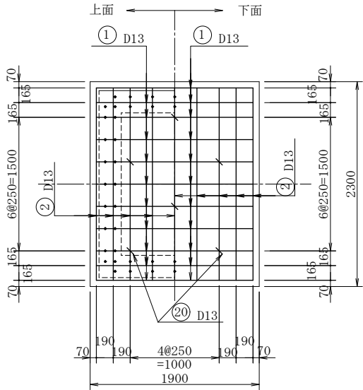
底 版
