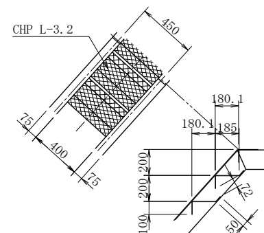
階段部詳細図
