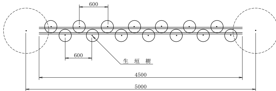
平面図
