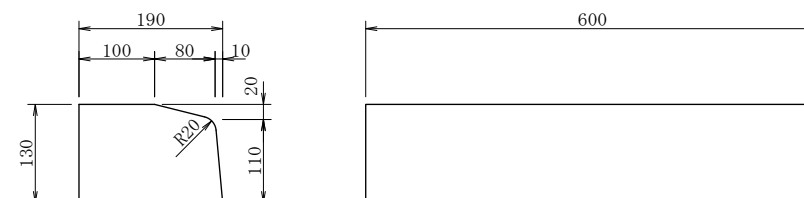
街渠工 寸 法 表 名 称 寸 法 表 単位 (mm) 摘 要 B H H' T b h 1 h 2 h 3 街渠工D 375 30 10 200 605 70 310 100 歩行者系道路に適用
