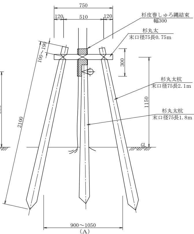
側 面 図
