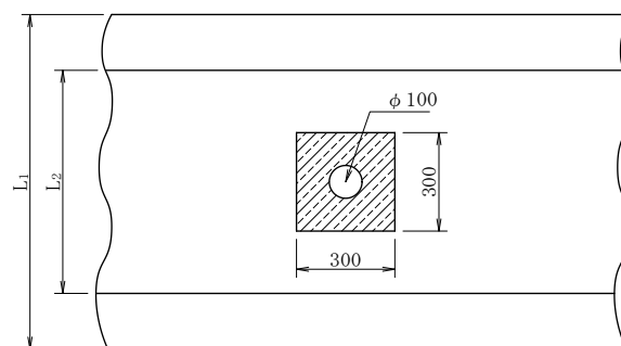
平面图
