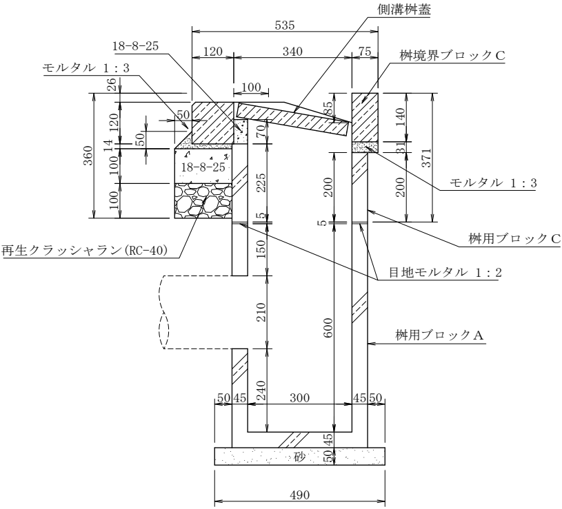
A-A 断面図
