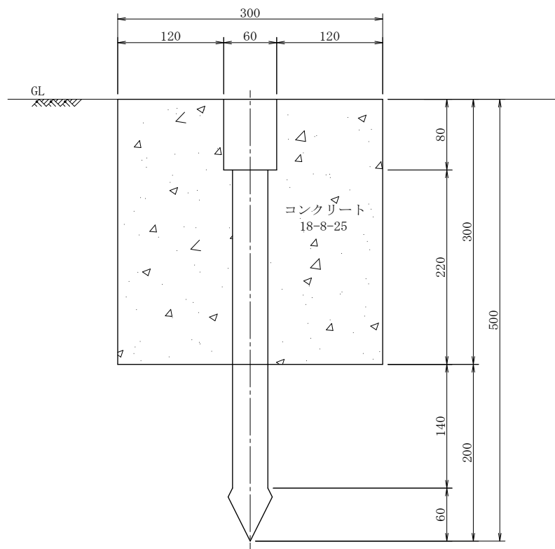
断 面 図
