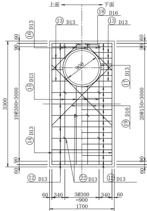
頂 版
