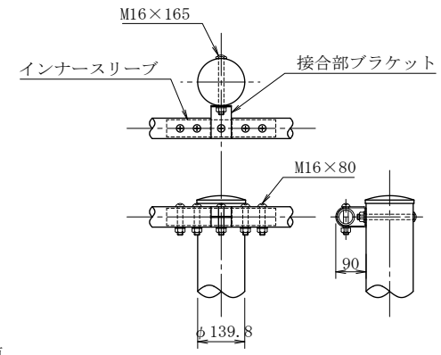
接合部詳細図
