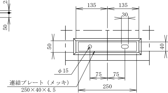
連結部詳細図
