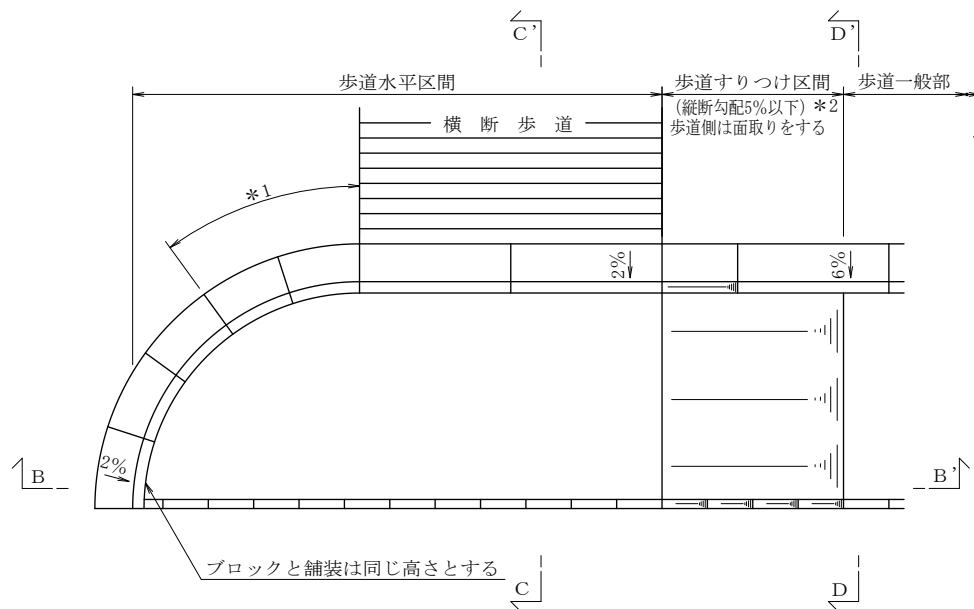
平 面 図
