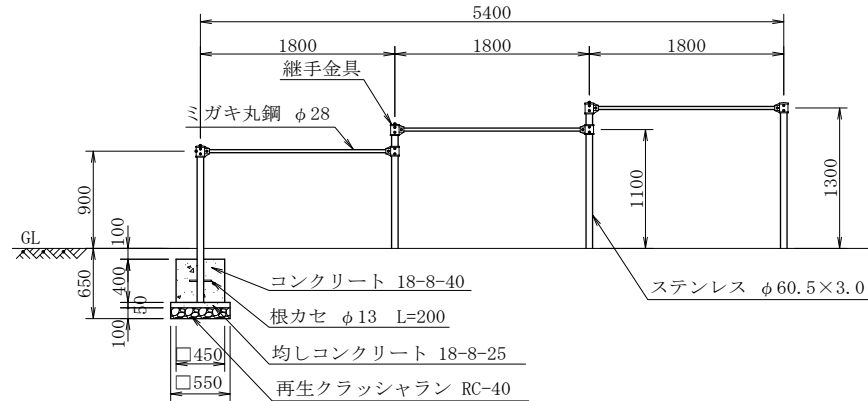
正 面 図
