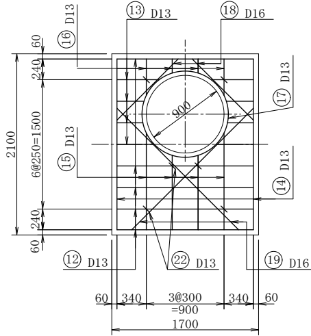
頂 版 上・下面共通
