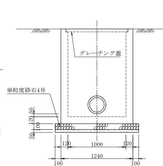
C-C 断面図
