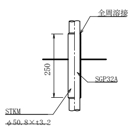
Ⓐ 地際補強参考図
