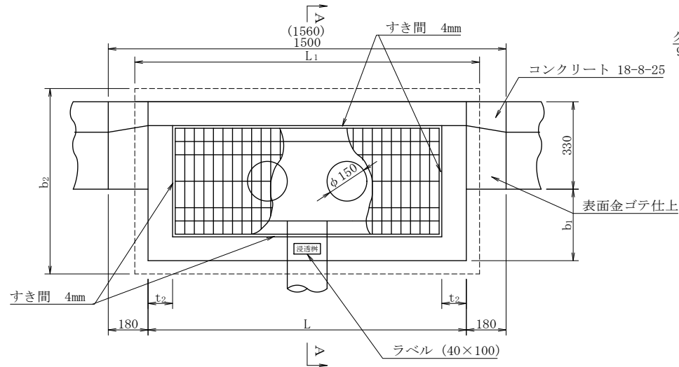
平 面 図
