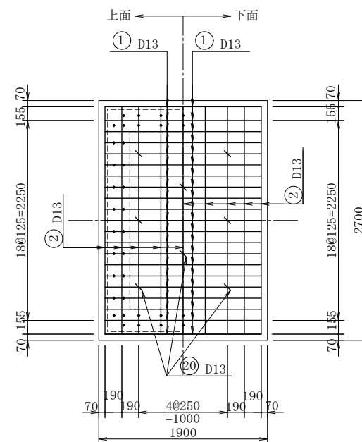
底 版
