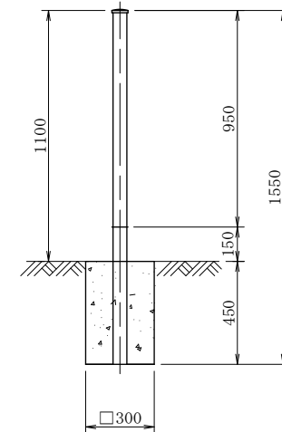
断 面 図
