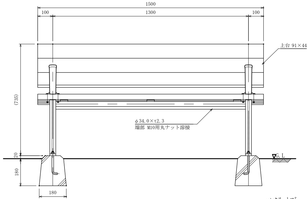
取合詳細図
