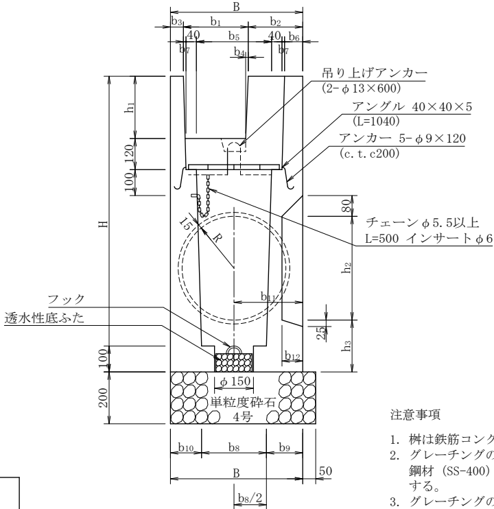
A-A 断面図
