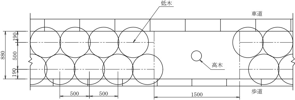
標 準 平 面 図
