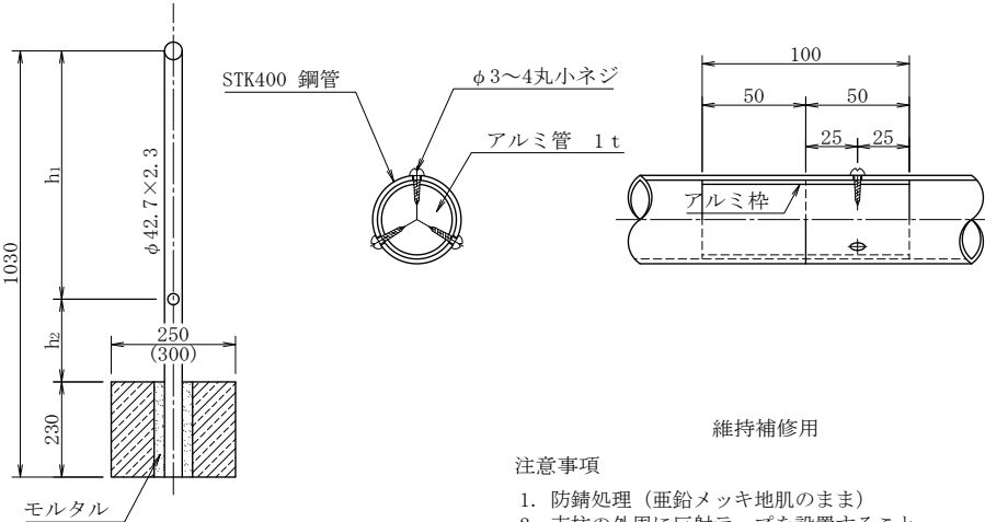
基礎工詳細図
