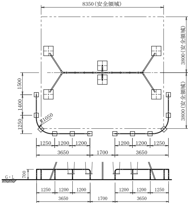
四連ブランコ（児童用） 四連用（R型）
