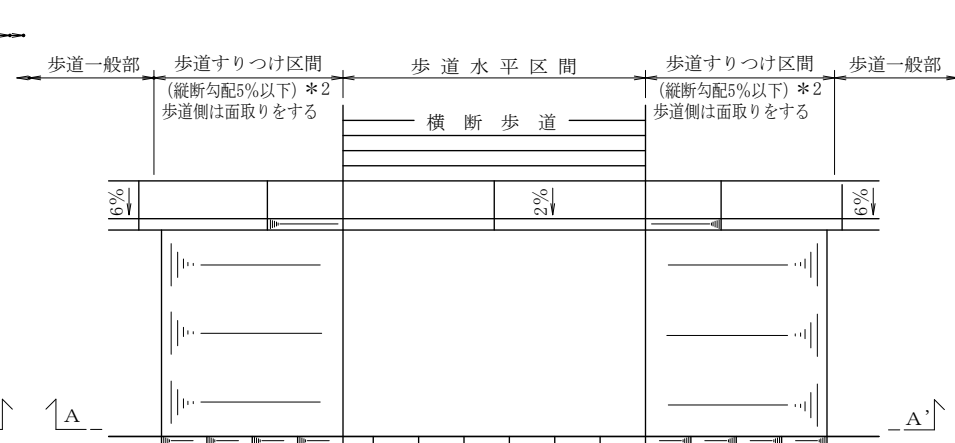
歩道切下げ平面図
