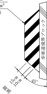
正面図
