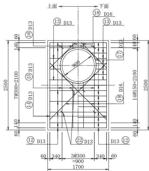
頂 版
