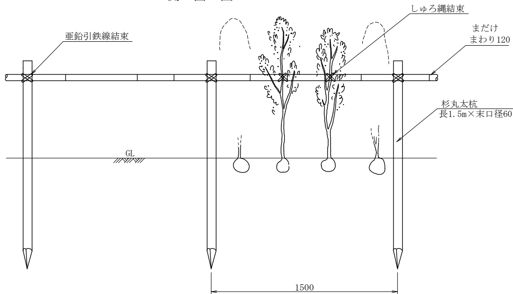
側面図
