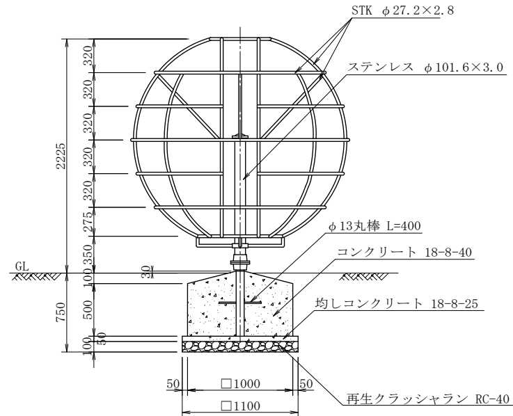
立面図
