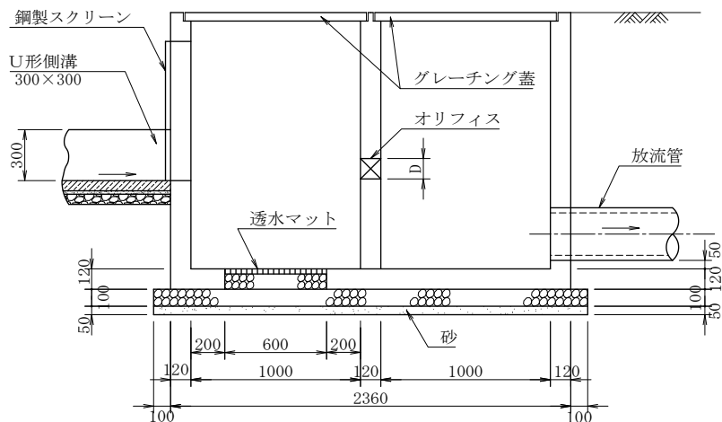
A-A 断面図
