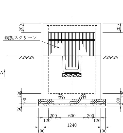
B-B 断面図
