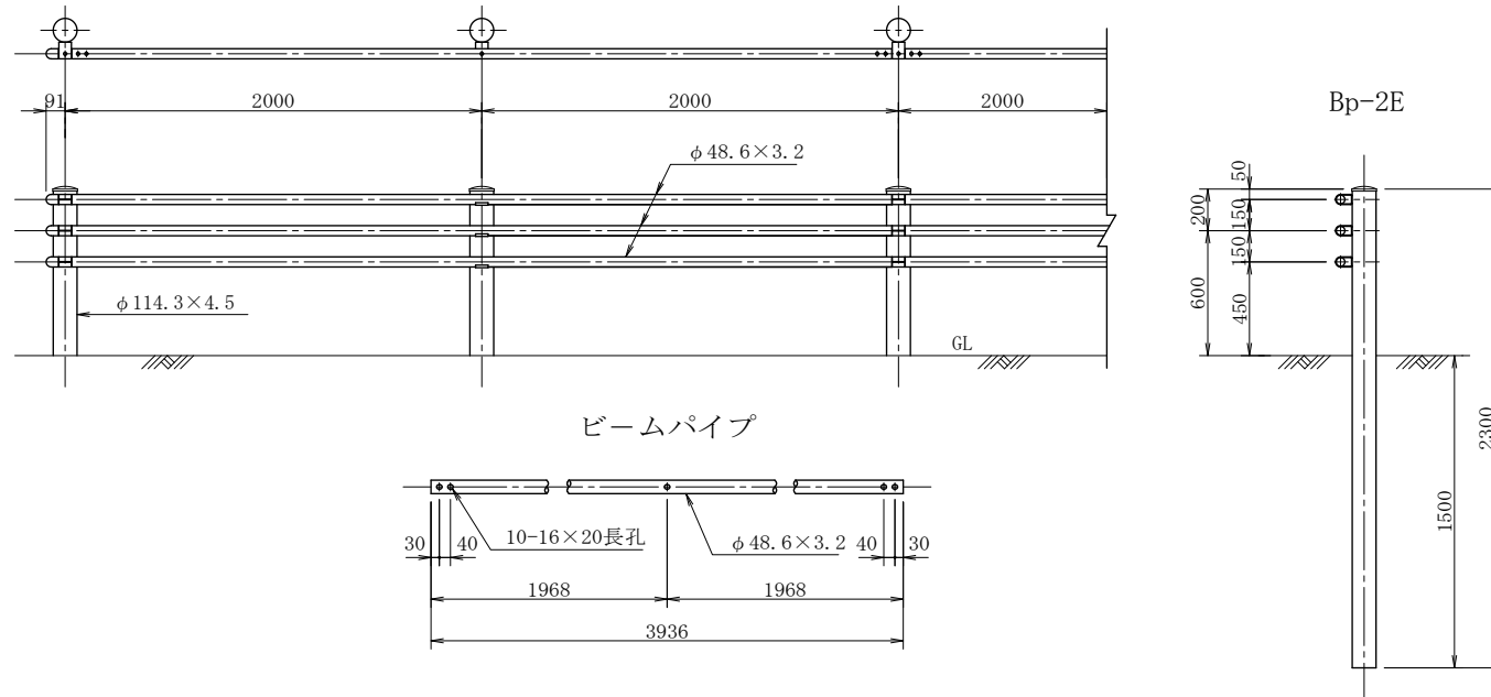
端部詳細図
