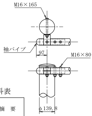
端部詳細図
