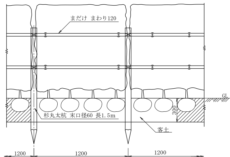
正面図
