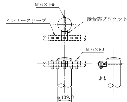
接合部詳細図
