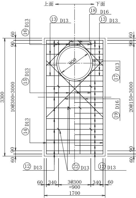
頂 版
