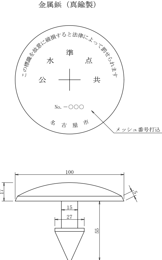
測量標(水準点)設置工材料表
