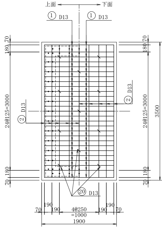
底 版
