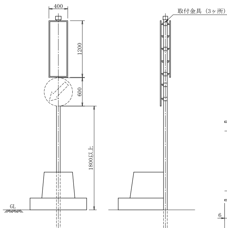
正 面 図
