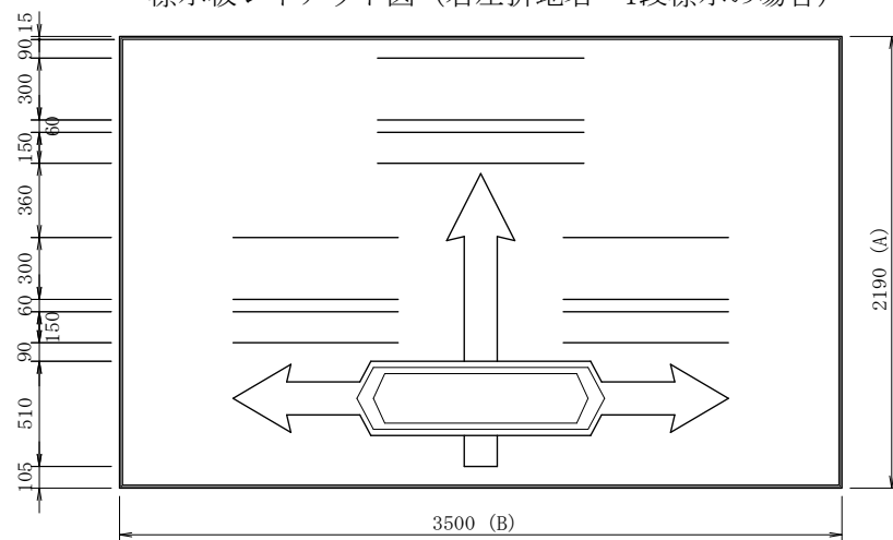
標示板レイアウト図（右左折地名 2段標示の場合）
