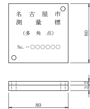
蓋取付用名板
