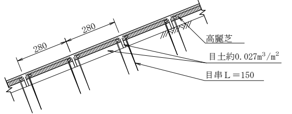
(E') 断 面 図
