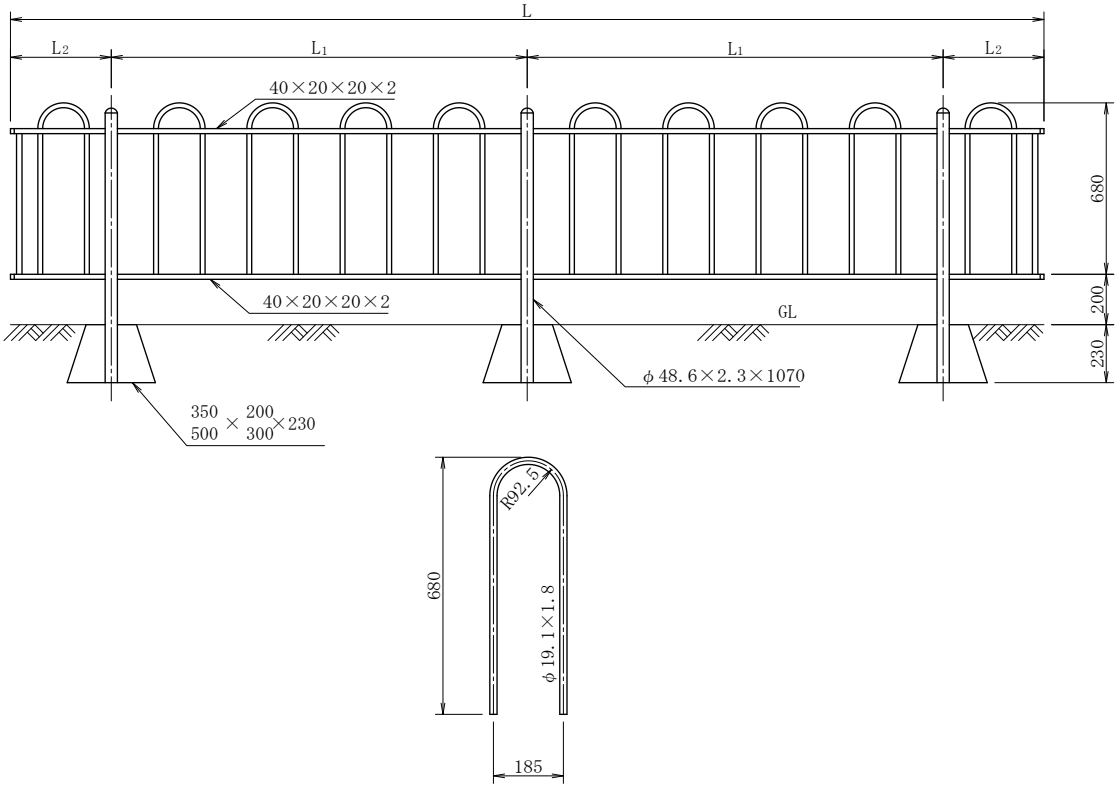
側面図
