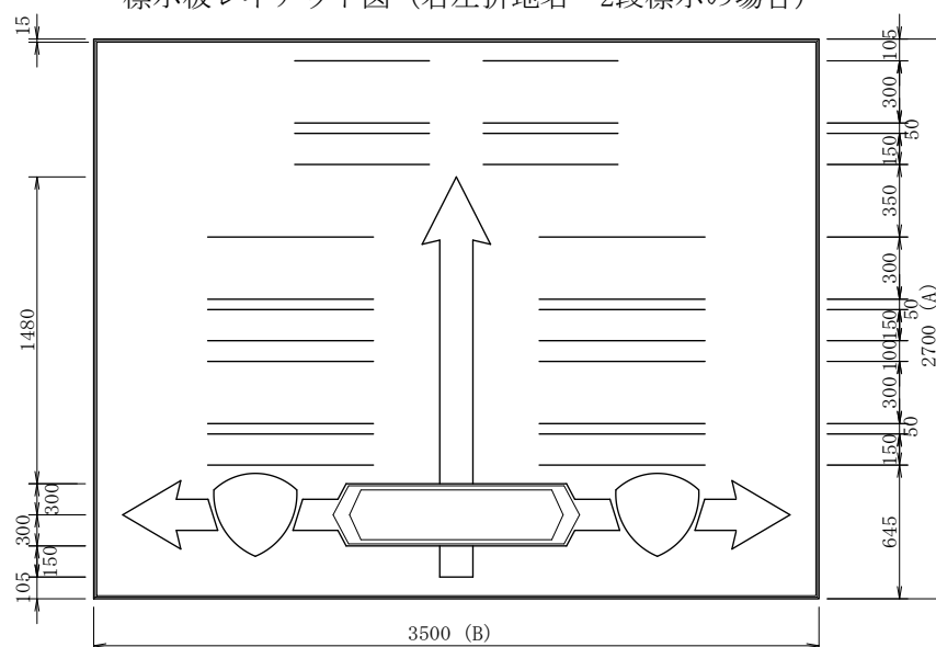
標示板レイアウト図（右左折地名 2段標示の場合）
