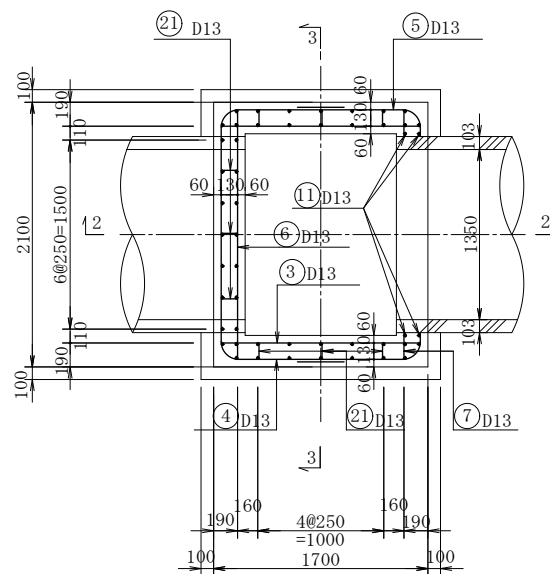
1 - 1 断 面
