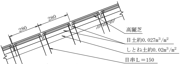
(E') 断 面 図
