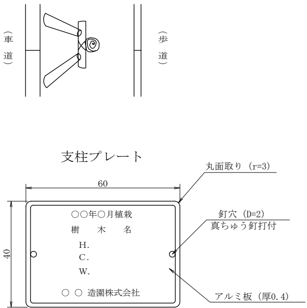
平 面 図
