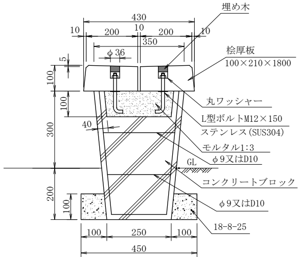
断面図
