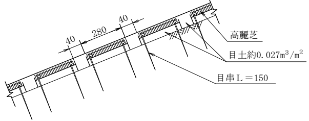
(B') 断 面 図
