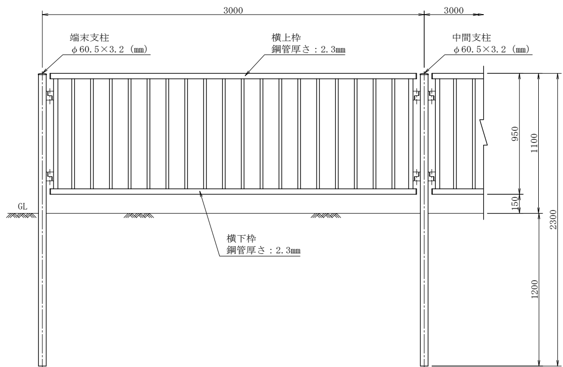
組立図
