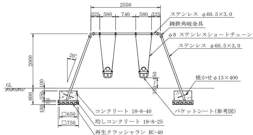
正 面 図
