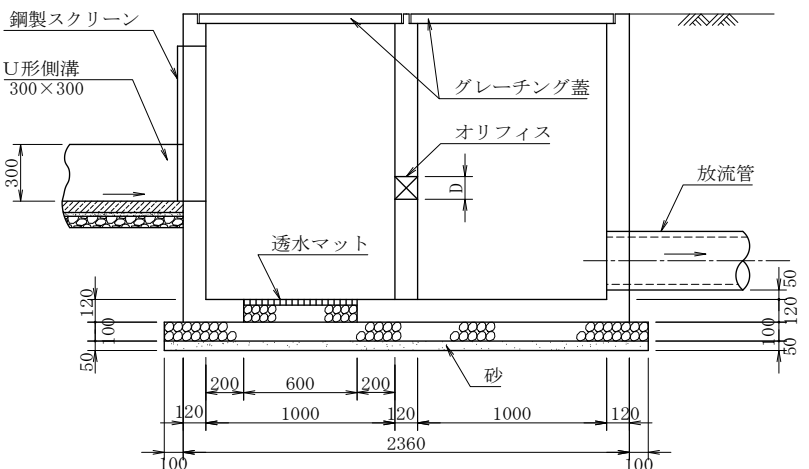
A-A 断面図
