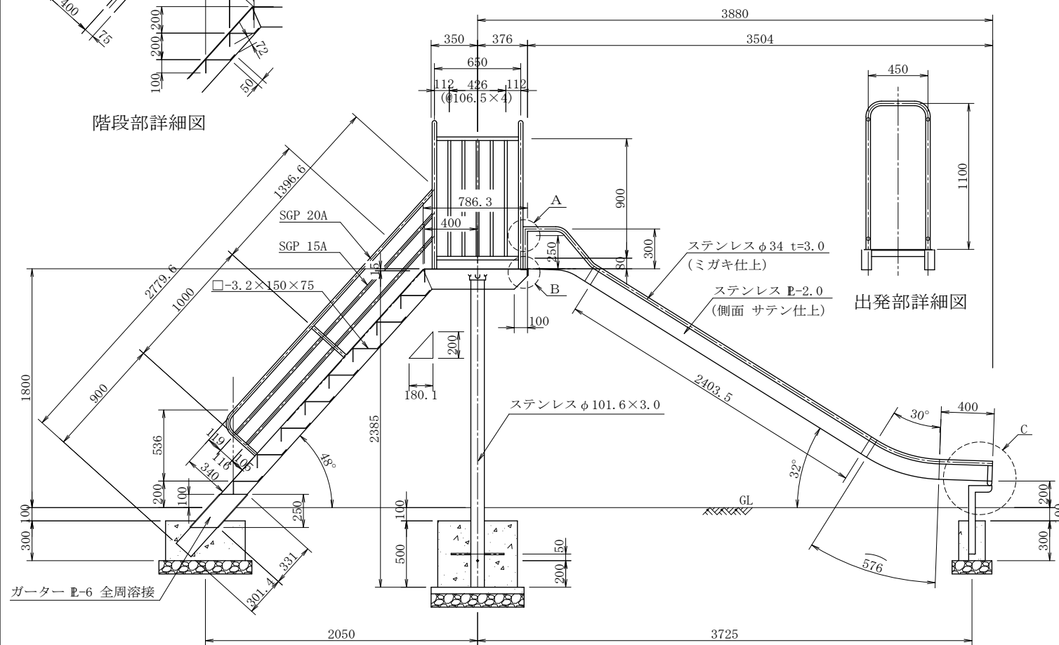
立面詳細図
