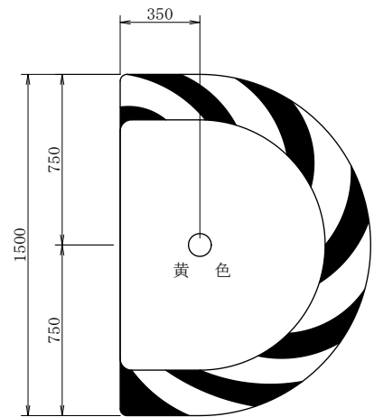
側 面 図
