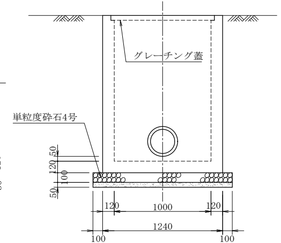
C-C断面図
