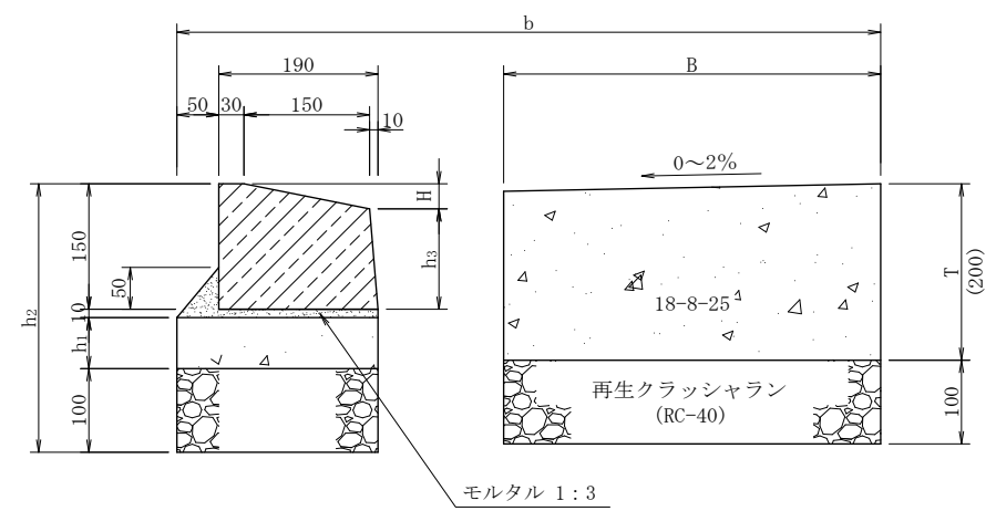
ブロック寸法
