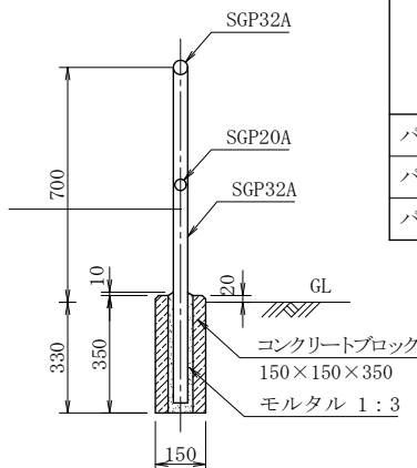
断面図 H=0.7m
