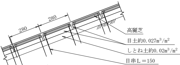
(E') 断 面 図
