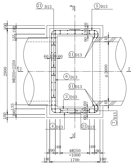
1 - 1 断 面
