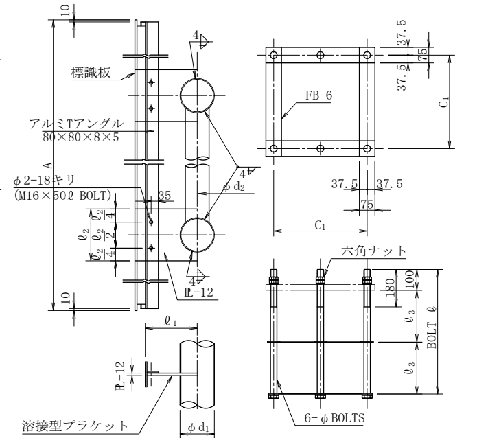
アンカーボルト詳細図
