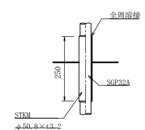
Ⓐ 地際補強参考図
