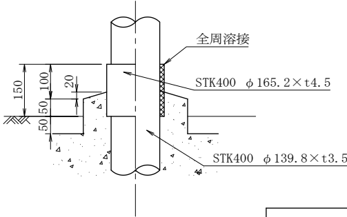
① 地際補強図
