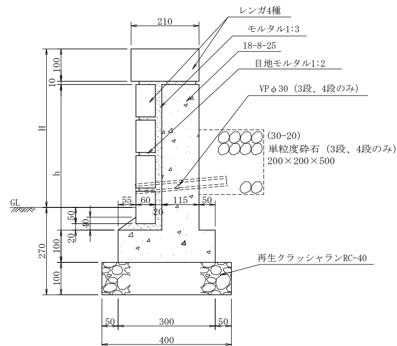
断面図
