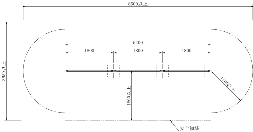
平 面 図
