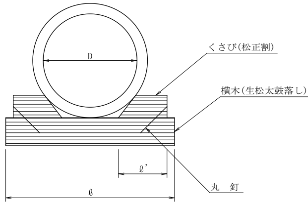
まくら土台基礎工材料表
