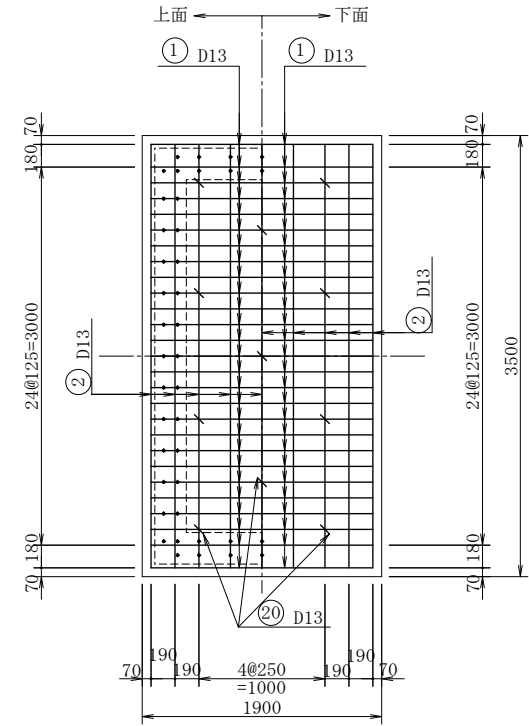
底 版
