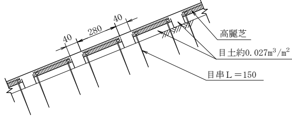
(B') 断 面 図
