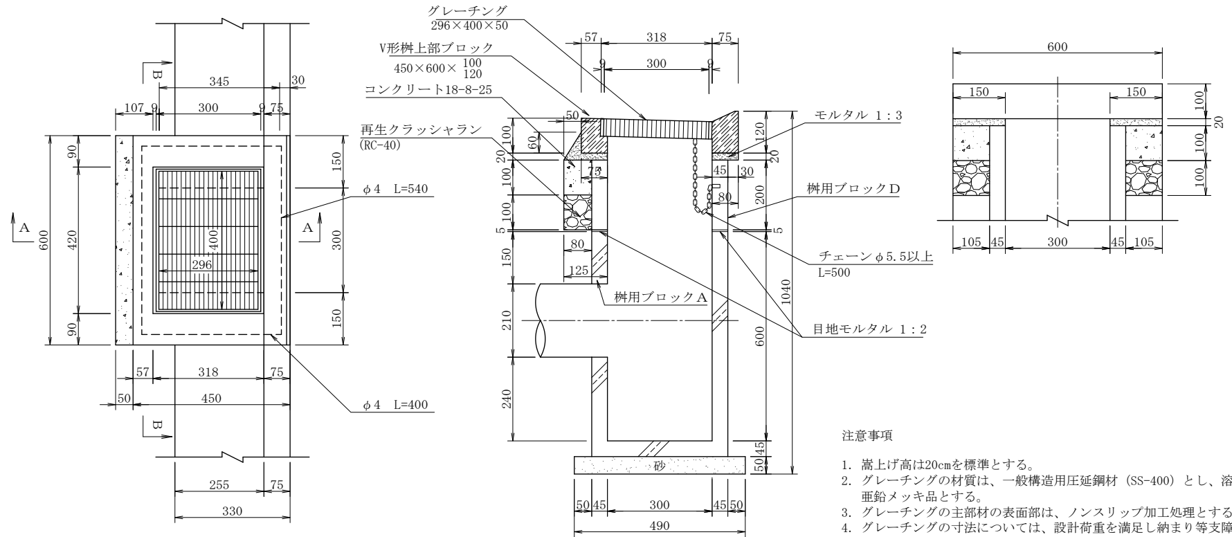
B—B 断面图
