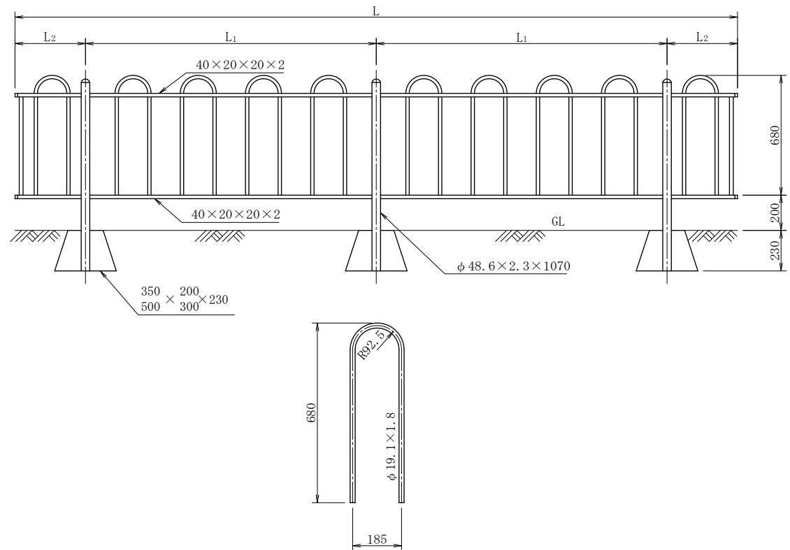
側面図
