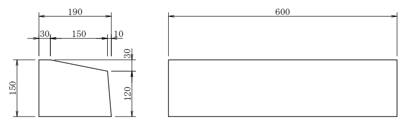
ブロック寸法
