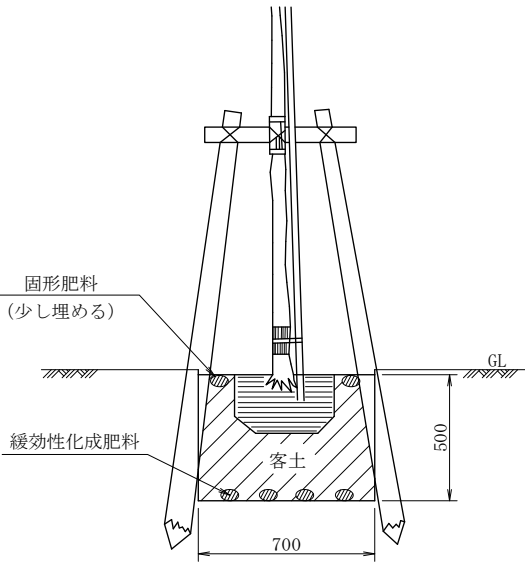
断 面 図
