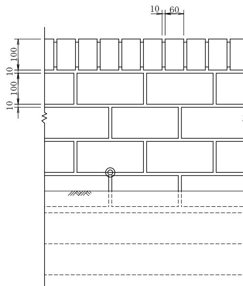
正面图
