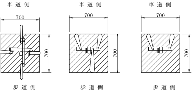
平 面 図
