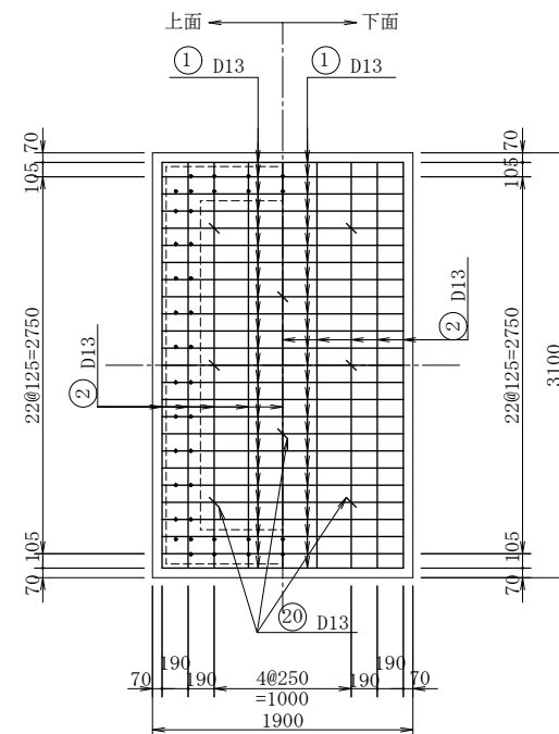
底 版
