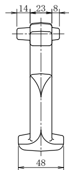
③ 蝶番金物詳細図
