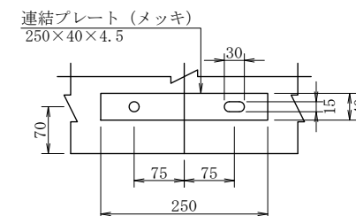
連結部詳細図
