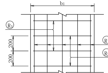
P3型(管きょ: 360° 固定基礎)寸法および材料表
