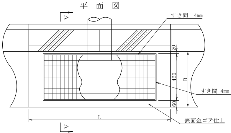
街渠枳工 (500A, 500B, 500C用) 寸法表
