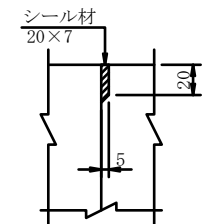
接合部詳細図
