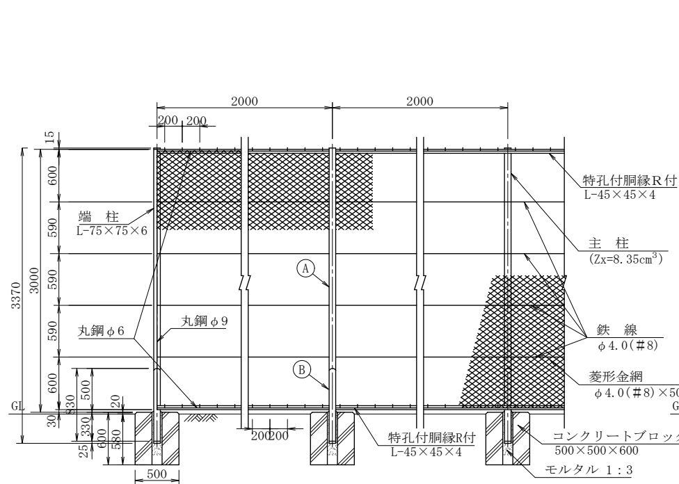
正面図
