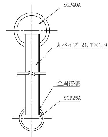
接 続 部 詳 細 図
