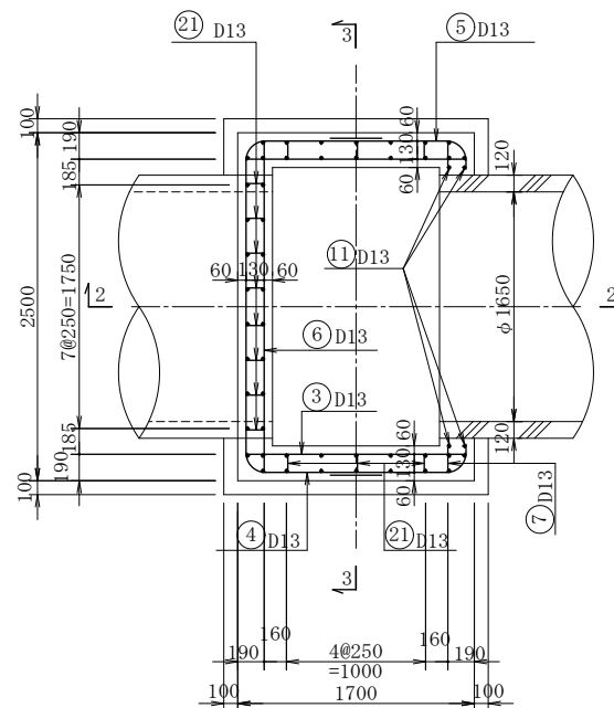
1 - 1 断 面
