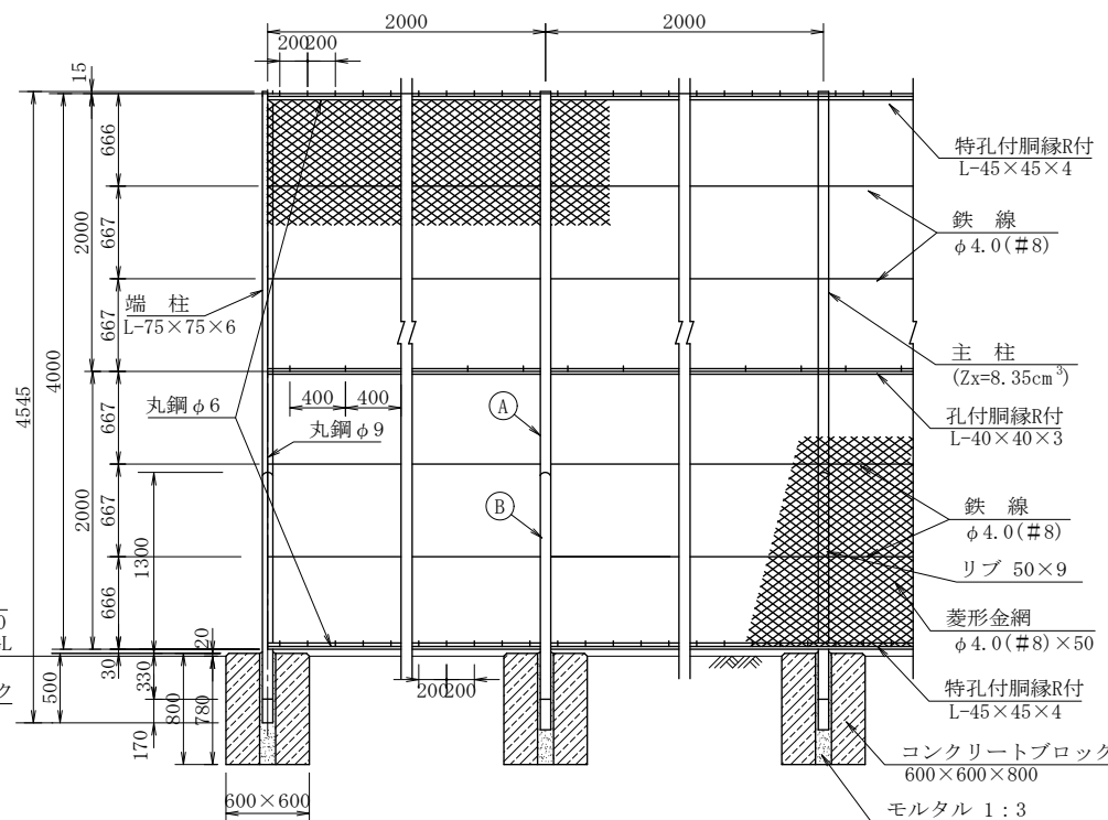
主柱(A)部断面参考図
