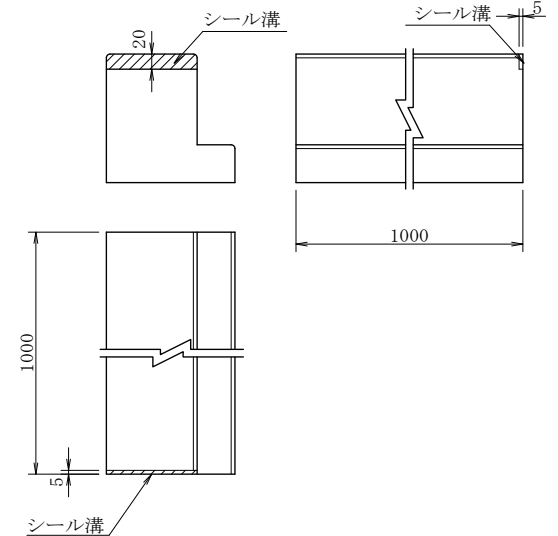
接合部詳細図
