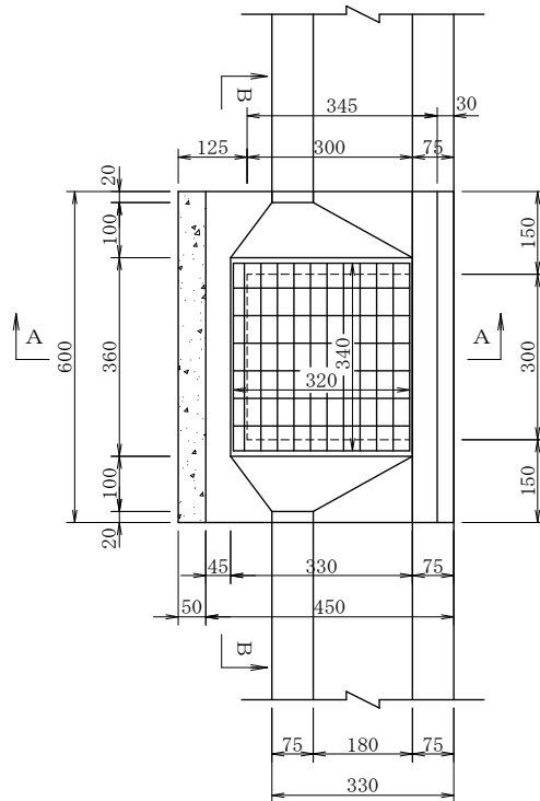
グレーチング 320×340×38 L形樹上部ブロック 450×600× \frac{159}{185} コンクリート18-8-25 再生クラッシュラン (RC-40) モルタル 1:3 樹用ブロック D チェーンφ5.5以上 L=500 目地モルタル 1:2 樹用ブロック A 砂 注意事項 1. 嵩上げ高は200mm 2. グレーチングは、 重鉛メッキ品 3. グレーチングは、 50mm厚 4. グレーチングは、 50mm厚
