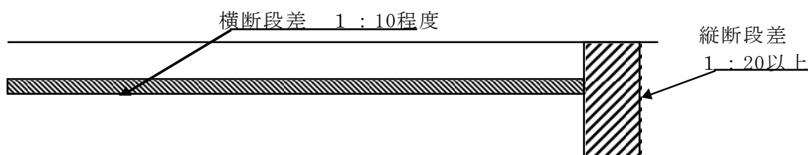
図15-1 縦・横断段差図
