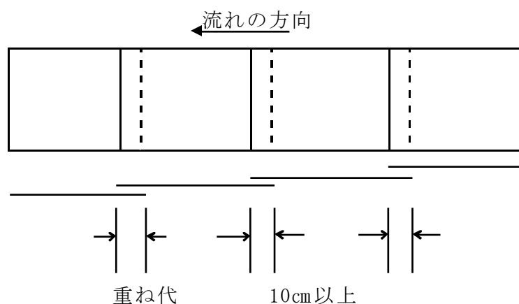
図 1 - 1 吸出し防止シートの重ね代
