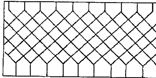
図3-2 谷積
