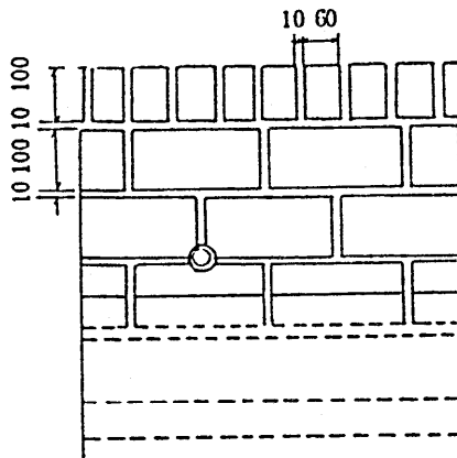
正 面 図
