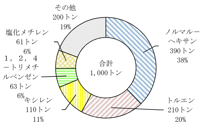
図8 大気への排出量の内訳
