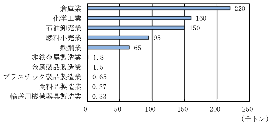
図12 取扱量の多い上位10業種
