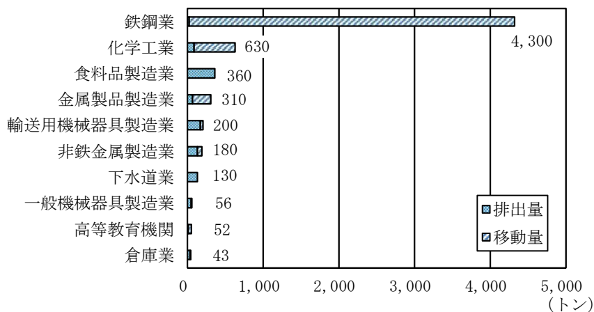
図15 排出量・移動量の多い上位10業種 (トン)
