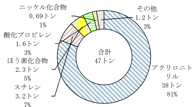
図11 下水道への移動量の内訳
