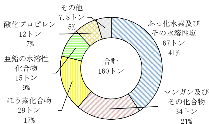
図9 公共用水域への排出量の内訳
