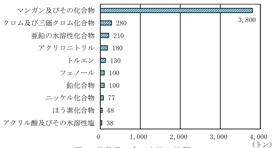
図6 移動量の多い上位10物質
