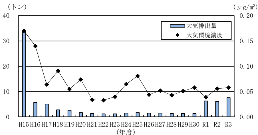
図20 酸化プロピレンの届出大気排出量と大気環境濃度
