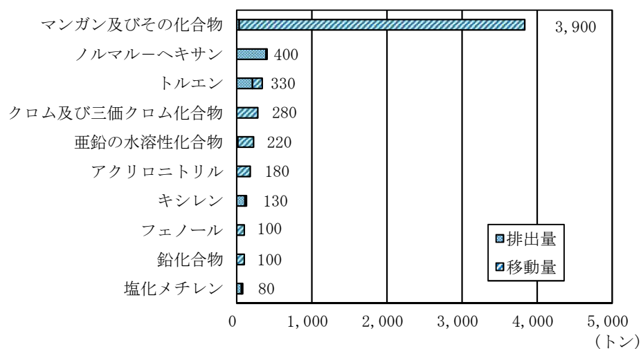
図7 排出量・移動量の多い上位10物質
