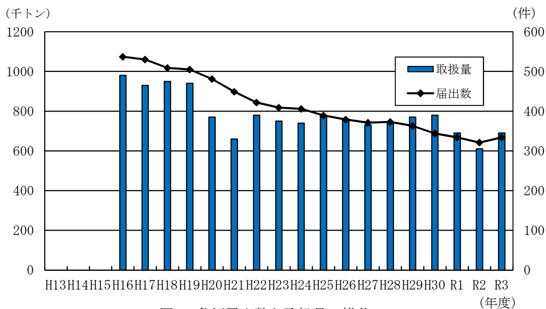
図1 条例届出数と取扱量の推移
