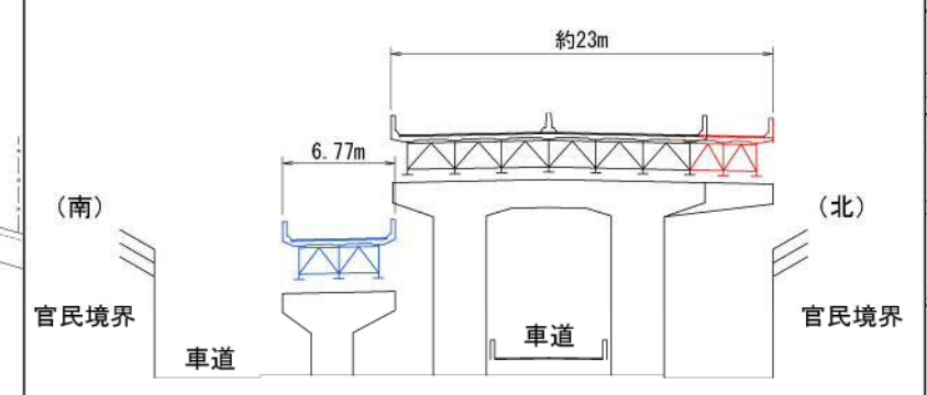
断面図 1（西行き入口）
