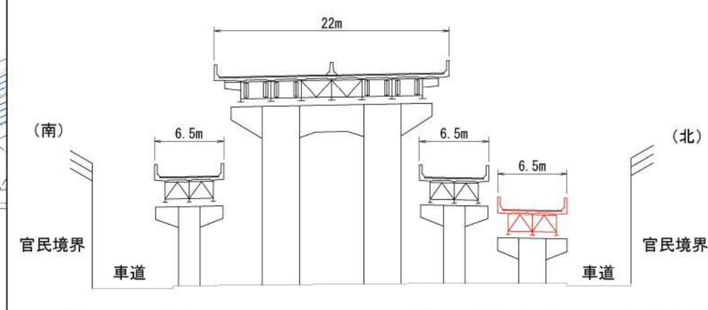
断面図 2（東行き出口）
