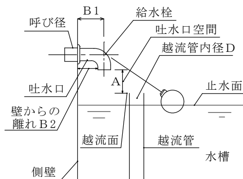
越流管（立取り出し）
