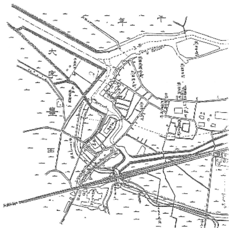
精進川の図面（明治四〇年代） （精進川改修工事竣工報告書）
