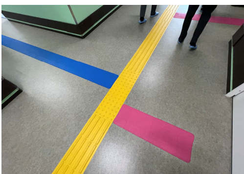
男女トイレを分別できる 誘導ブロック
