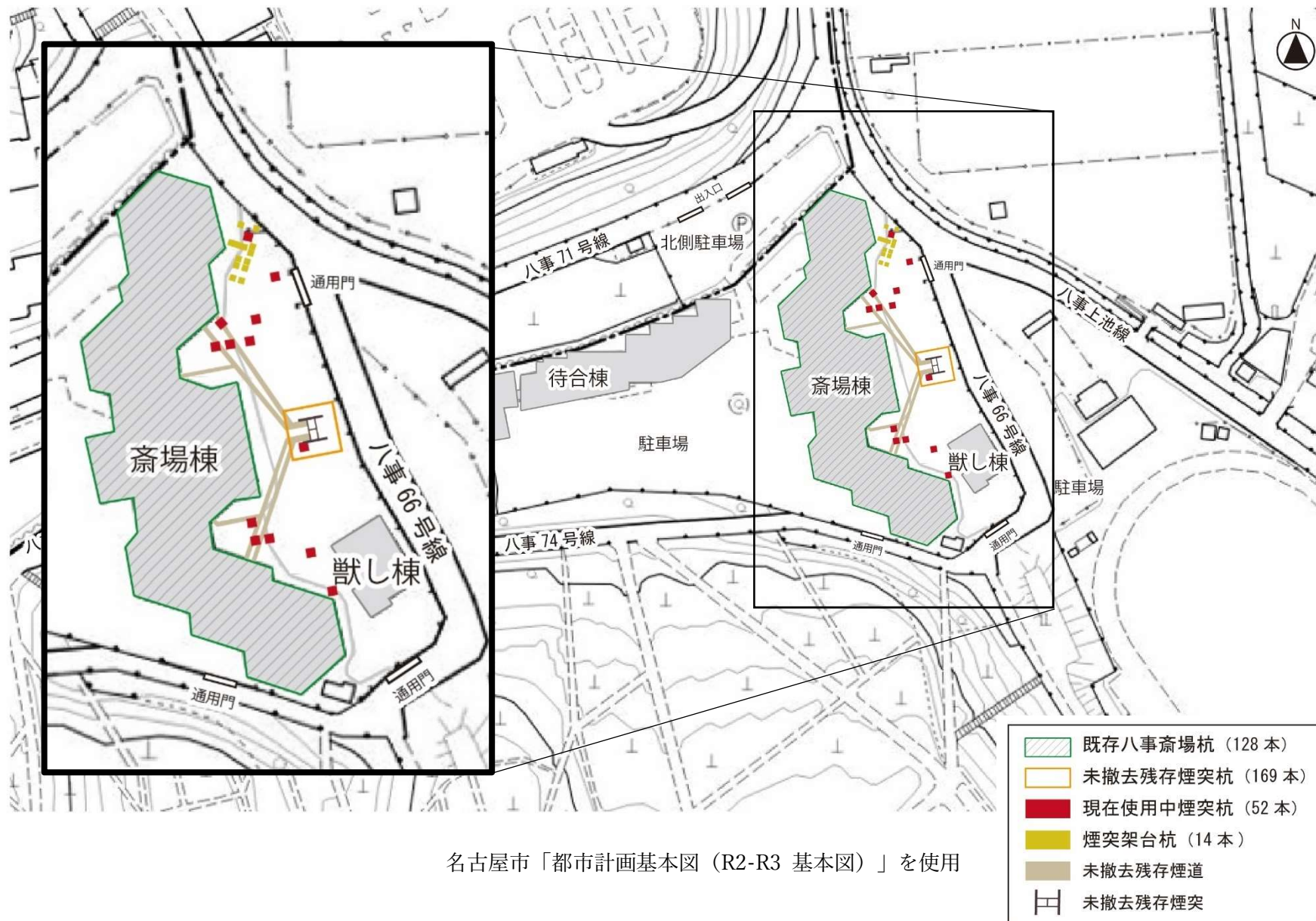
参考 d 地中障害物位置図
