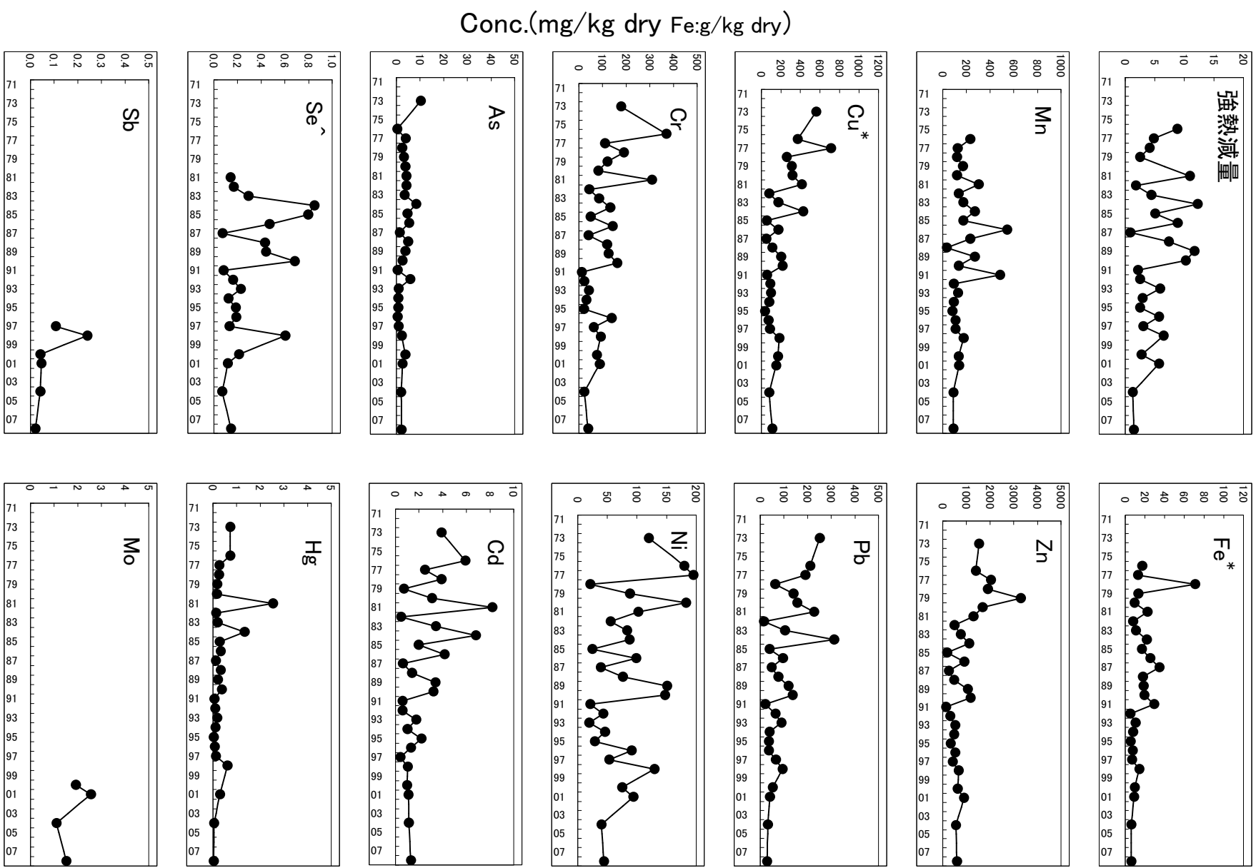
Fig.6 新堀川日の出橋の重金属経年変化
