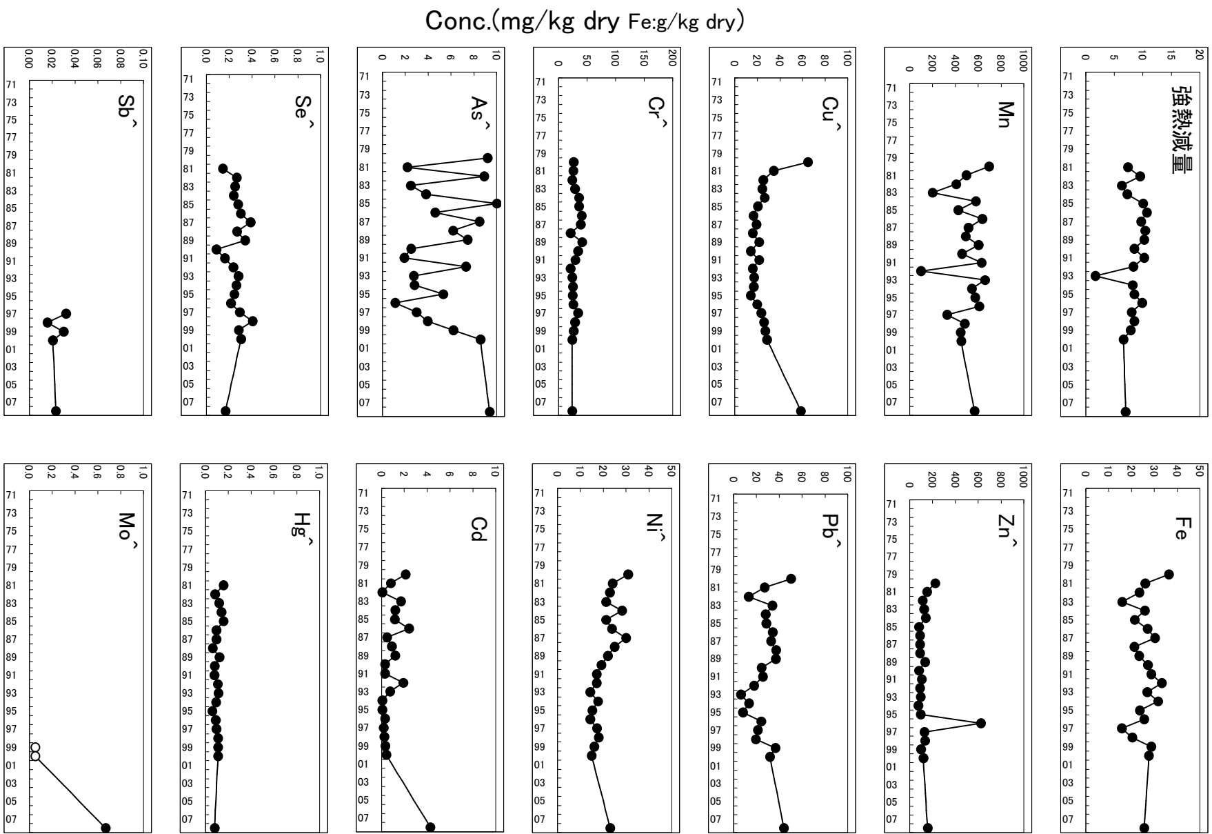
Fig.31 防潮堤外側の重金属経年変化
