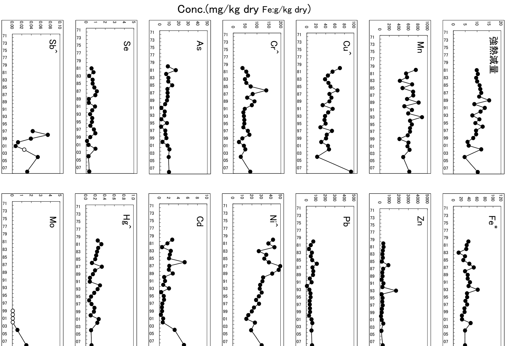
Fig.27 新日鉄沖の重金属経年変化
