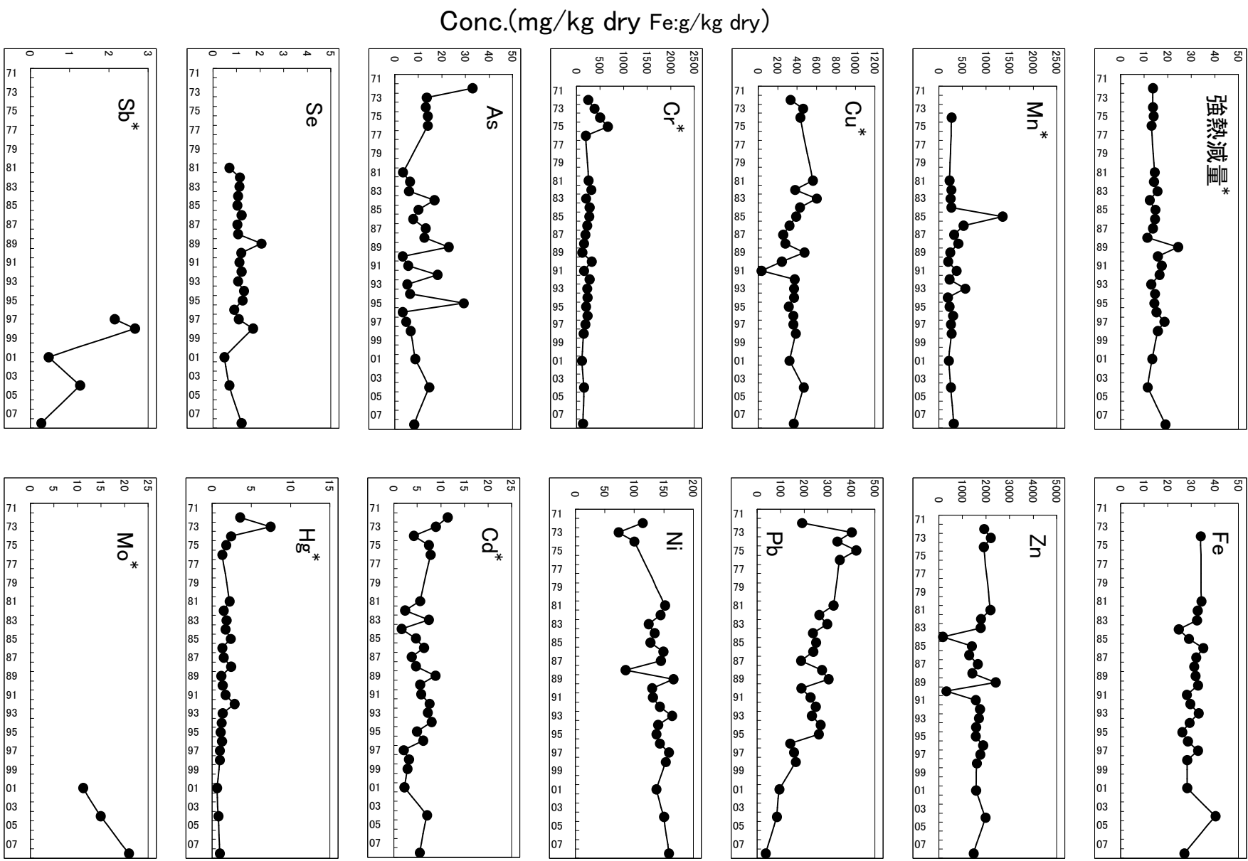
Fig.1.7 南北橋の重金属経年変化
