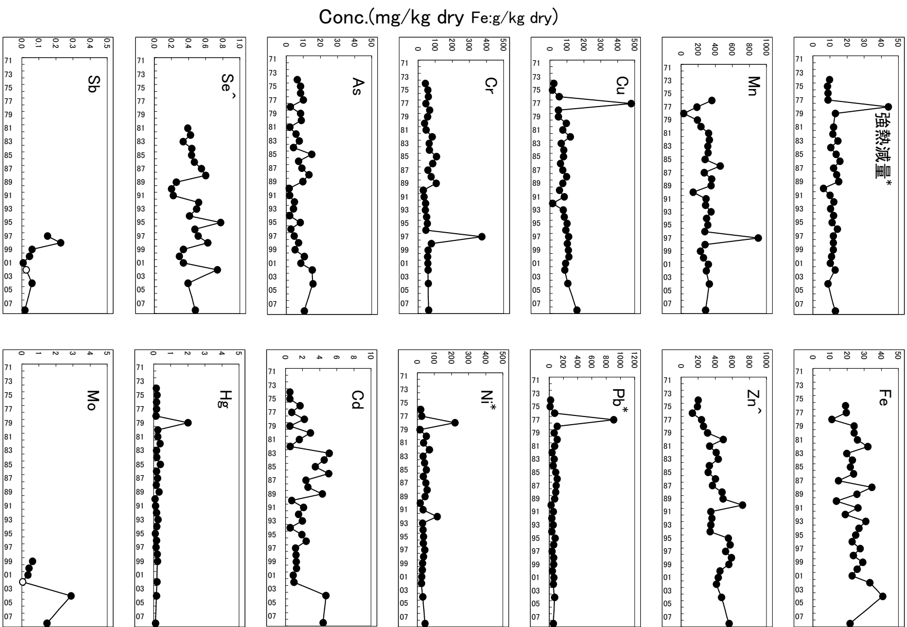
Fig.1.1 金城埠頭の重金属経年変化
