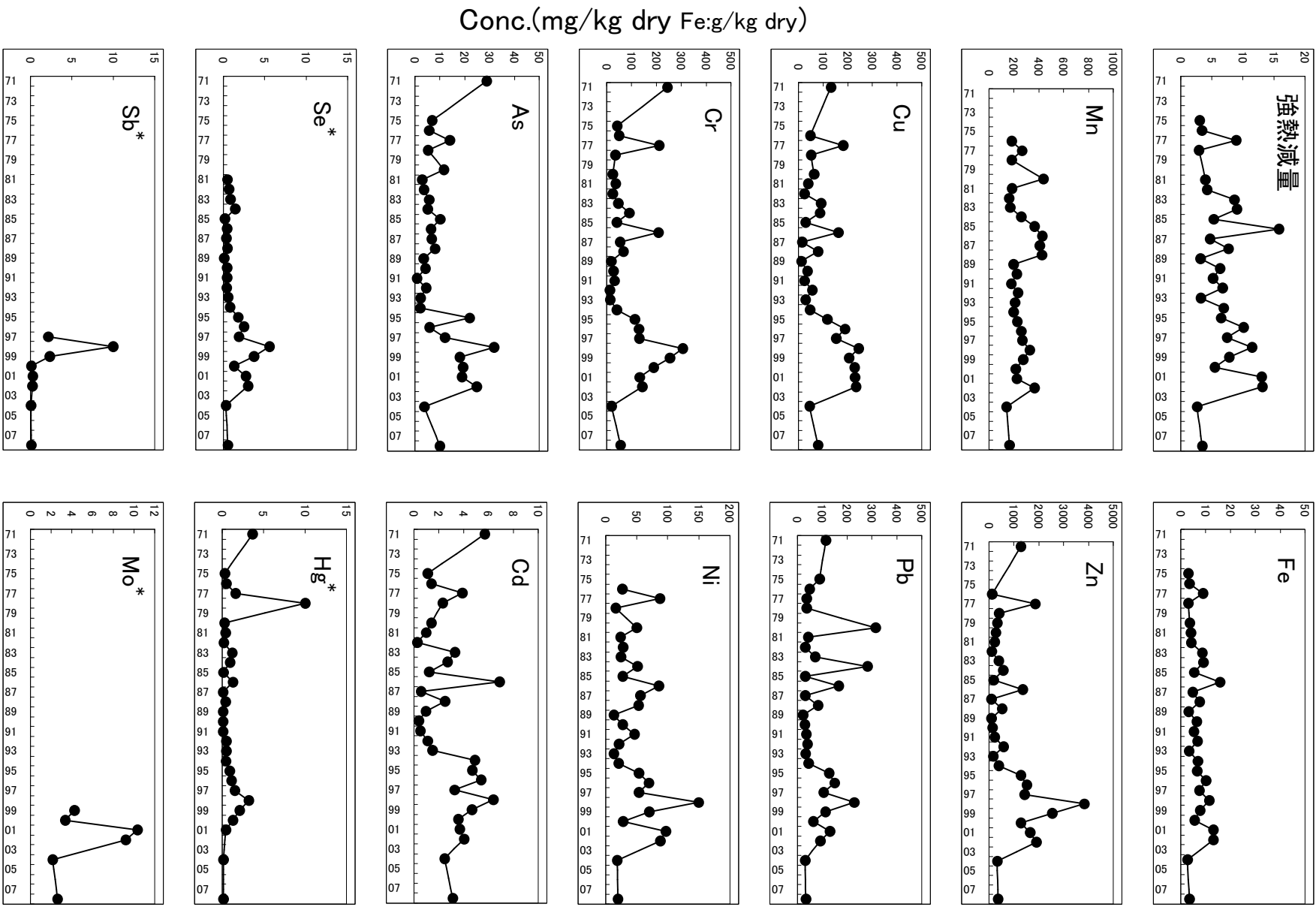
Fig. 3 東海橋の重金属経年変化
