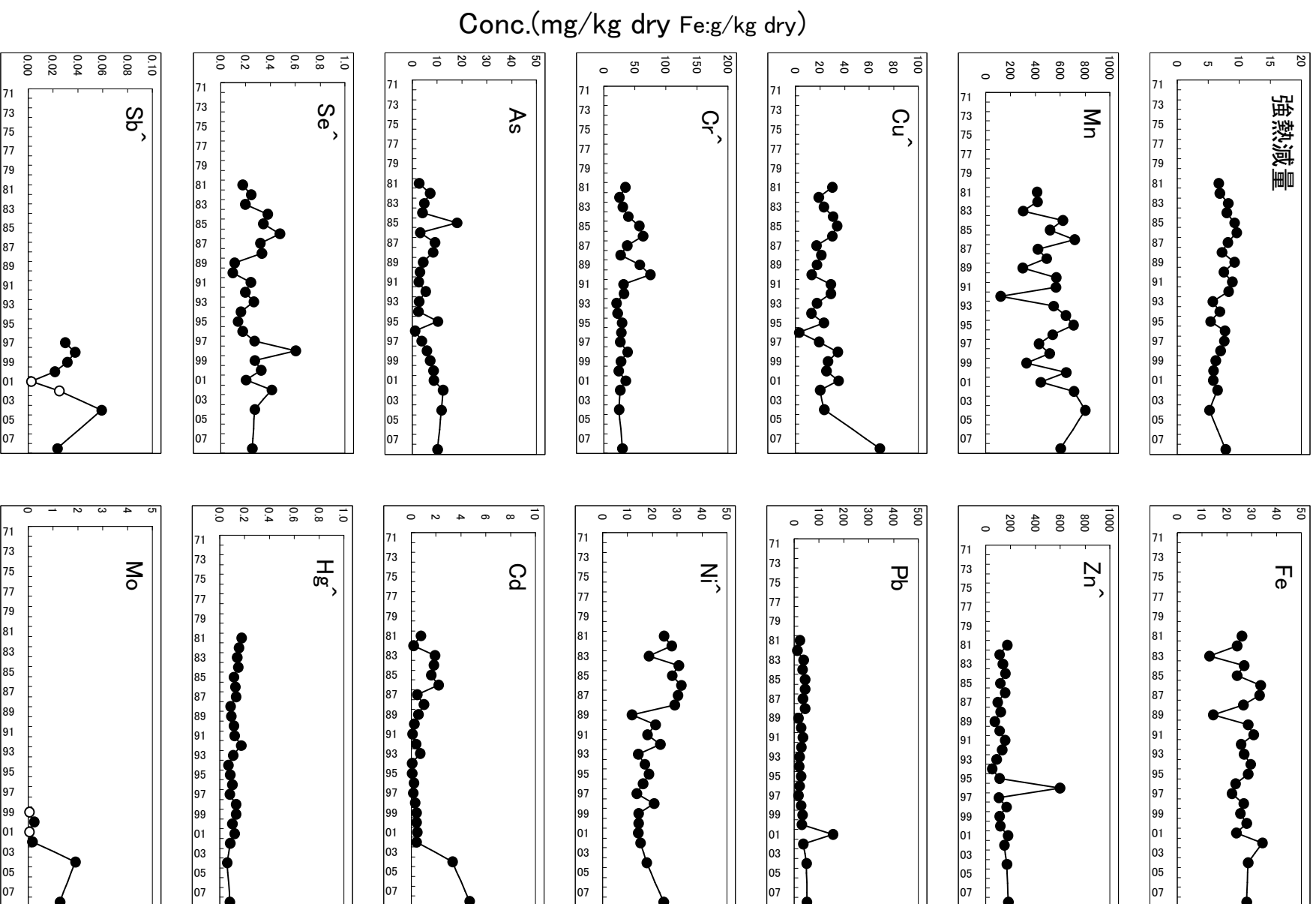
Fig. 29 防潮堤内側の重金属経年変化
