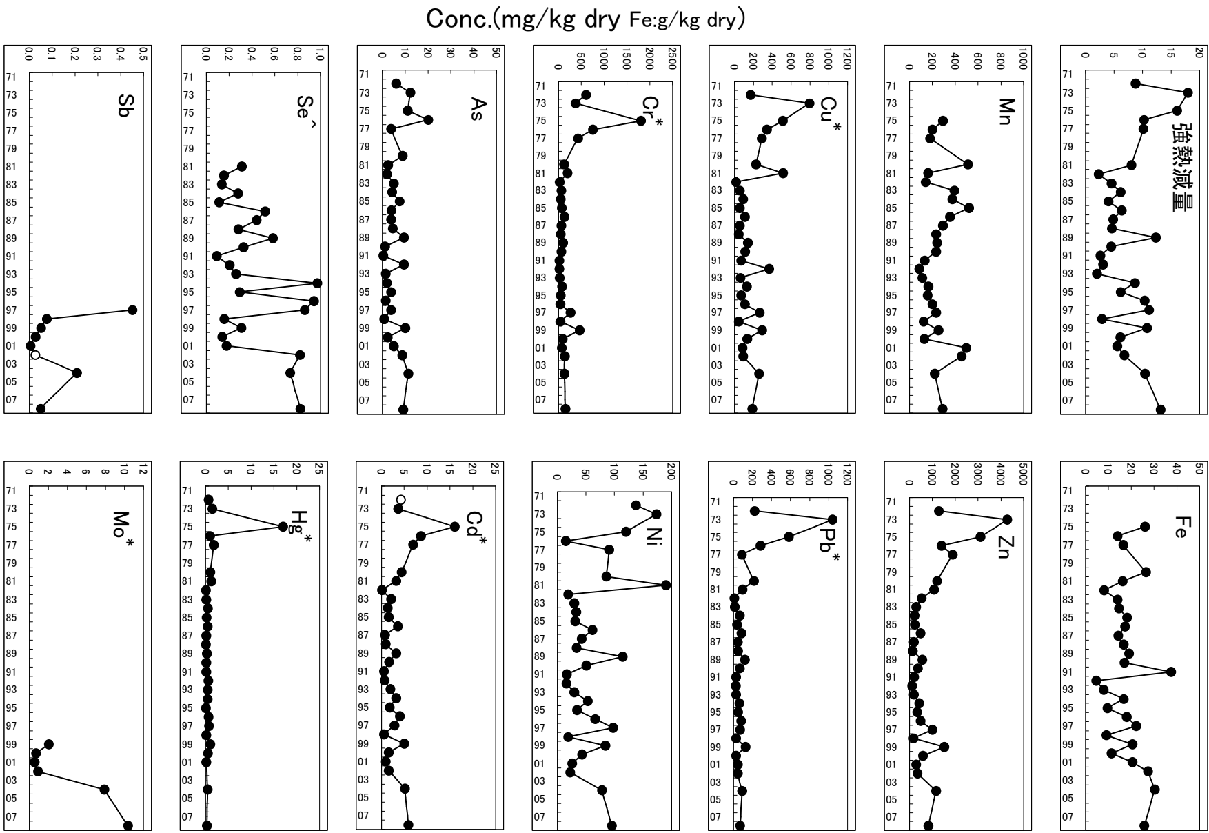
Fig. 7 道徳橋の重金属経年変化
