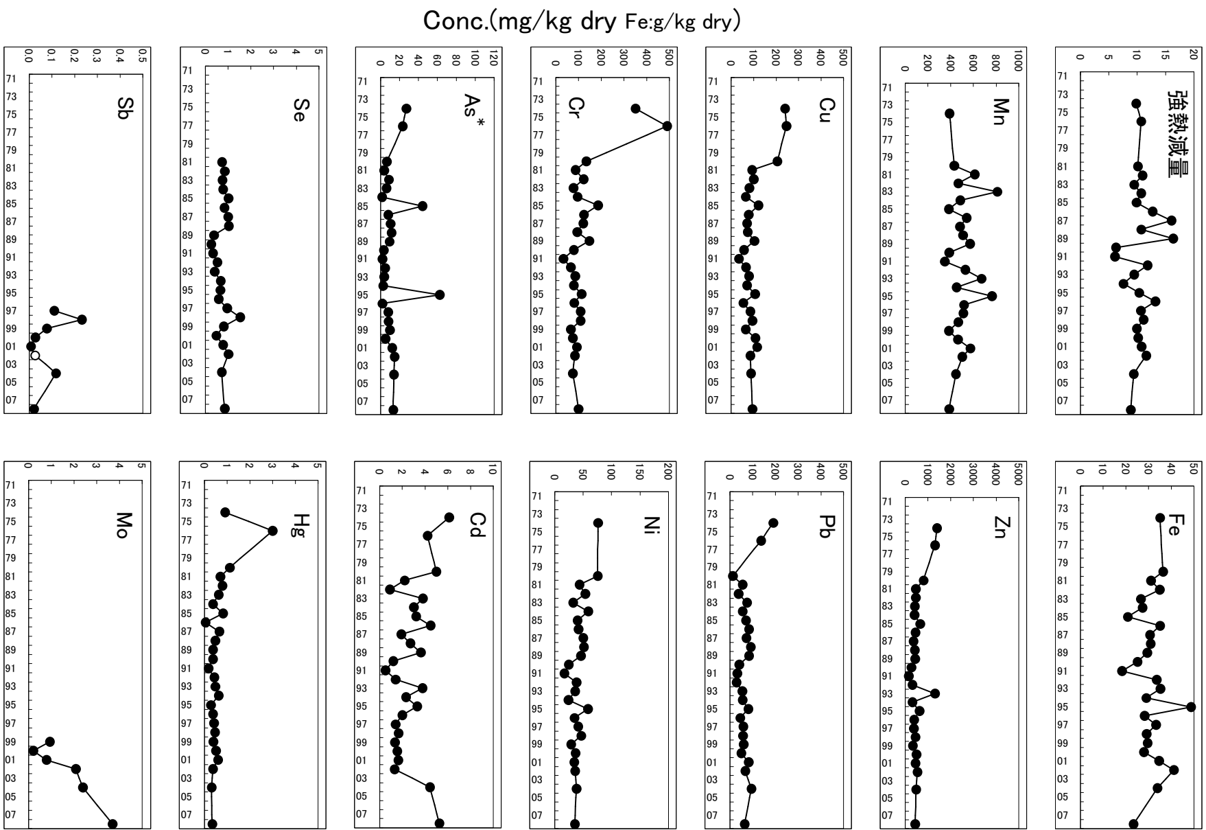
Fig.25 潮見埠頭西の重金属経年変化
