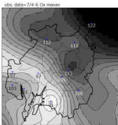
Fig. 7 2008 年 7 月 4 日-6 日における Ox の日最高濃度平均値
