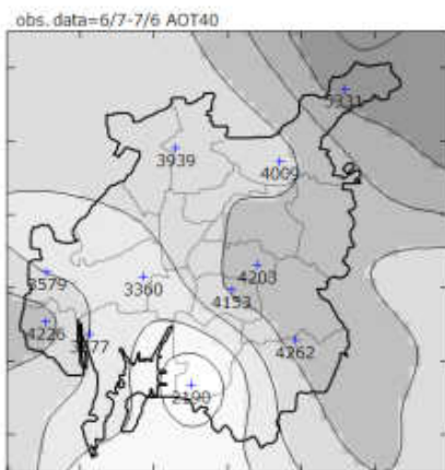
Fig. 8 2008 年 6 月 7 日-7 月 6 日にお ける AOT40
