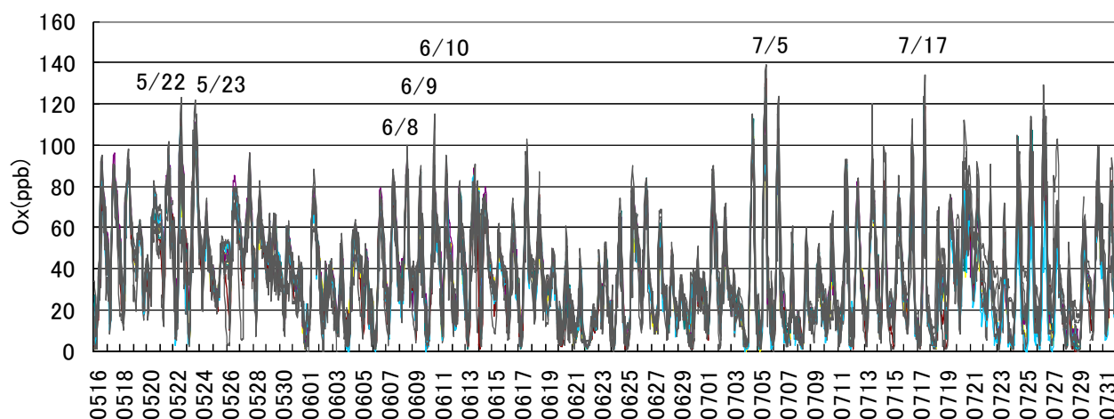
Fig.2 名古屋市内 11 地点における光化学オキシダント濃度一時間値の推移
