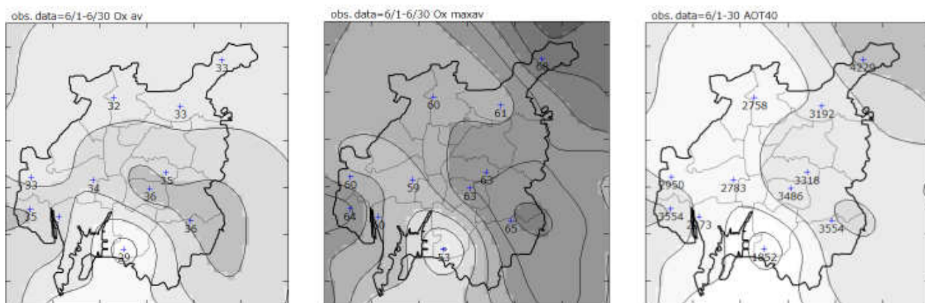
Fig. 5 2008 年 6 月 1 日-30 日における Ox の平均濃度（左）、日最高濃度平均値（中）AOT40（右）
