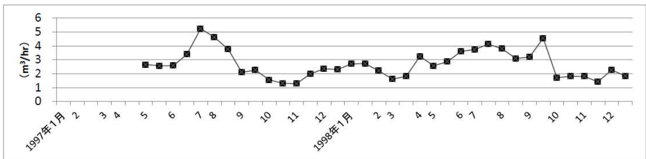
Fig.2 湧水 E における湧水量の変動
