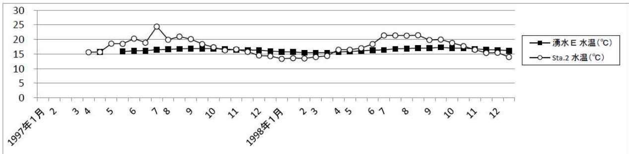
Fig.3 Sta.2 と湧水 E における水温の変動
