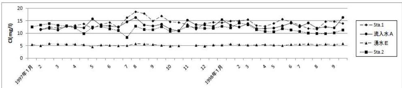
Fig.9 塩素イオン(Cl⁻)の変動
