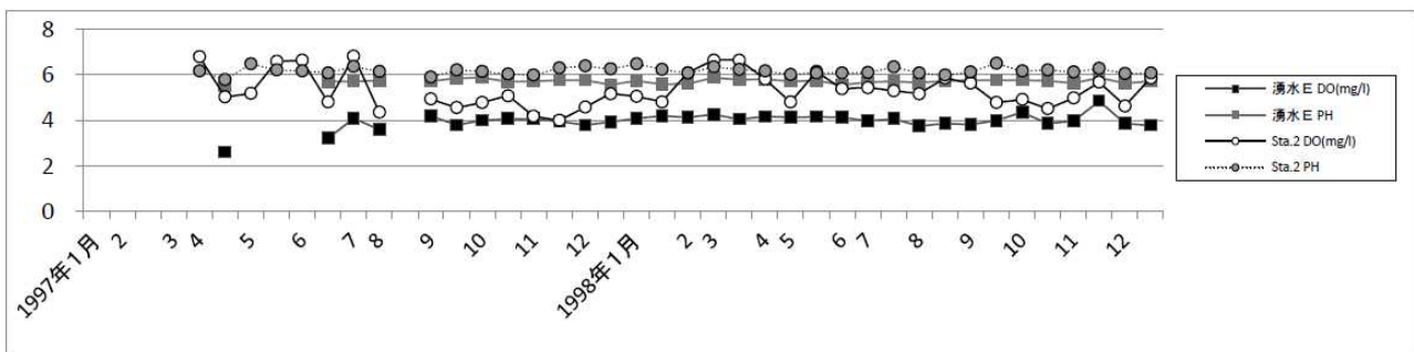
Fig.4 Sta.2 と湧水 E における pH と溶存酸素(DO)の変動
