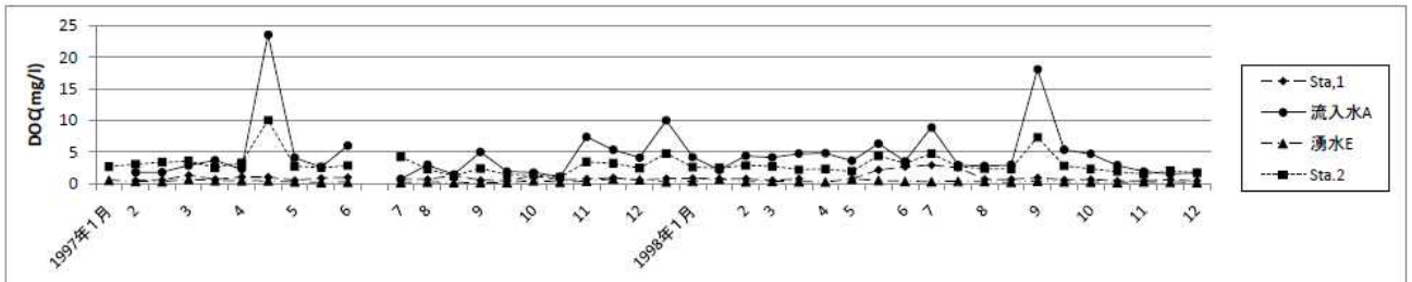
Fig.6 溶存有機炭素(DOC)の変動
