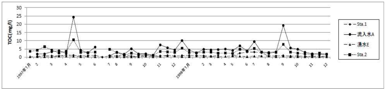
Fig.5 全有機炭素(TOC)の変動
