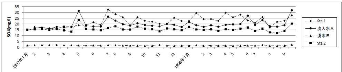
Fig.10 硫酸イオン( \text{SO}_4^{2-} )の変動
