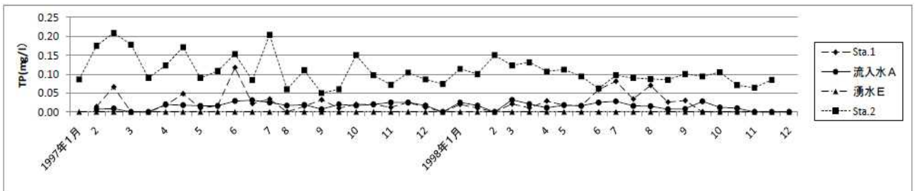
Fig.8 全リン(TP)の変動
