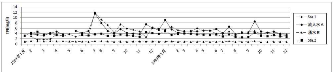
Fig.7 全窒素(TN)の変動
