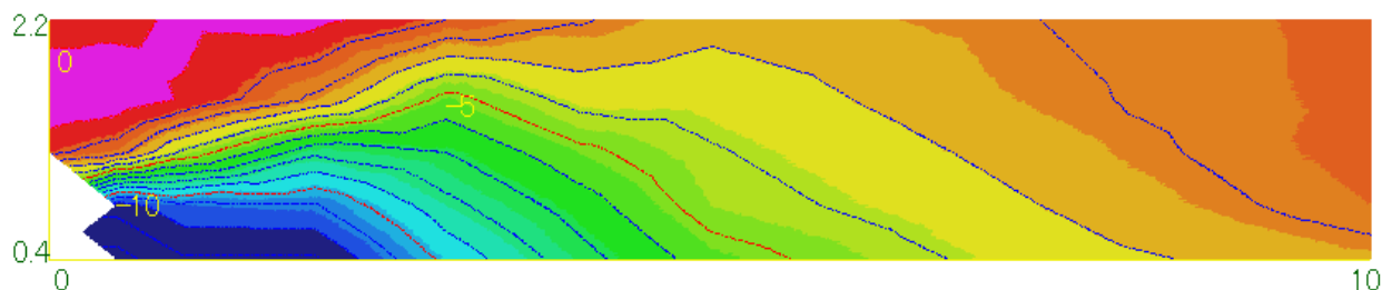
Fig.4 中心断面のコンター図（花壇型5m長）
