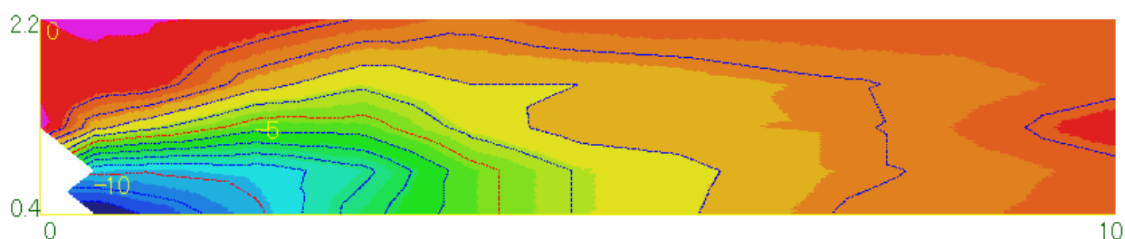
Fig.3 中心断面のコンター図（標準型両面吸音5m長）
