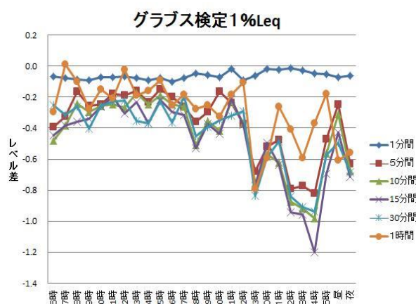
図 2.3 環境騒音全地点差の平均値
