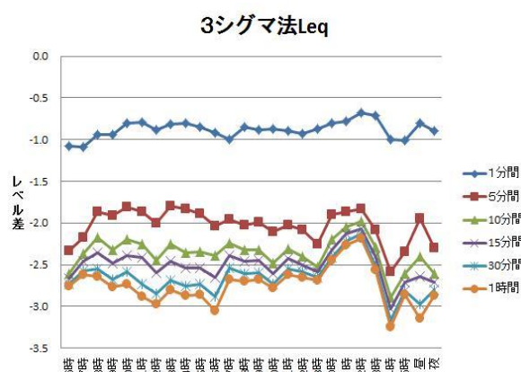
図 2.4 環境騒音全地点差の平均値
