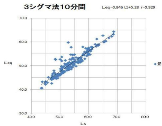
図 3.4 Leq と L5 との散布図
