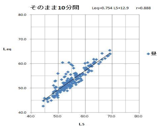
図 3.5 Leq と L5 との散布図
