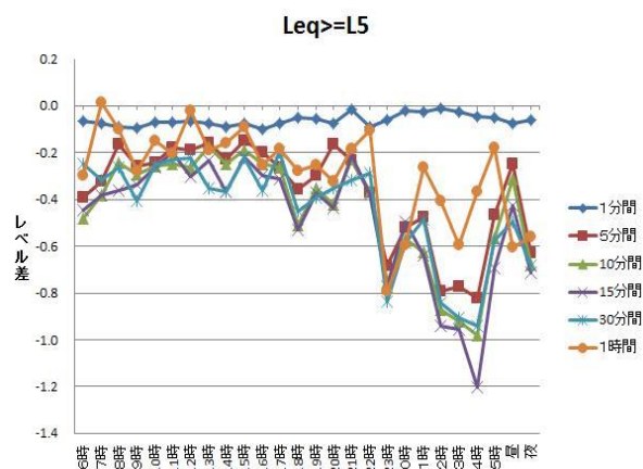
図 2.1 環境騒音全地点差の平均値
