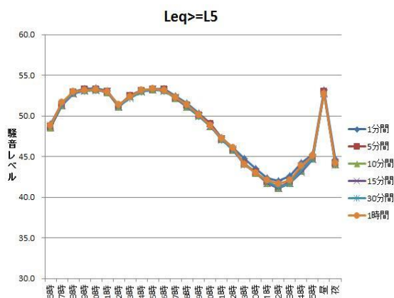
図 1.1 環境騒音全地点平均値
