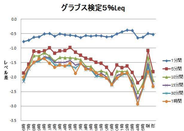
図 2.2 環境騒音全地点差の平均値
