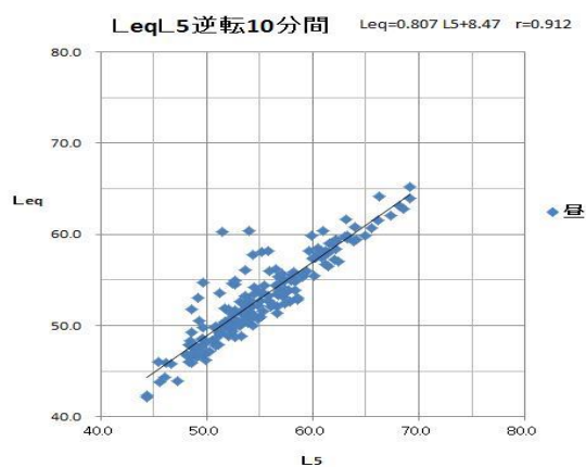
図 3.1 Leq と L5 との散布図
