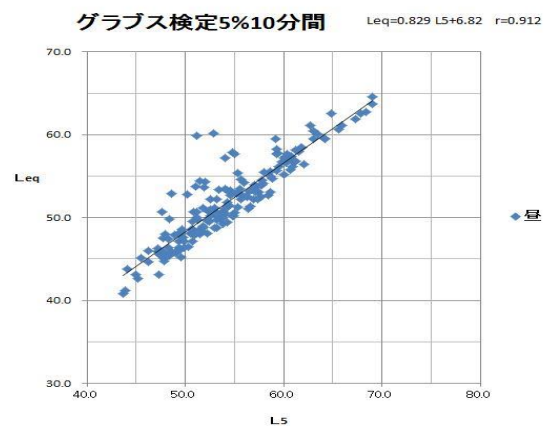
図 3.2 Leq と L5 との散布図
