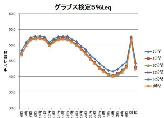
図 1.2 環境騒音全地点平均値
