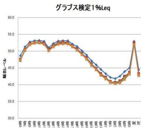
図 1.3 環境騒音全地点平均値
