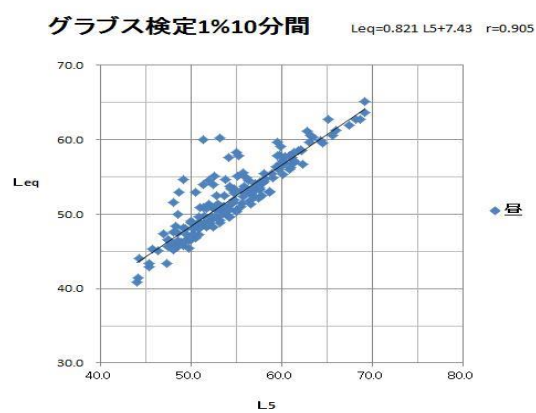
図 3.3 Leq と L5 との散布図
