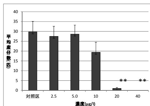
図 1 銅を用いたミジンコ繁殖阻害試験結果
